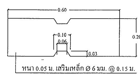
รูปขยาย ①
