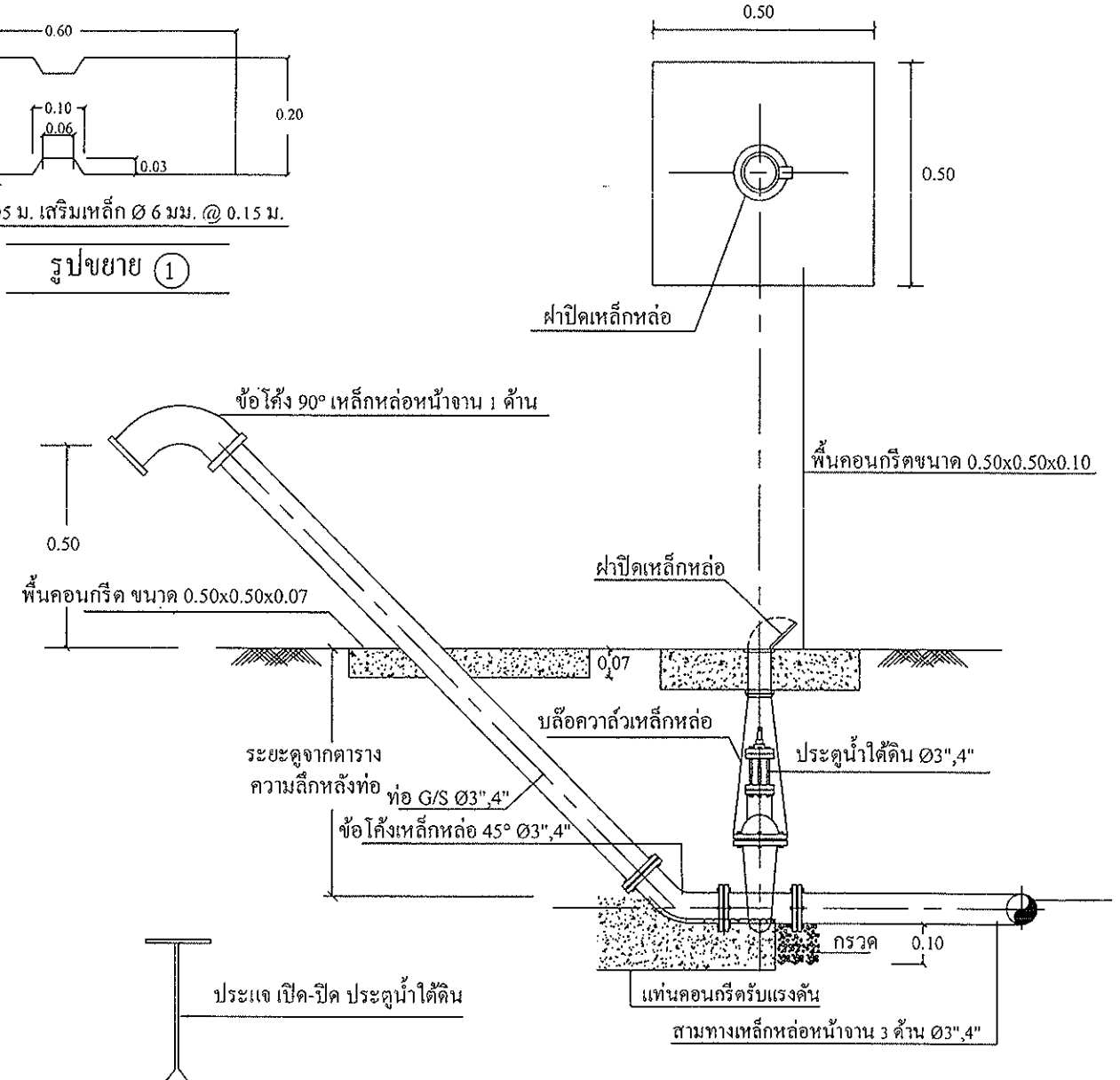
13. แบบการติดตั้งประตูปะทะระบายตะกอน
