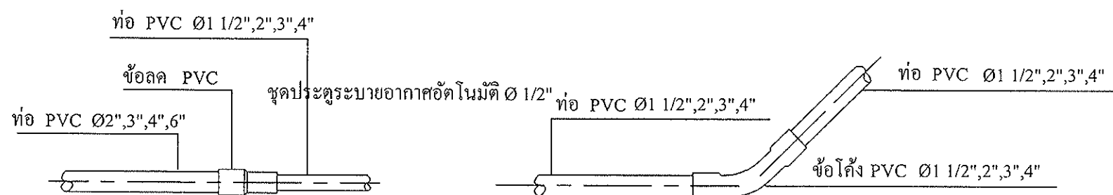
1. แบบการวางท่อทั่วไป
