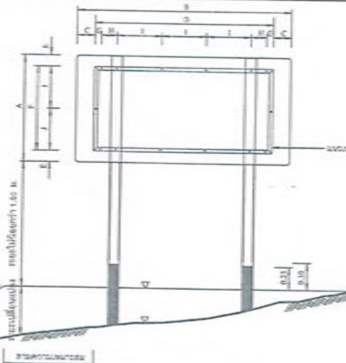
รูปแสดงการประกอบแผ่นป้าย ขนาดตัว 1:20
