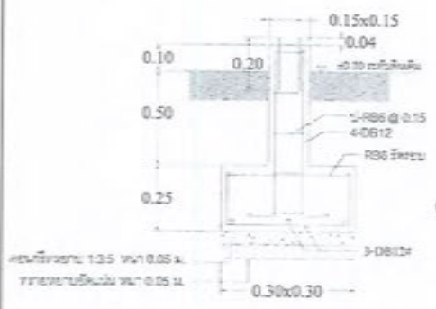
แบบขยายฐานราก F
