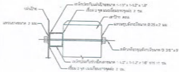
รูปตัดขยายการยึดแผ่นป้ายและเสา ขนาดตัว 1:20
