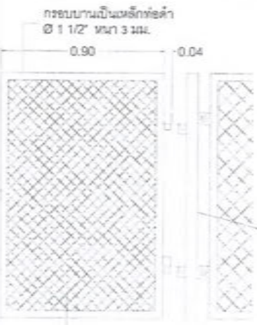
แบบขยายรายละเอียดแสดงการยึดระหว่างรั้วกับเสา
