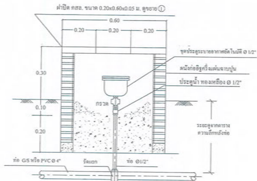
11. การติดตั้งประตูละบายอากาศอัดโนมิตี
