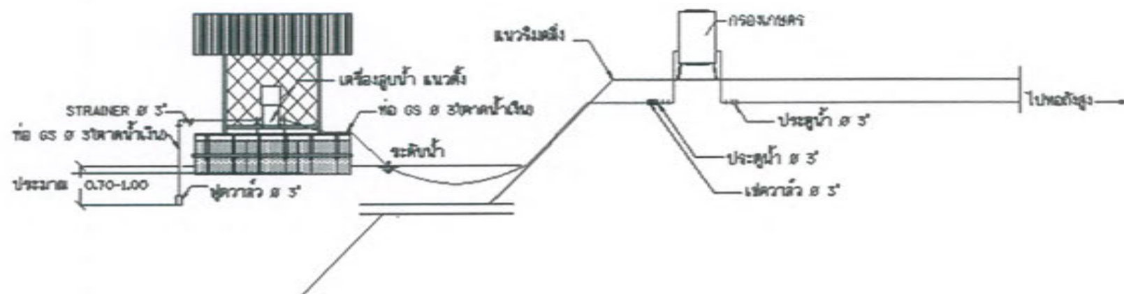
รูปด้านข้าง 1:25
