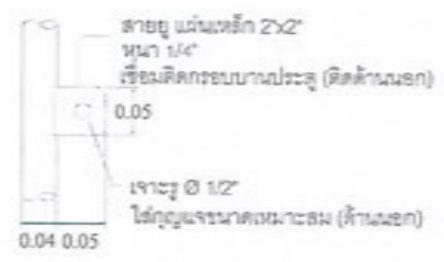
แบบขยายสายยู
