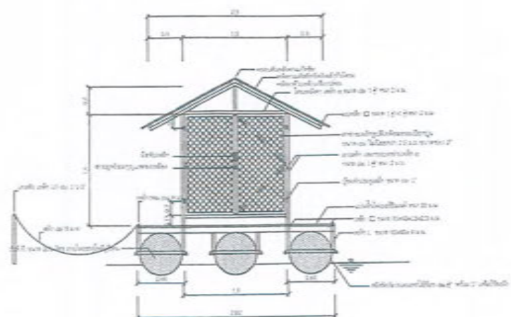
รูปด้านหน้า 1:25
