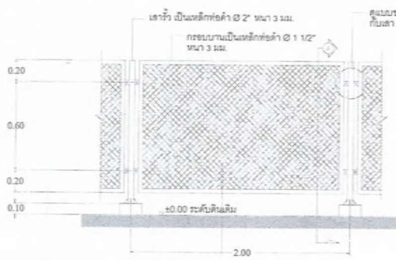
ลดค่าข้อยื่นรูปด้วยการหัก แบบค่าข้อยื่นเหลี่ยมจตุรัส ขนาดช่องคาน้ำ 1 1/4" ขนาดเส้นลวด 3 มม. (เบอร์ 11)
