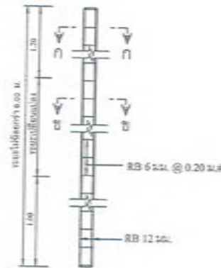
รายละเอียดเสาป้าย คสล. ขนาดตัว 1:20
