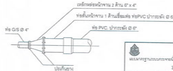
8. การบรรจุท่อเหล็กอบสังกะสี (G/S) กับท่อ PVC.
