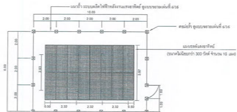
แปลนการติดตั้งแผงเซลล์แสงอาทิตย์ พร้อมรั้ว
