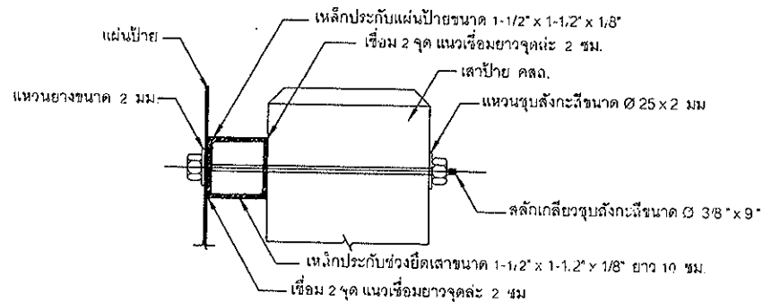
รูปตัดขยายการยึดแผ่นป้ายและเสา มาตรฐาน 1:20
