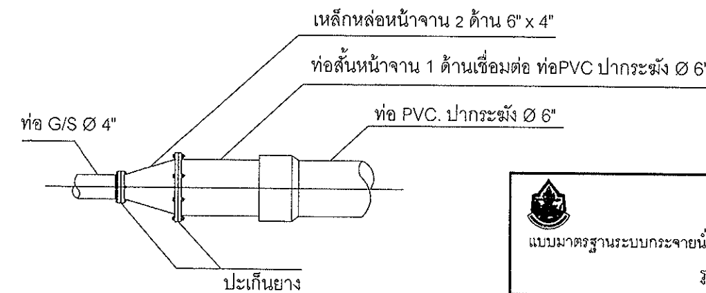
8. การบรรจบท่อเหล็กอาบสังกะสี (G/S) กับท่อ PVC.
