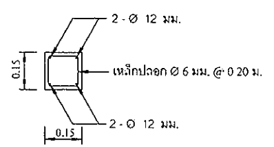
รูปตัด ก - ก มาตรฐาน 1:10
