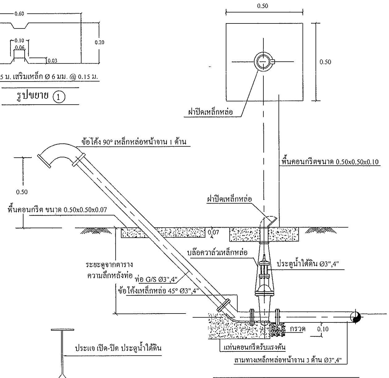
13. แบบการติดตั้งประตูปะบายตะกอน
