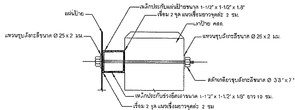
รูปตัดขยายการยึดแผ่นป้ายและเสา มาตรฐาน 1:20
