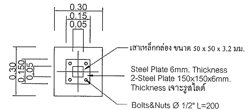
รูปขยายเสาหลัก C1
