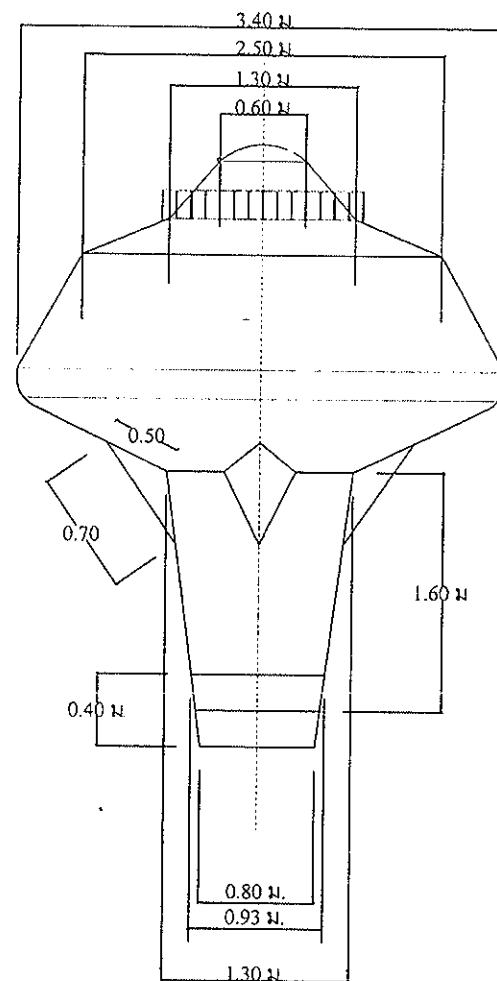
แบบขยายแมนโซลบนห้องสูง มาตราส่วน 1 : 50
