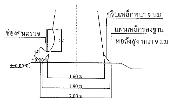
แบบขยายแมนโซลล่างห้องสูง มาตราส่วน 1 : 50
