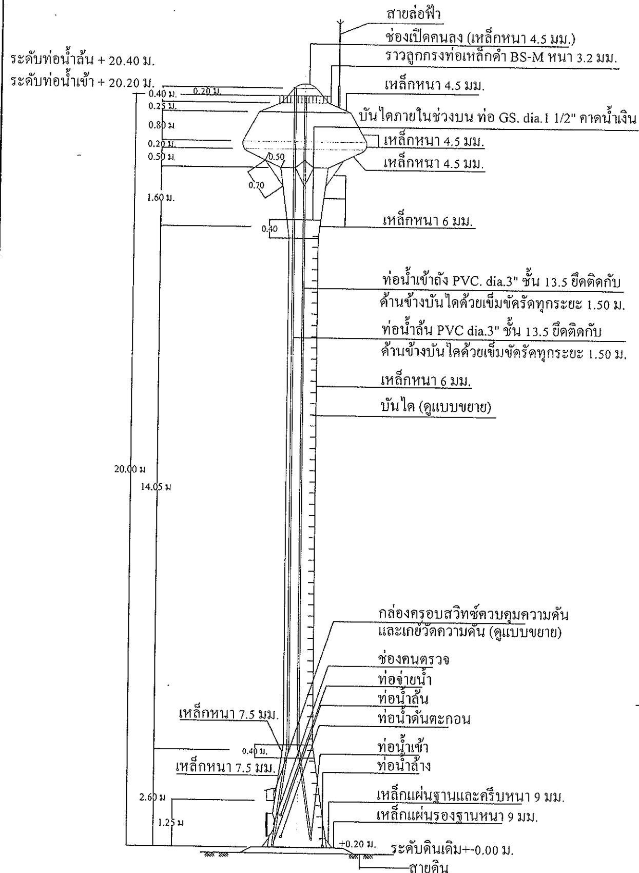
รูปด้านข้างห้องสูง แบบถังเหล็กรูปทรงแชมเปญ มาตราส่วน 1 : 100
