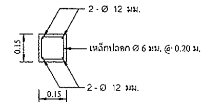
รูปตัด ก - ก มาตรฐาน 1:10
