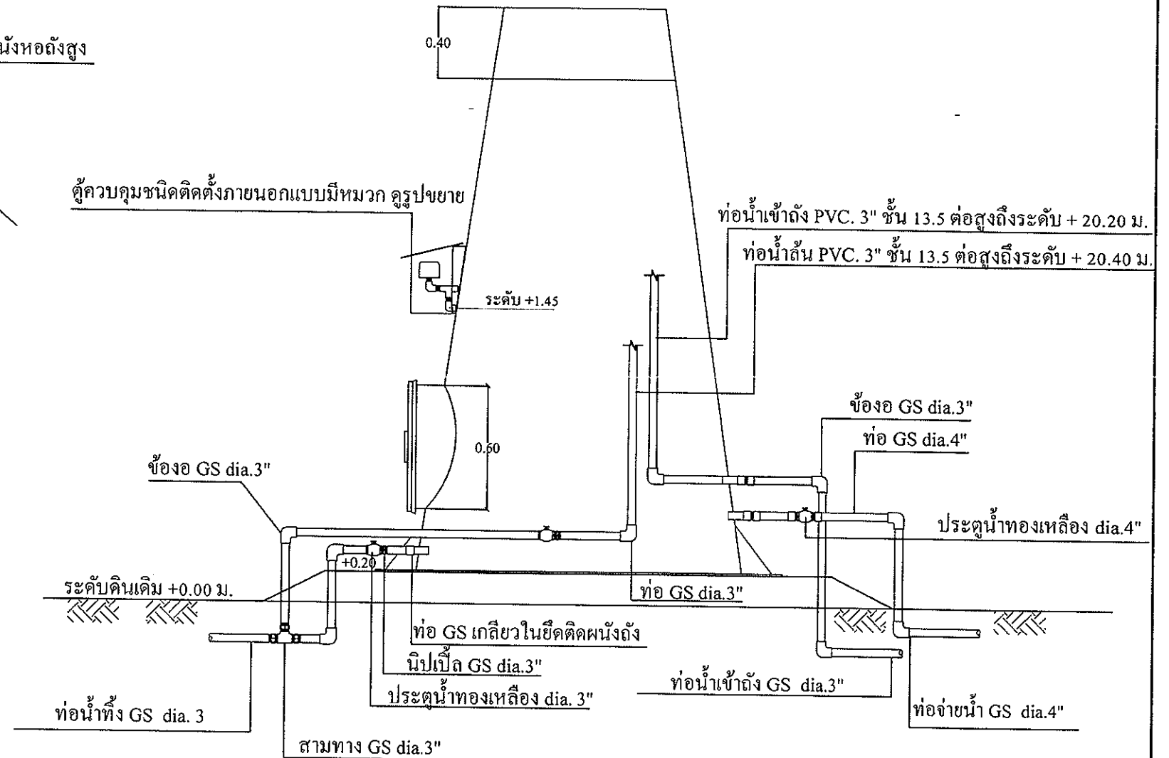
แบบแสดงการเดินท่อในห้องสูง มาตราส่วน 1 : 25
