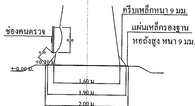
แบบขยายแมนโซลล่างหอดังสูง มาตราส่วน 1 : 50
