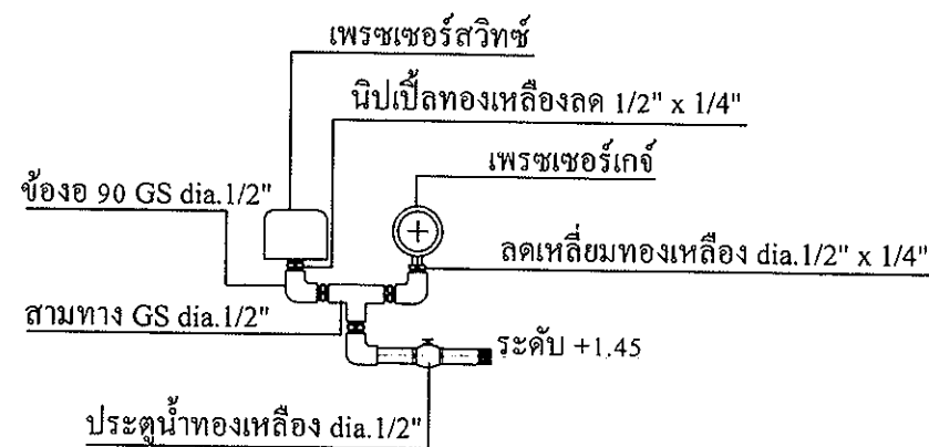
แบบขยายสวิทช์ควบคุมและแก้วัดความดัน
