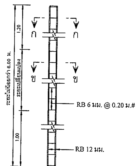
รายละเอียดภายใน คสท. มาตราส่วน 1:20
