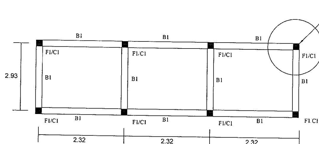
แปลนฐานรากและคานหลัก
