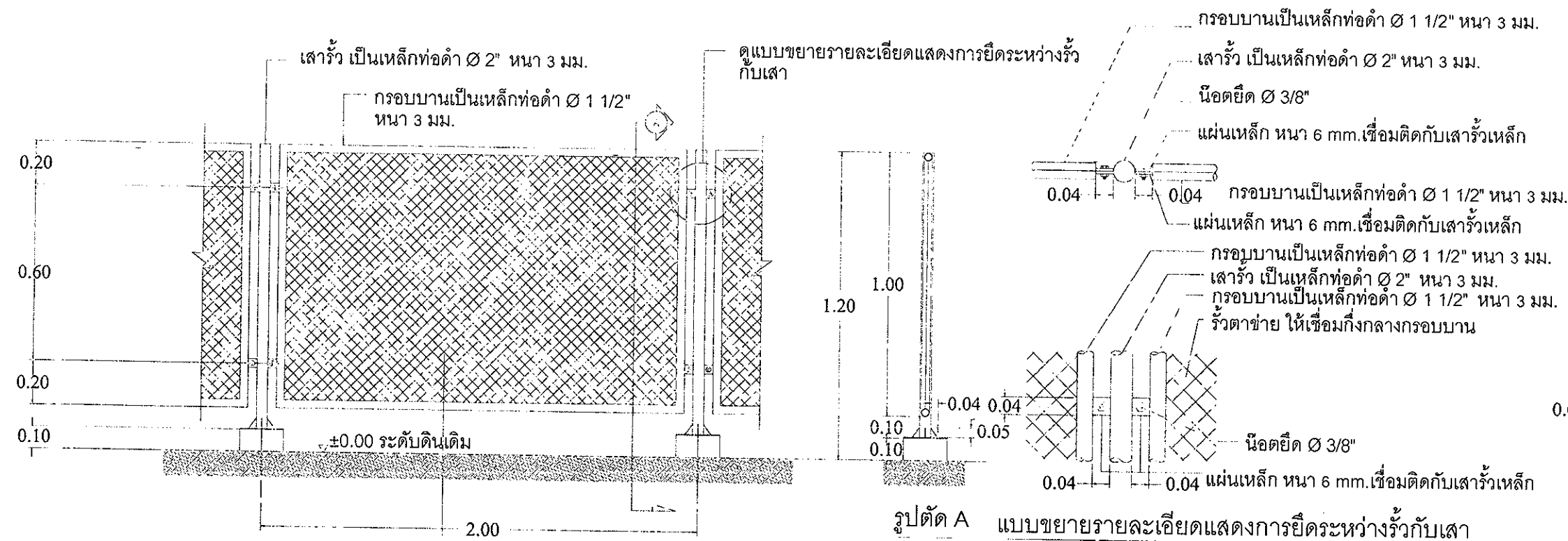
แบบขยายรั้วลวดตาข่าย
