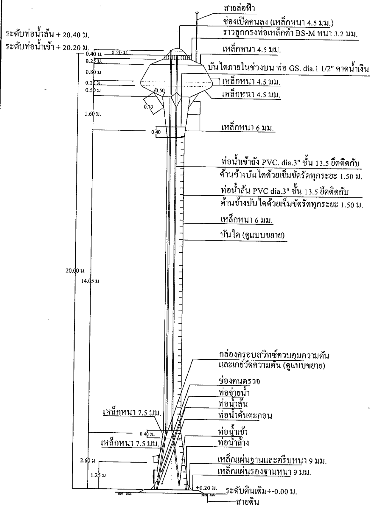
รูปด้านข้างหอดังสูง แบบถังเหล็กรูปทรงแชมเปญ มาตราส่วน 1 : 100
