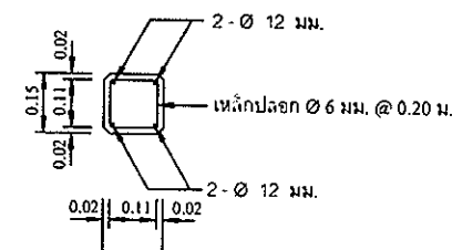
รูปตัด ข - ข
