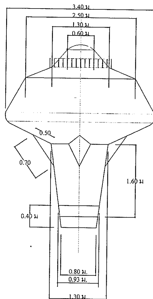
แบบขยายแมนโซลบนหอดังสูง มาตราส่วน 1 : 50
