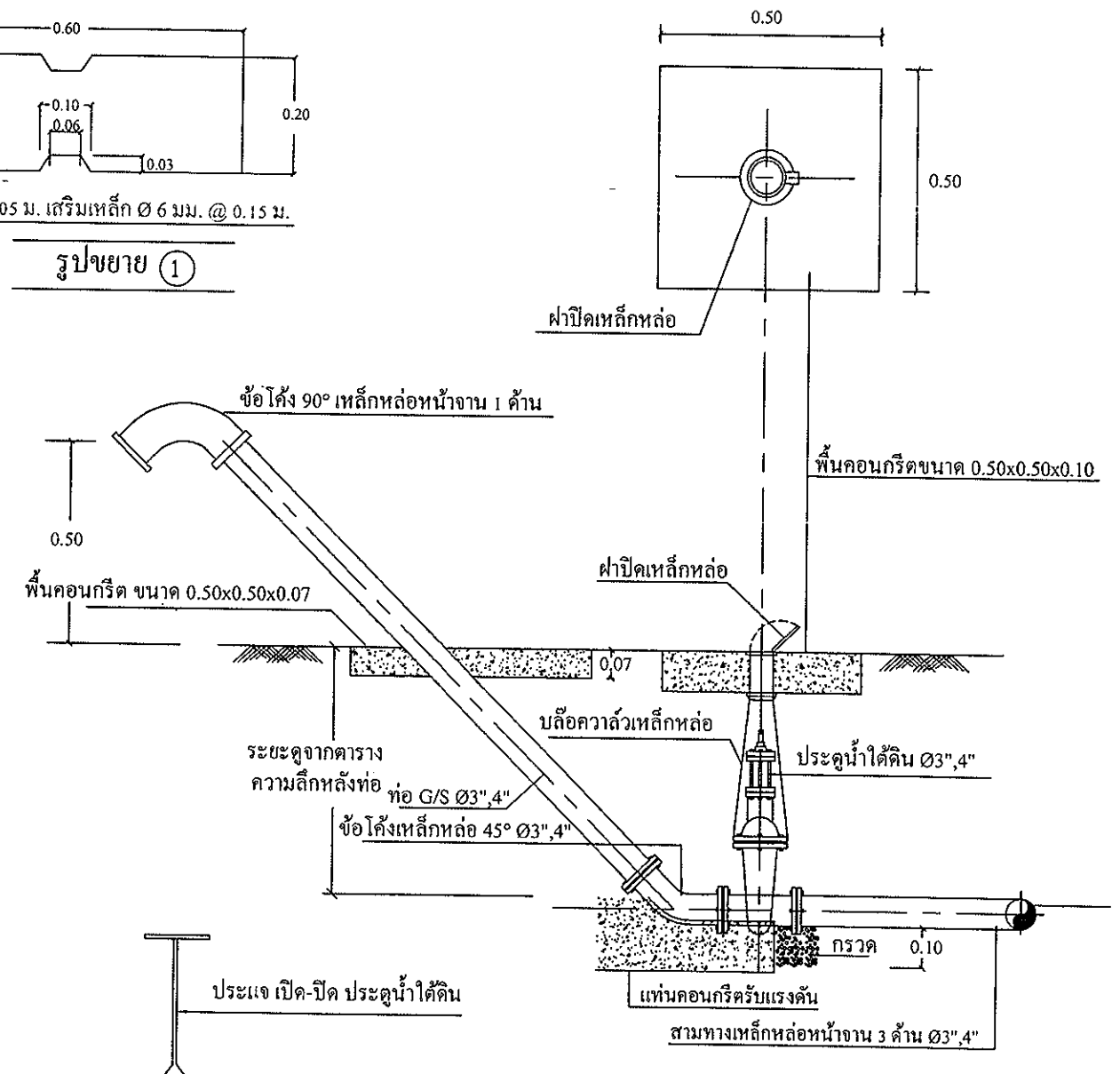
13. แบบการติดตั้งประตูละบายตะกอน
