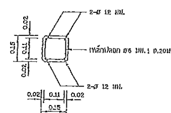
รูปตัด ข - ข
