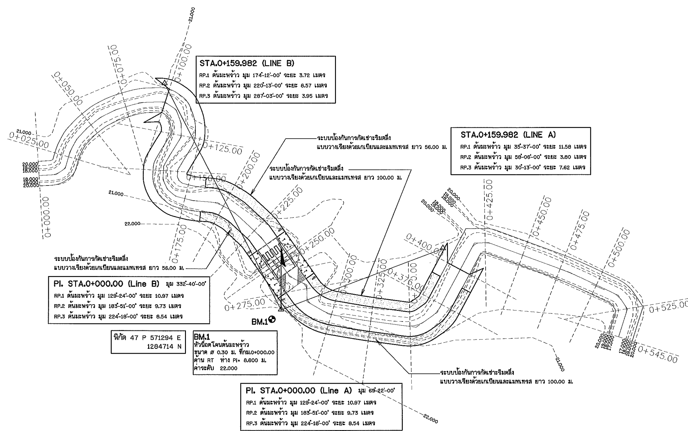
แปลนแสดงการขุดลอกทั่วไป มาตราส่วน 1:1000
