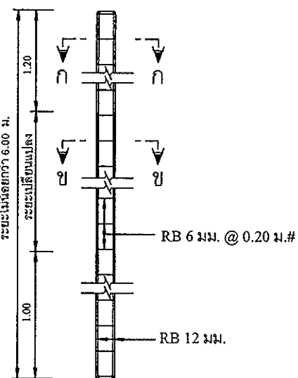
รายละเอียดเสาป้าย คสล. มาตรฐาน 1:20
