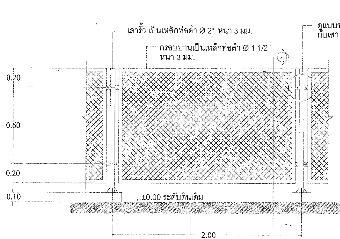
แบบขยายหัวลดตาข่าย
