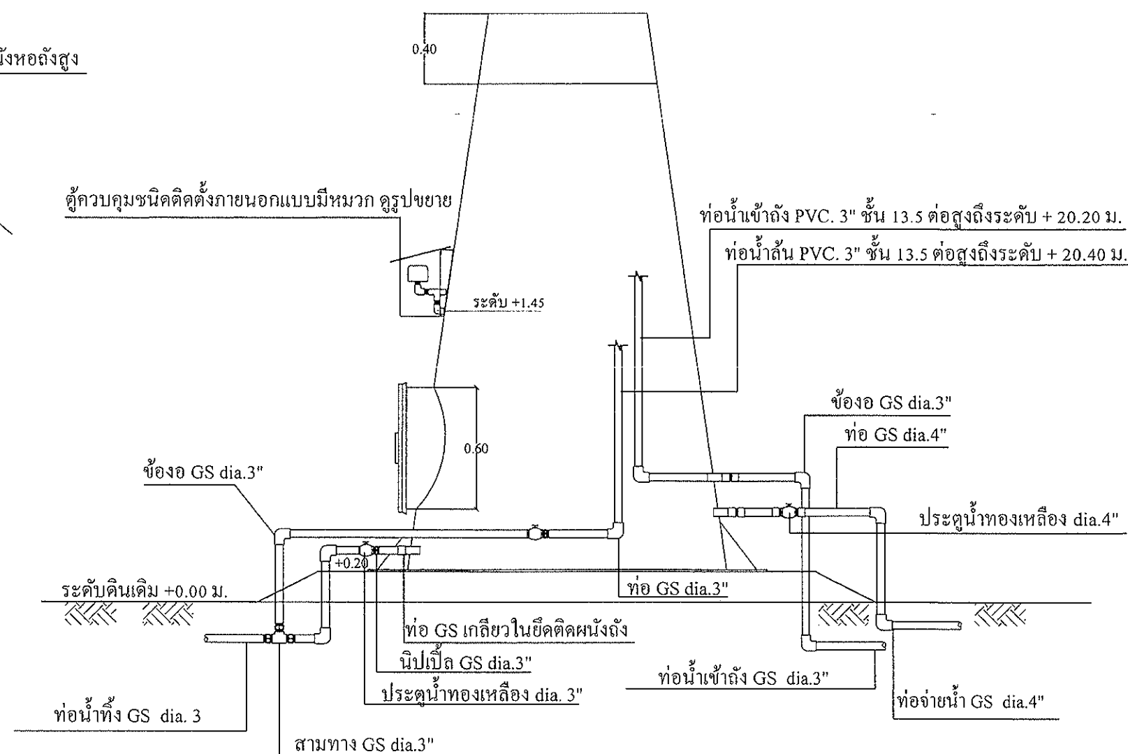
แบบแสดงการเดินท่อในหอถังสูง มาตราส่วน 1 : 25
