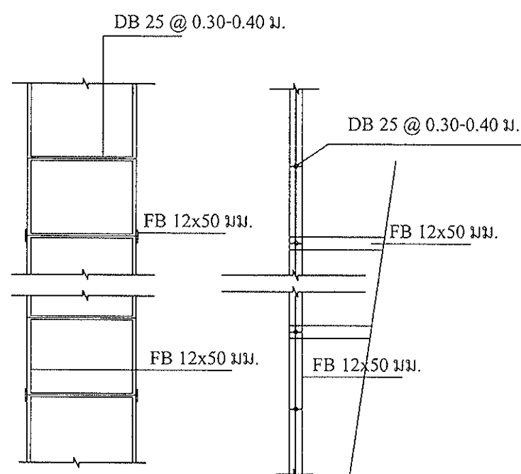
แบบขยายบันได ภายในหอถังสูง มาตราส่วน 1 : 20
