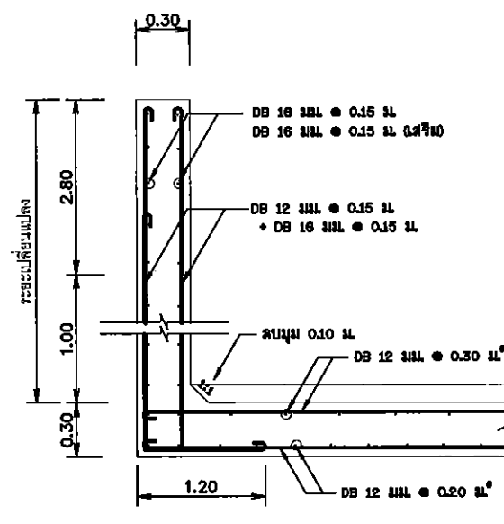
รูปตัด "ค" มาตราส่วน 1:25
