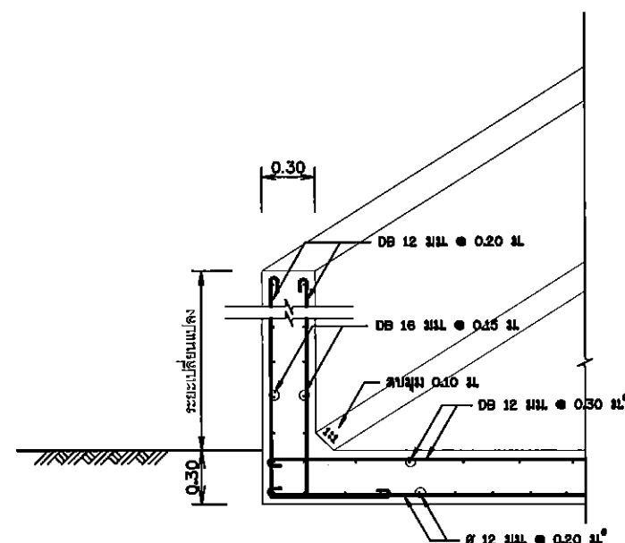
รูปตัด "ง" มาตราส่วน 1:25
