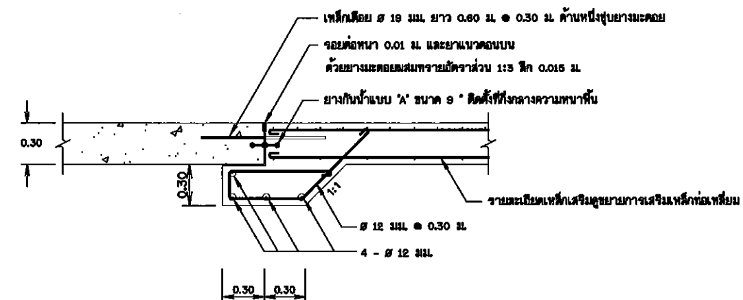
รูปขยายรอยต่อคอนกรีต มาตราส่วน 1:25
