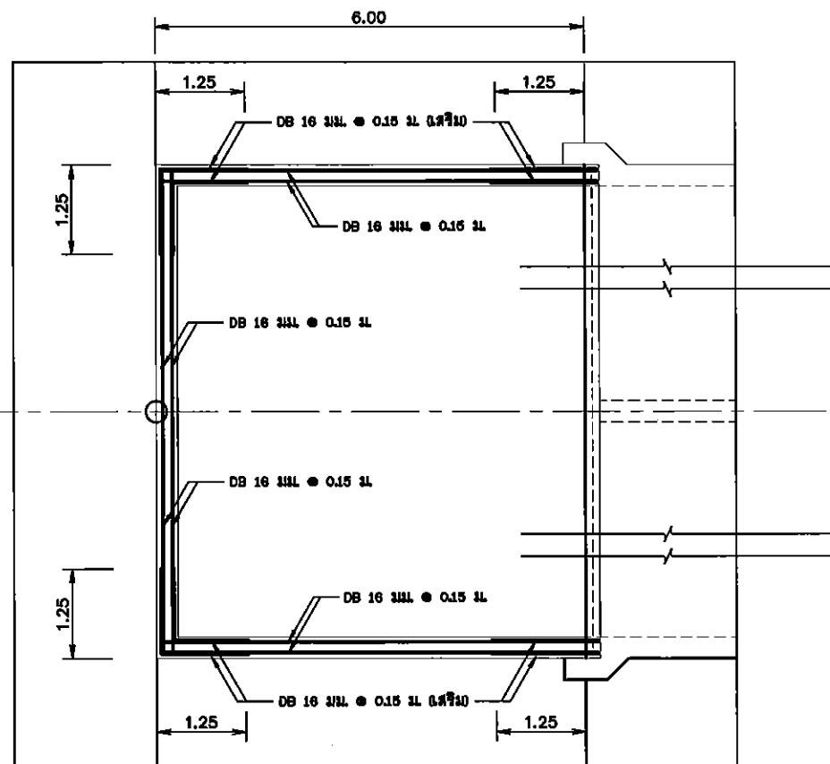
แบบขยายเหล็กกำแพง มาตราส่วน 1:25
