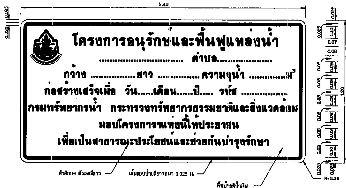
ป้ายโครงการ 1:10
