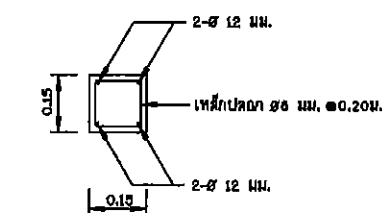
รูปตัด ก - ก 1:10
