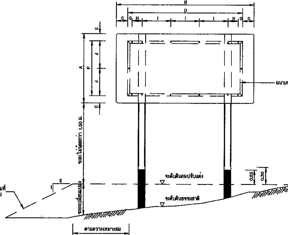
รูปแสดงการประกอบแผ่นป้าย 1:20
