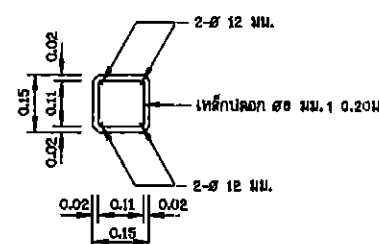
รูปตัด ข - ข 1:10
