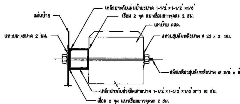
รูปตัดขยายการยึดแผ่นป้ายและเสา 1:20
