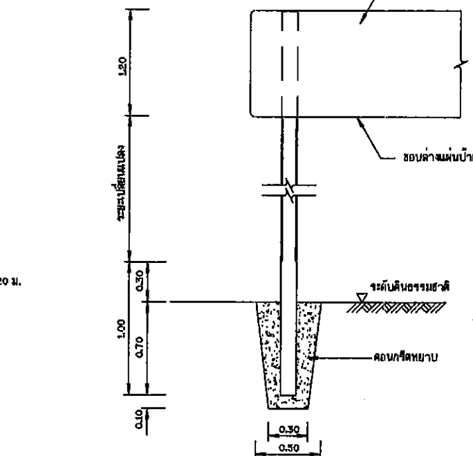
รายละเอียดการติดตั้งเสาป้าย 1:20
