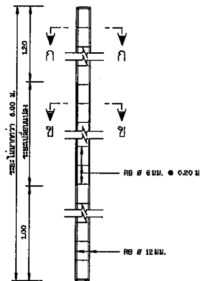
รายละเอียดเสาป้าย คสล. 1:20
