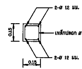
รูปตัด ก - ก 1:10
