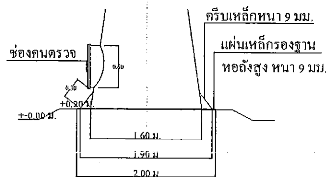
แบบขยายแมนโฮลล่างถังสูง มาตราส่วน 1:50
