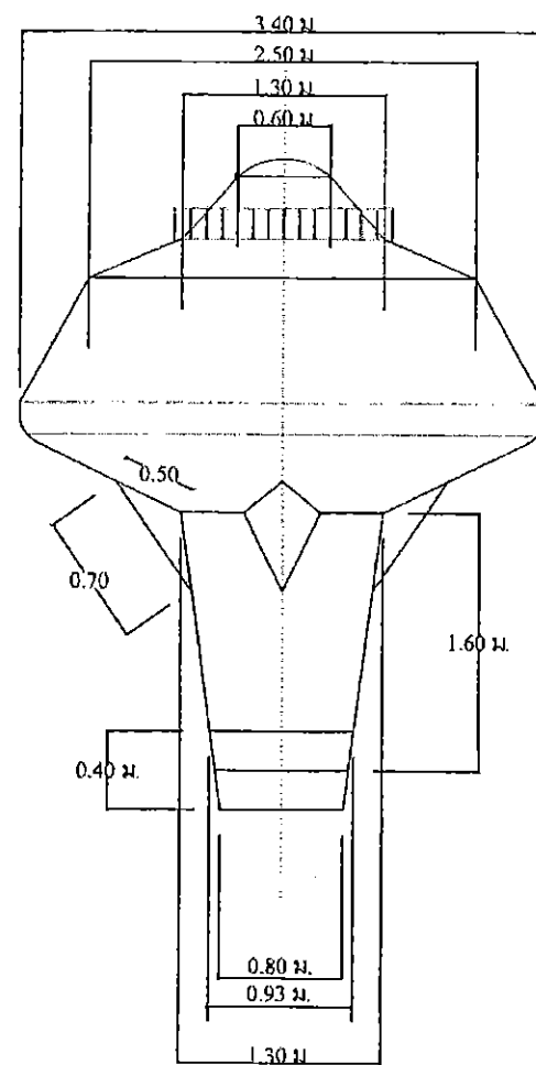
แบบขยายแมนโฮลบนถังสูง มาตราส่วน 1:50
