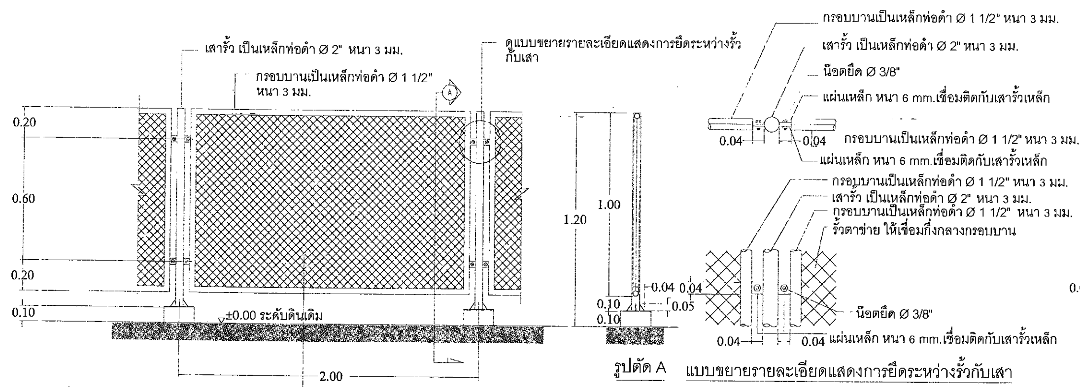
แบบขยายรั้วลดทอน
