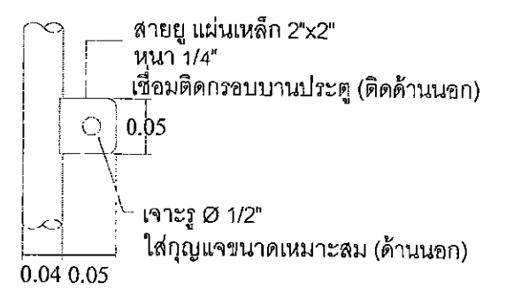
แบบขยายสายยู
