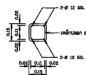
รูปตัด ข - ข 1:10
