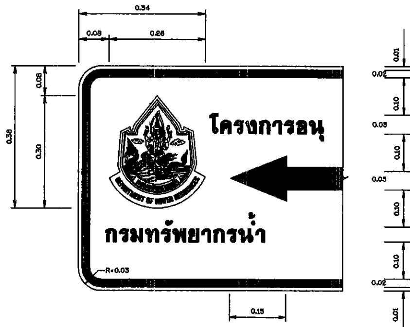
รูปขยายตราสัญลักษณ์ มาตราส่วน 1:15
