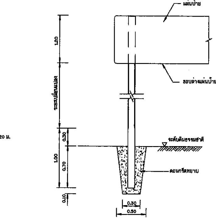
รายละเอียดการติดตั้งเสาป้าย 1:20
