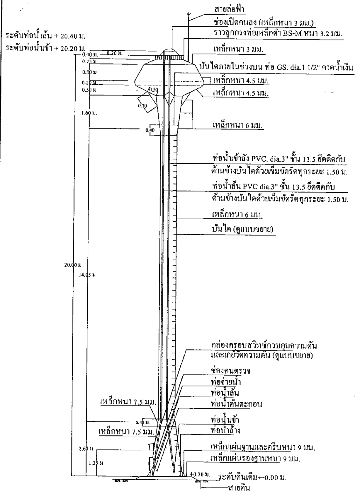
รูปด้านข้างของถังสูง แบบถังเหล็กทรงกลมแป้น มาตราส่วน 1:100
