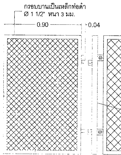
รูปตัด A แบบขยายรายละเอียดแสดงการยึดระหว่างรั้วกับเสา
