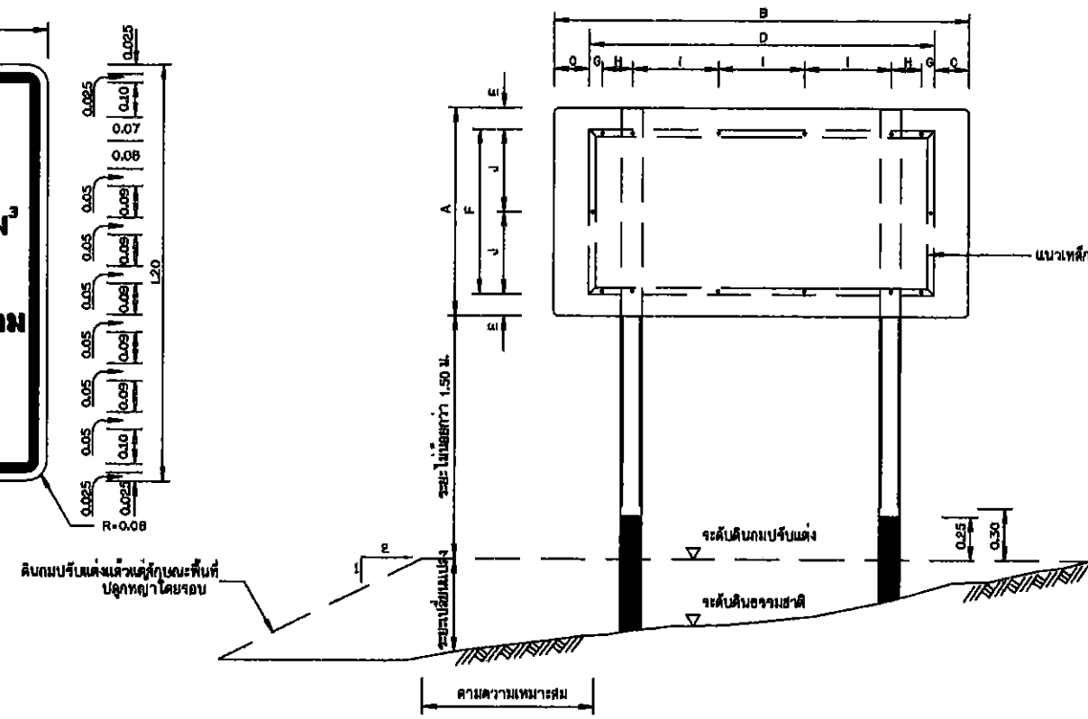
รูปแสดงการประกอบแผ่นป้าย 1:20
