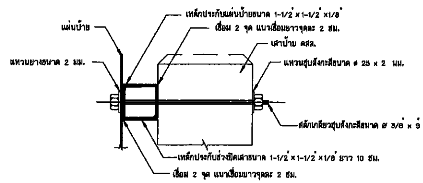
รูปตัดขยายการยึดแผ่นป้ายและเสา 1:10
