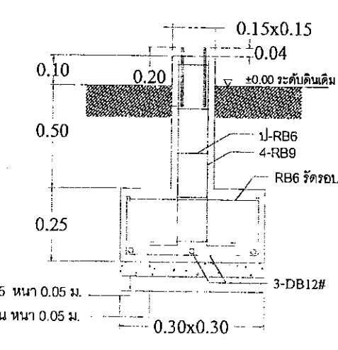
แบบขยายฐานราก F
