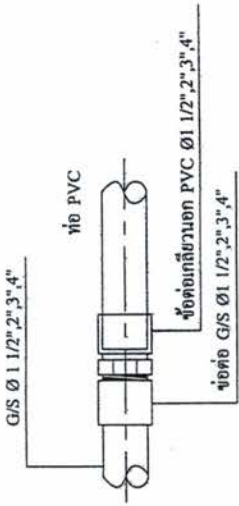
2. แบบการต่อท่อ G/S กับท่อ PVC
