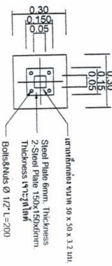
รูปขยายเสาเหล็ก CI
