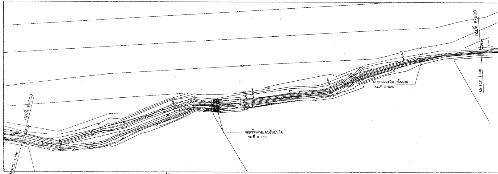
แปลนห้วยจระไซ่ กม.ที่ 8+000 ถึง กม.ที่ 8+600 มาตราส่วน 1:1,000
