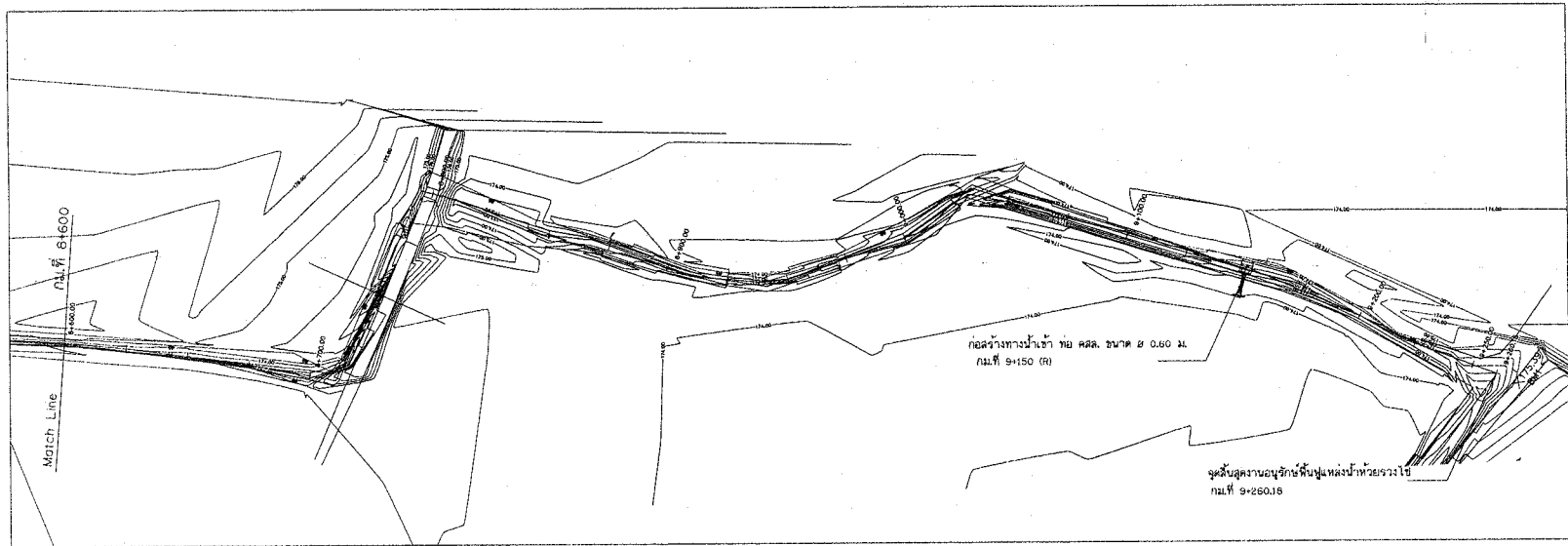
แปลนห้วยขวางไข่ กม.ที่ 8+600 ถึง กม.ที่ 9+260.18 มาตราส่วน 1:1,000
