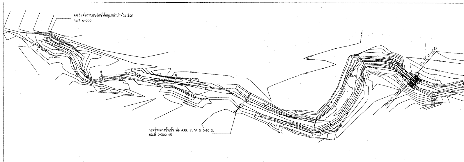
แปลนห้วยเขื่อน กม.ที่ 0+000 ถึง กม.ที่ 0+600 มาตราส่วน 1:1,000
