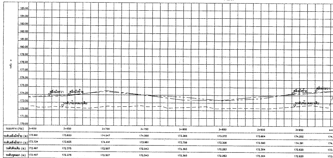
แนวลำน้ำห้วยเหือก กม.ที่ 3+600 ถึง กม.ที่ 3+996.30 มาตราส่วน 1:1,000
