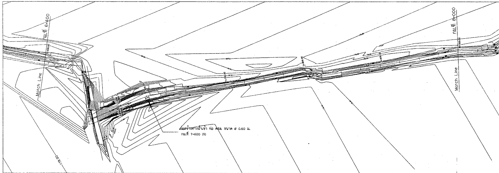
แปลนห้วยรวงไซ กม.ที่ 7+400 ถึง กม.ที่ 8+000 มาตราส่วน 1:1,000
