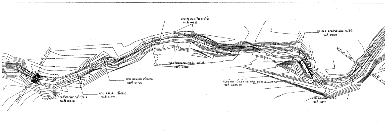
แปลนห้วยเข็ก กม.ที่ 0+600 ถึง กม.ที่ 1+200 มาตราส่วน 1:1,000
