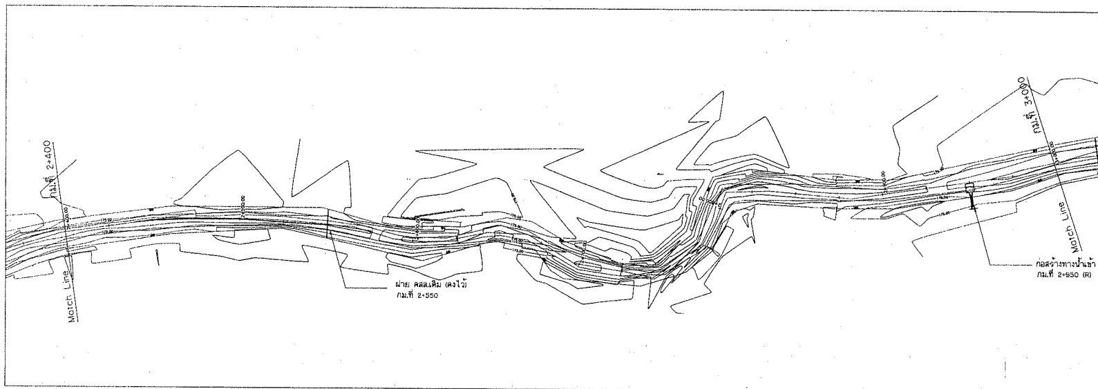
แปลนห้วยเหือก กม.ที่ 2+400 ถึง กม.ที่ 3+000 มาตราส่วน 1:1,000
