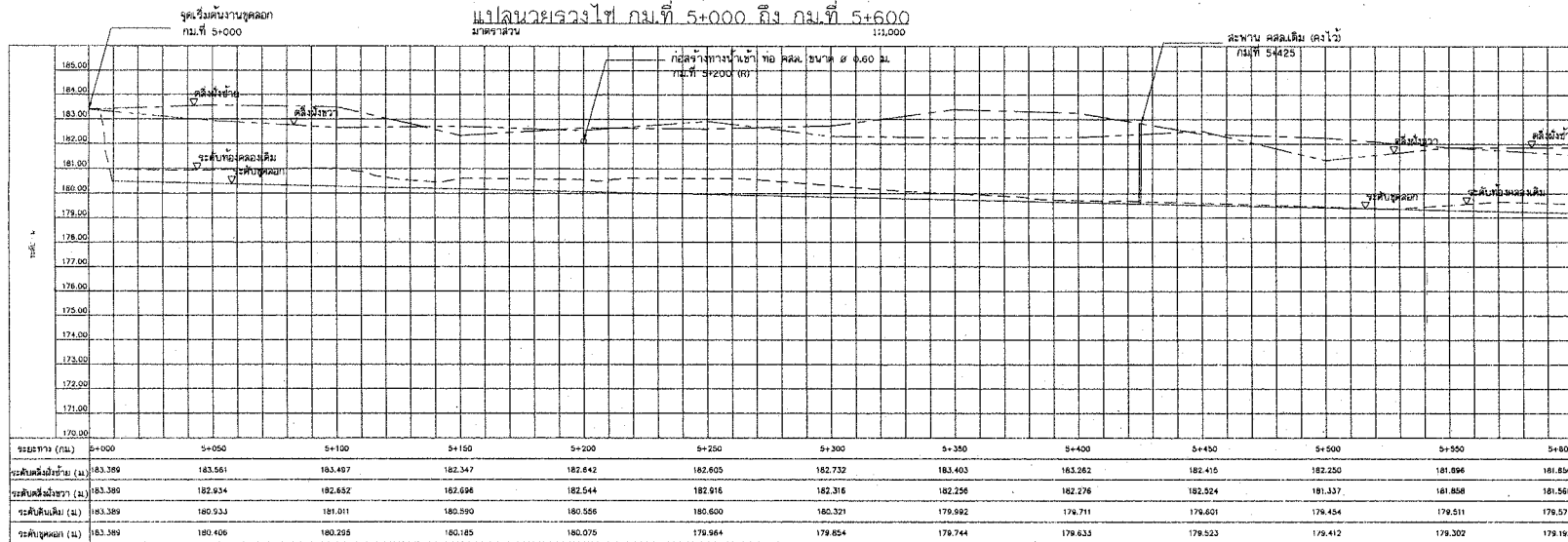
รูปตัดตามยาววางท่อ กม.ที่ 5+000 ถึง กม.ที่ 5+600
