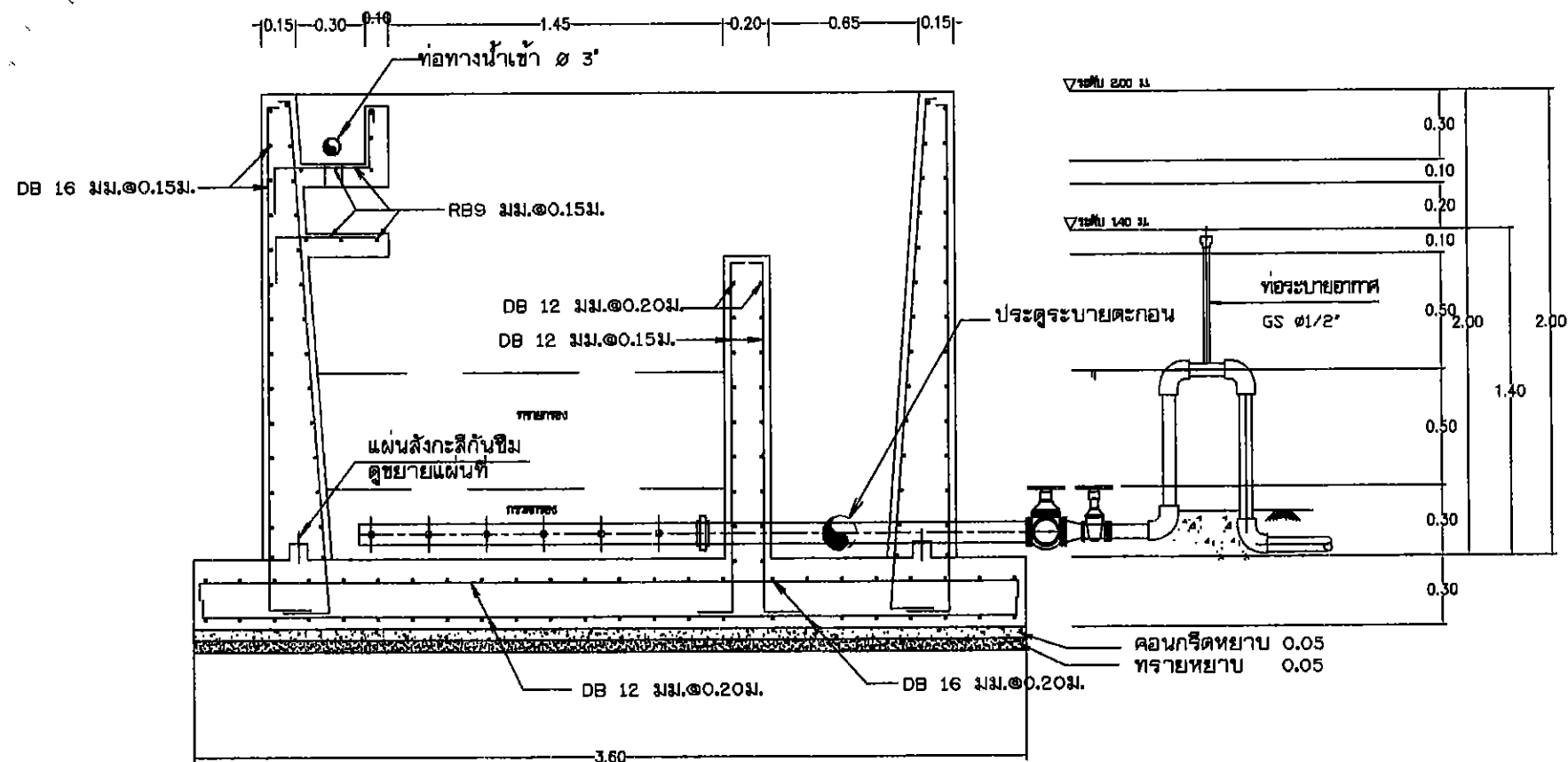
รูปตัด (จ) - (จ) 1:20
