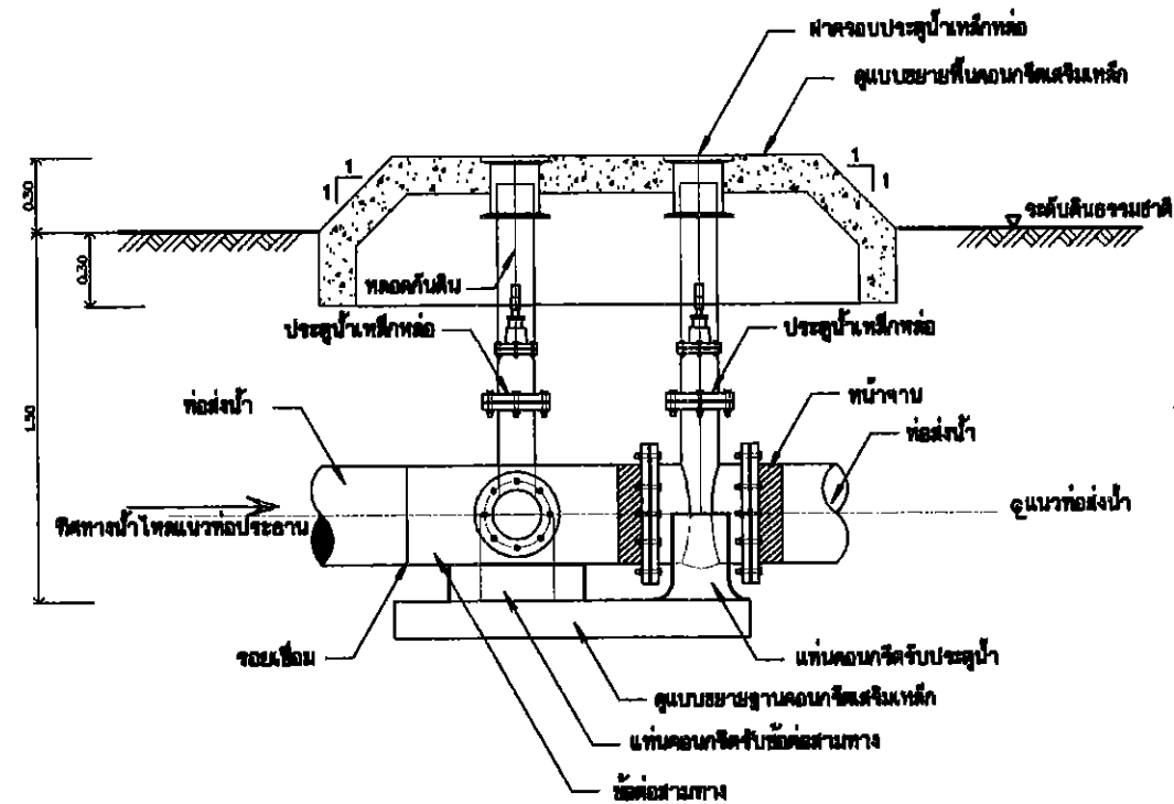
รูปตัดจุดแยก ( เข้าจุดรับน้ำ )
