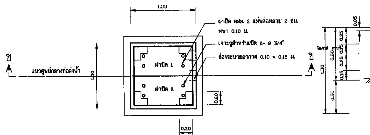
แปลนท่อระบายอากาศ
