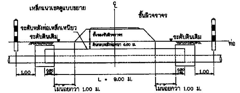
รูปตัดหัวไปท่อลอดถนน
