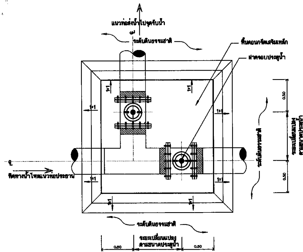
แปลนจุดแยก ( เข้าจุดรับน้ำ )
