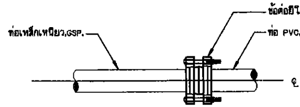
การบรรจุท่อเหล็กเหนียว, GSP กับท่อ PVC.
