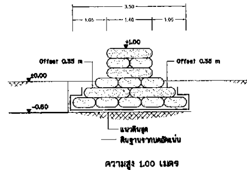
ฝายต้นน้ำแบบถูทราย (รูปตัด ข-ข) มาตราส่วน 1:50
