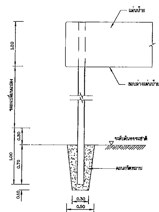
รายละเอียดการติดตั้งเสาป้าย 1:20
