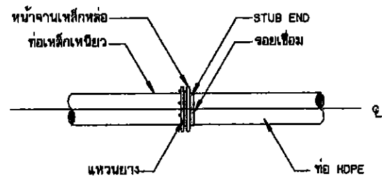
การบรรจุท่อเหล็กเหนียว, GSP กับท่อ HDPE
