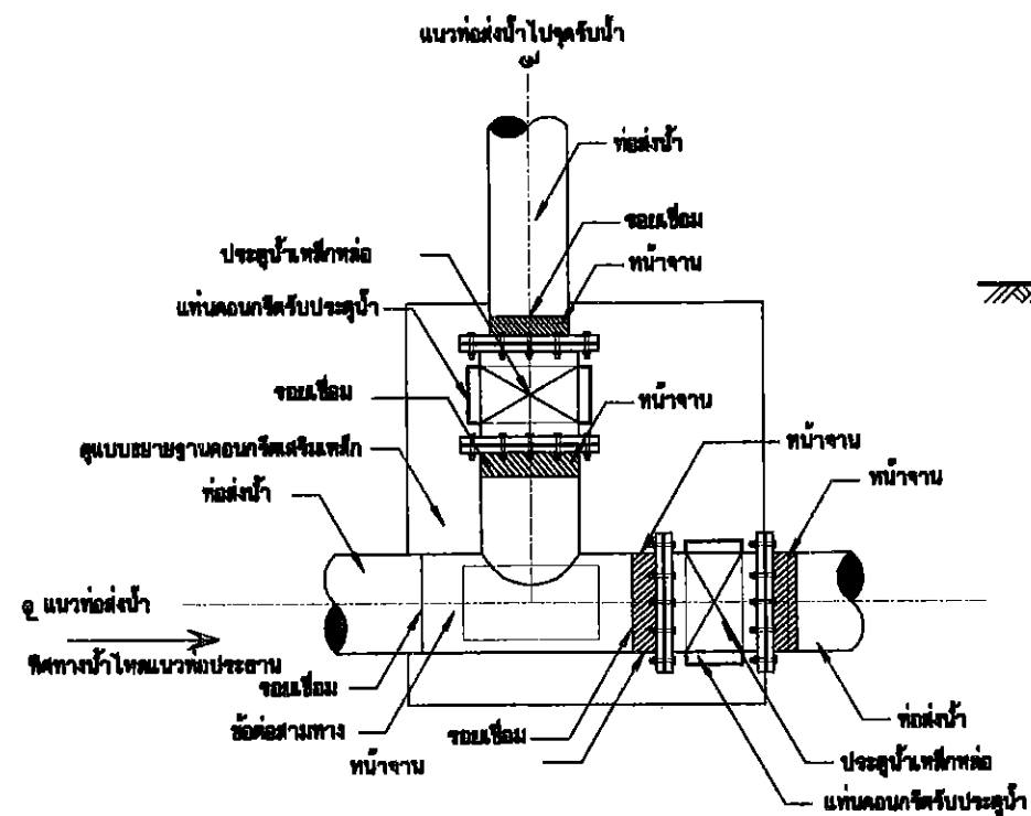
รูปขยายการติดตั้งจุดแยก ( เข้าจุดรับน้ำ )
