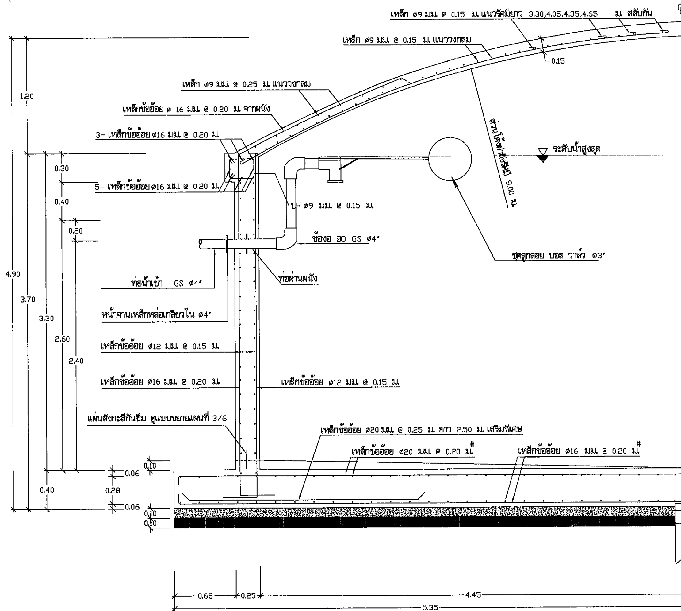
รูปตัด ขยาย (ข) - (ข) 1:25
