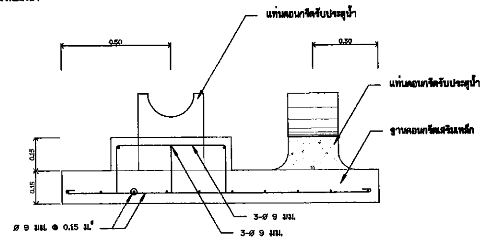
รูปตัด ก - ก
