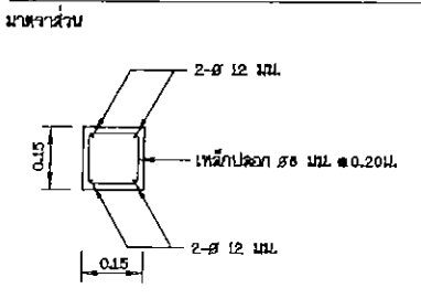
รูปตัด ก - ก 1:10
