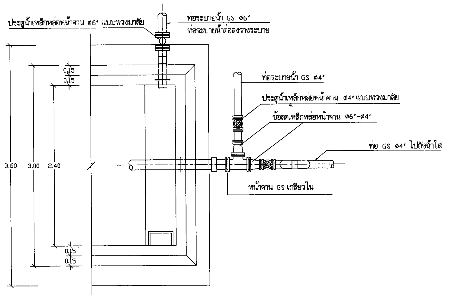
แบบขยายการประสานท่อออกจากถังกรองตะกอน 1 : 30
