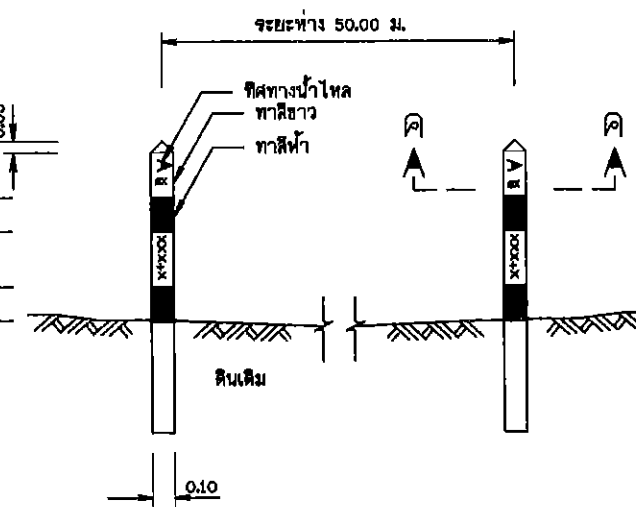
รูปขยายหลักแนวท่อ คสล.
