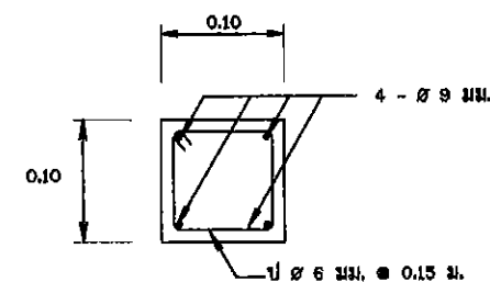
รูปตัด ค - ค
