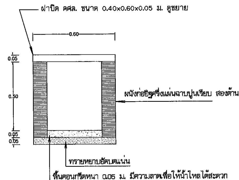
แบบขยาย รางระบายน้ำ -
