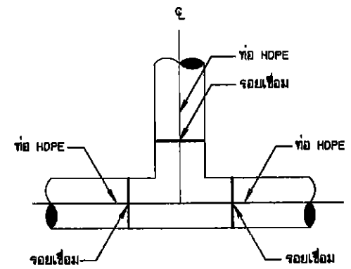
การต่อเชื่อมท่อ HDPE กับท่อ HDPE
