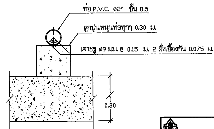
แบบขยายการประสานท่อออกจากถังกรองตะกอน 1 : 30
