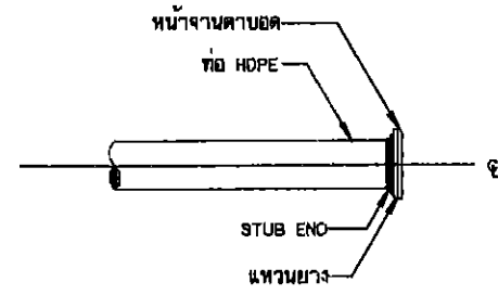
การปิดปลายท่อ
