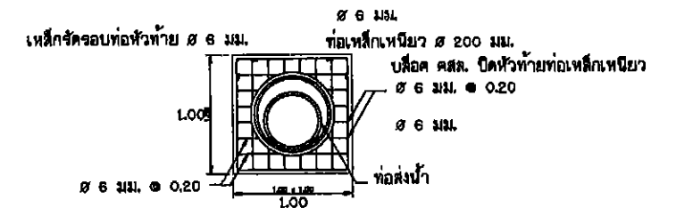
รูปตัดตามขวาง A-A
