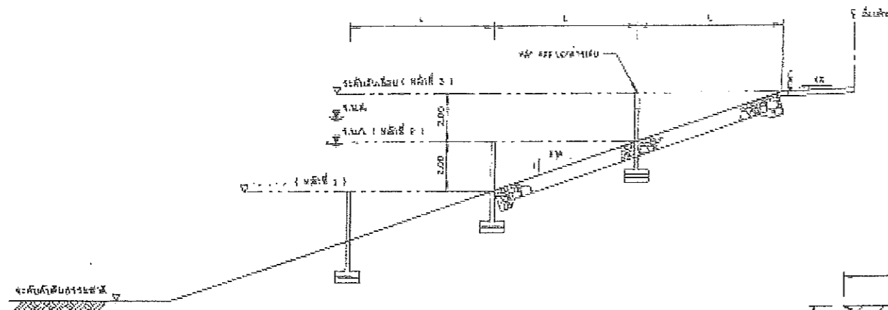
รูปตัดทั่วไปแสดงตำแหน่งหลักบ่อค่าระดับน้ำ มาตราส่วน 1:100
