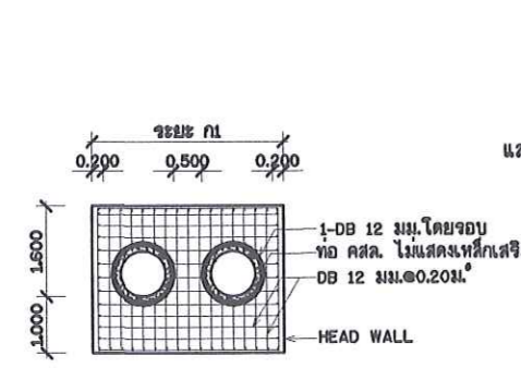
ขยายการเสริมเหล็กกำแพงท้ายท่อ
