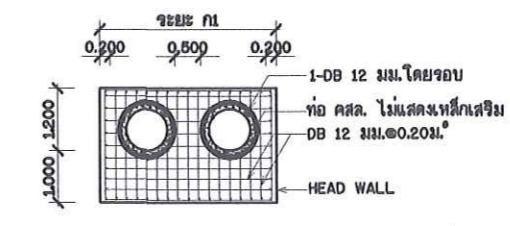
ขยายการเสริมเหล็กกำแพงปากท่อ มาตราส่วน 1:100
