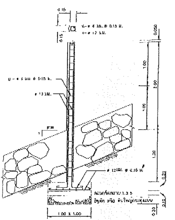
ขยายหลัก คสล.บ่อค่าระดับ มาตราส่วน 1:25
