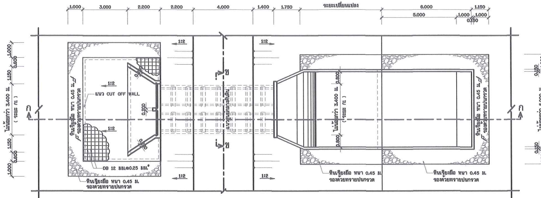
แปลนอาคารระบายน้ำ 2-Ø 1.00 m. มาตราส่วน 1:100
