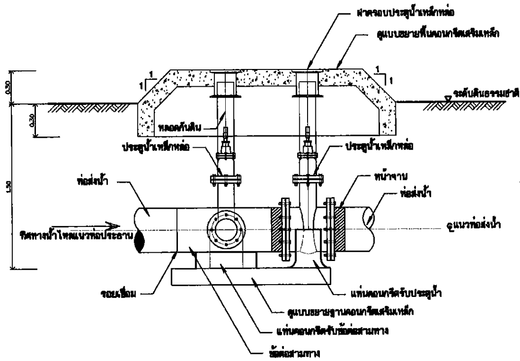
รูปตัดจุดแยก (เข้าจุดรับน้ำ)
