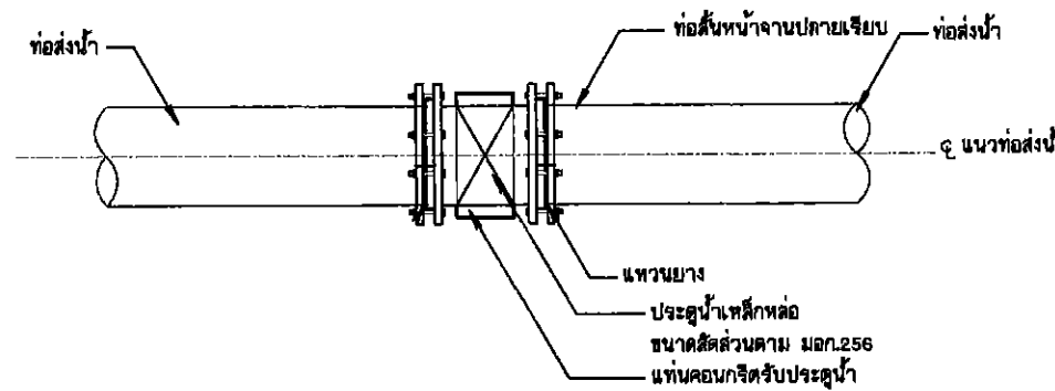
รูปขยายการติดตั้งประตุน้ำเชื่อมแนวท่อ
