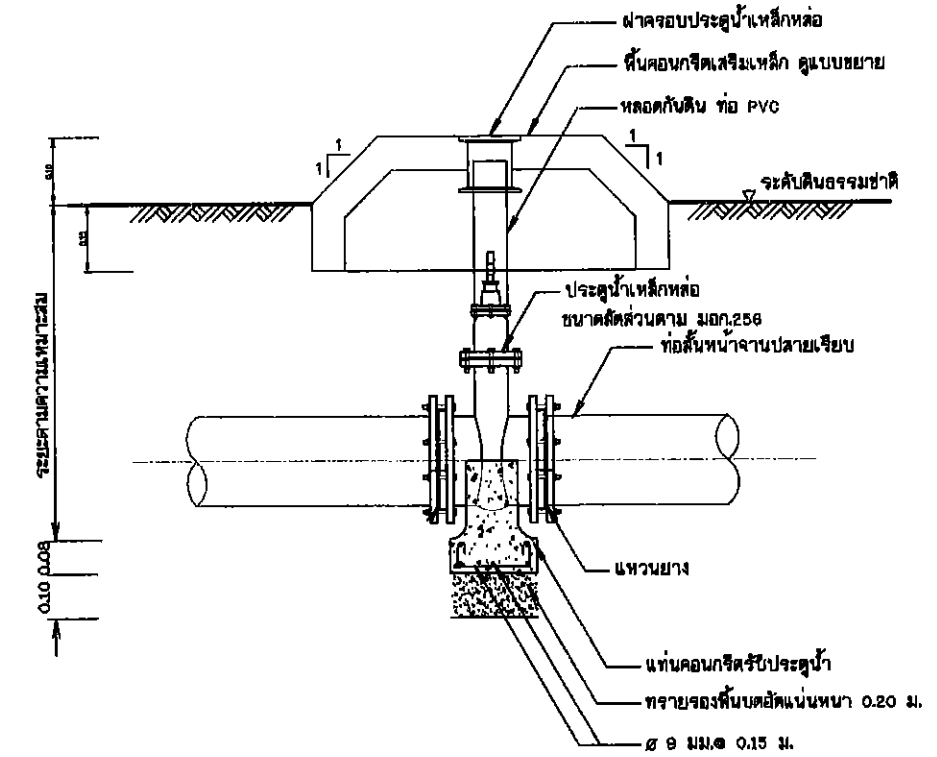
รูปตัดประตุน้ำเชื่อมกับระบบท่อ
