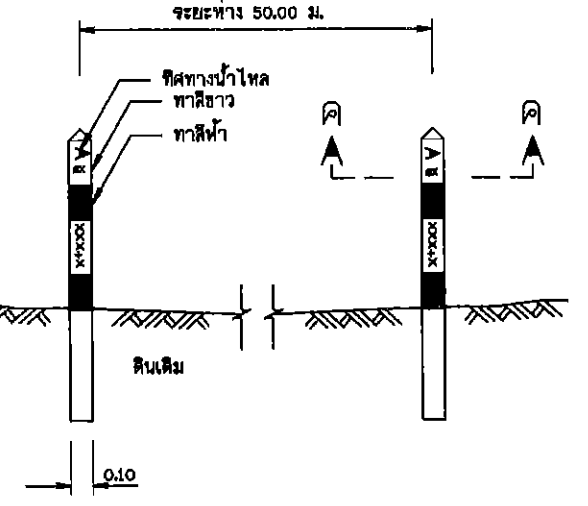
รูปขยายหลักแนวท่อ คสล. มาตราส่วน 1 : 25
