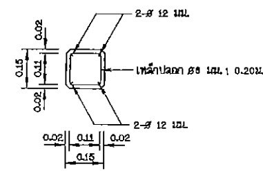
รูปตัด ข - ข 1:90 (หน้า) 1:10
