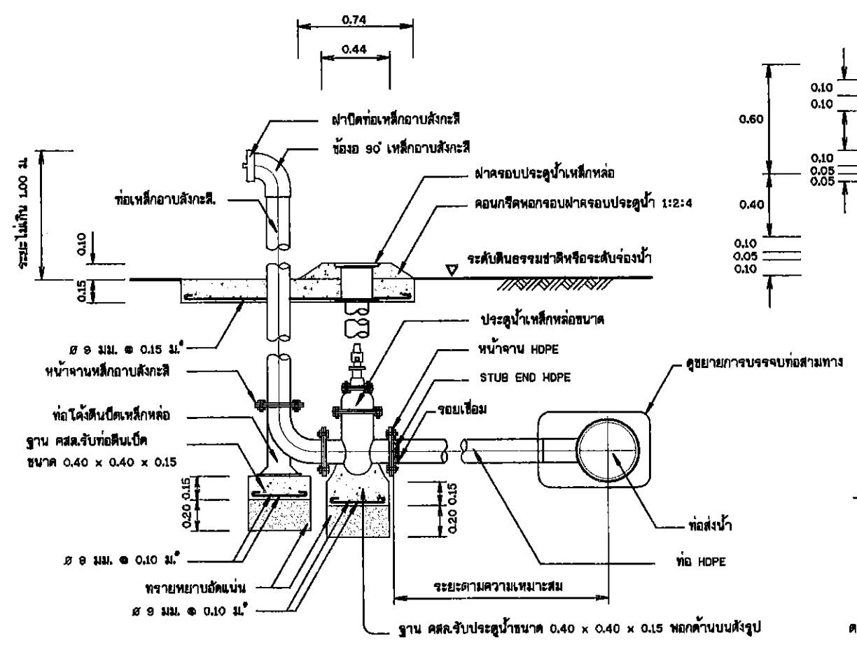
รูปตัด ก - ก แสดงการติดตั้งประตูระบายตะกอน มาตราส่วน 1 : 25
