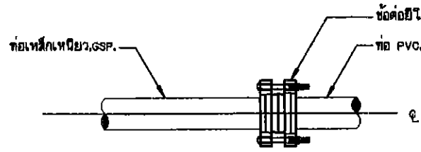
การบรรจุท่อเหล็กเหนียว, GSP กับท่อ PVC.
