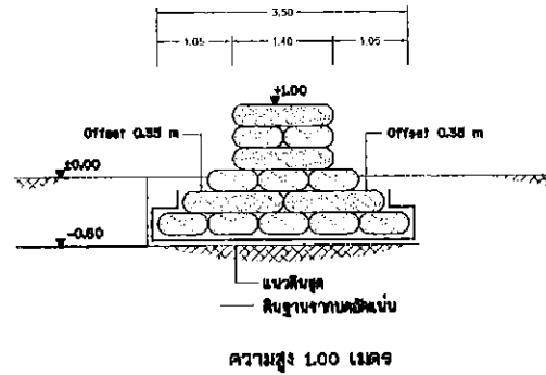
ฝายต้นน้ำแบบถุงทราย (รูปตัด ข-ข) มาตราส่วน 1:50
