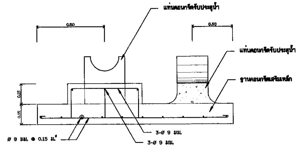
รูปตัด ก - ก
