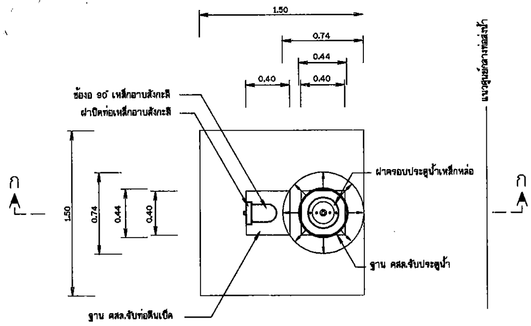
แปลนประตูระบายตะกอน มาตราส่วน 1 : 25
