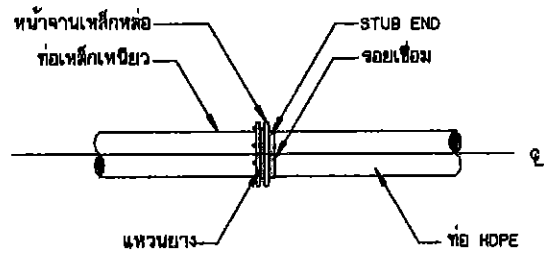
การบรรจุท่อเหล็กเหนียว, GSP กับท่อ HDPE
