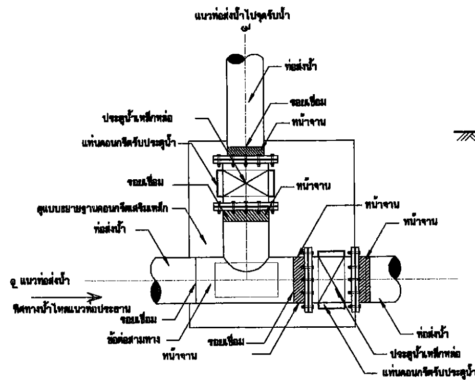
รูปขยายการติดตั้งจุดแยก (เข้าจุดรับน้ำ)
