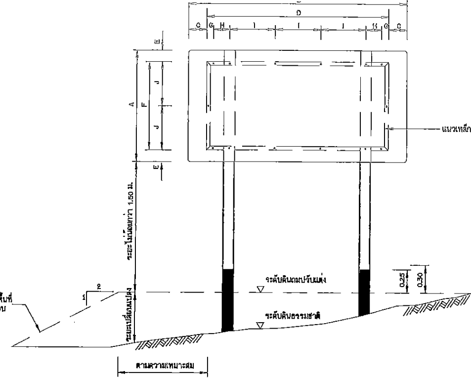
รูปแสดงการประกอบแผ่นป้าย 1:90 (หน้า) 1:20
