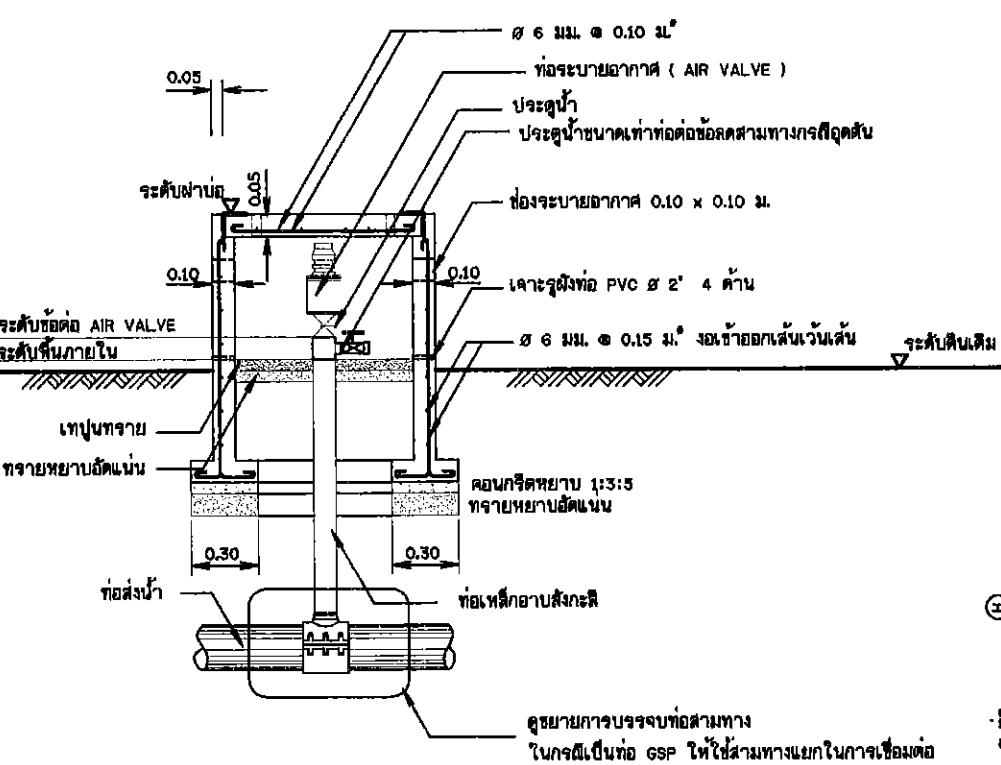
รูปตัด ข - ข แสดงการติดตั้งท่อระบายอากาศ มาตราส่วน 1 : 25
