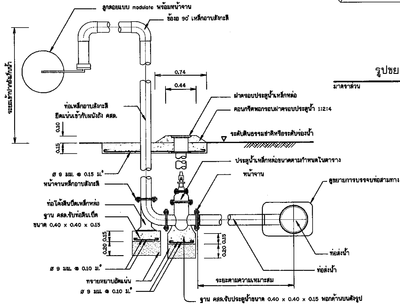
รูปตัด ก - ก แสดงการติดตั้งประตูจุดปล่อยน้ำ
