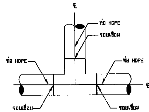
การต่อเชื่อมท่อ HDPE กับท่อ HDPE
