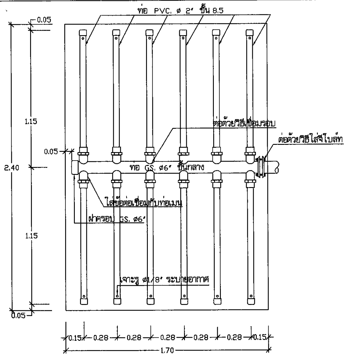
แบบขยายท่อแกงปลา 1:20
