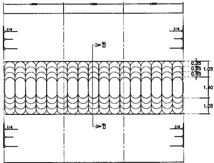
แปลน มาตราส่วน 1:100
