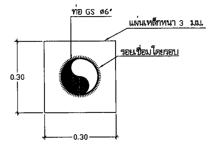
ขยายท่อผ่านผนัง 1 : 10
