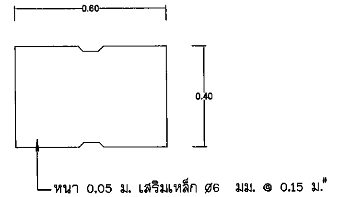
แบบฝาปิด คสล. -
