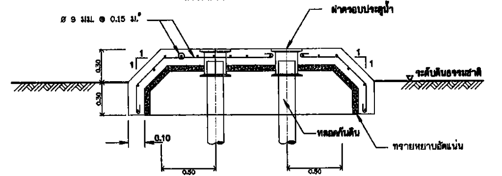
รูปตัด ก - ก
