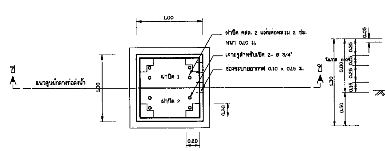
แปลนท่อระบายอากาศ มาตราส่วน 1 : 25
