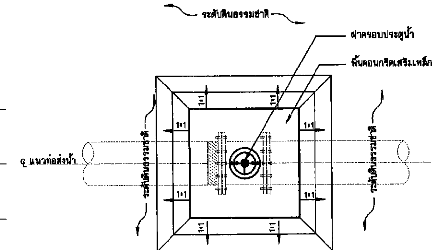
รูปตัดประตุน้ำเชื่อมกับระบบท่อ
