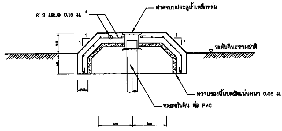
รูปขยายการเสริมเหล็กพื้นคอนกรีตเสริมเหล็ก
