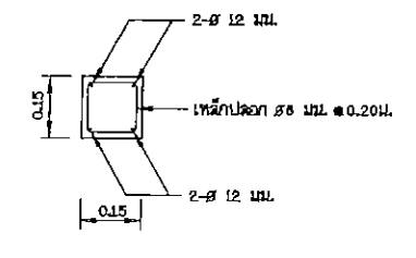
รูปตัด ก - ก 1:90 (หน้า) 1:10
