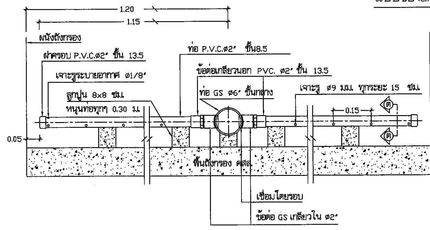
แบบขยายท่อแกงปลา 1:20
