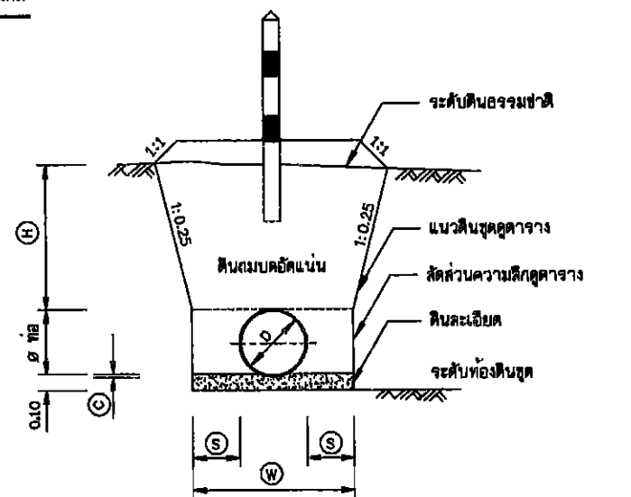
รูปตัดทั่วไปแสดงการวางท่อ มาตราส่วน -
