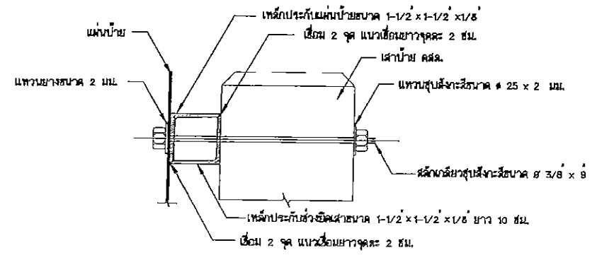
รูปตัดขยายการยึดแผ่นป้ายและเสา 1:90 (หน้า) 1:20
