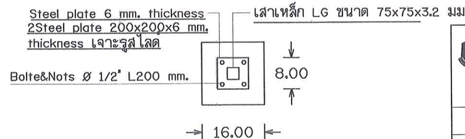
รูปขยาย C1
