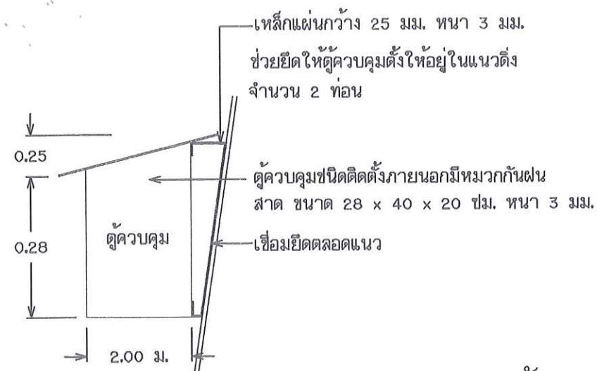
แบบขยายตัวควบคุม มาตราส่วน 1 : 10
