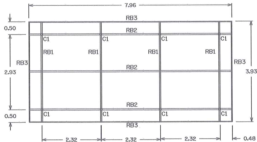
แปลนคานโครงหลังคา
