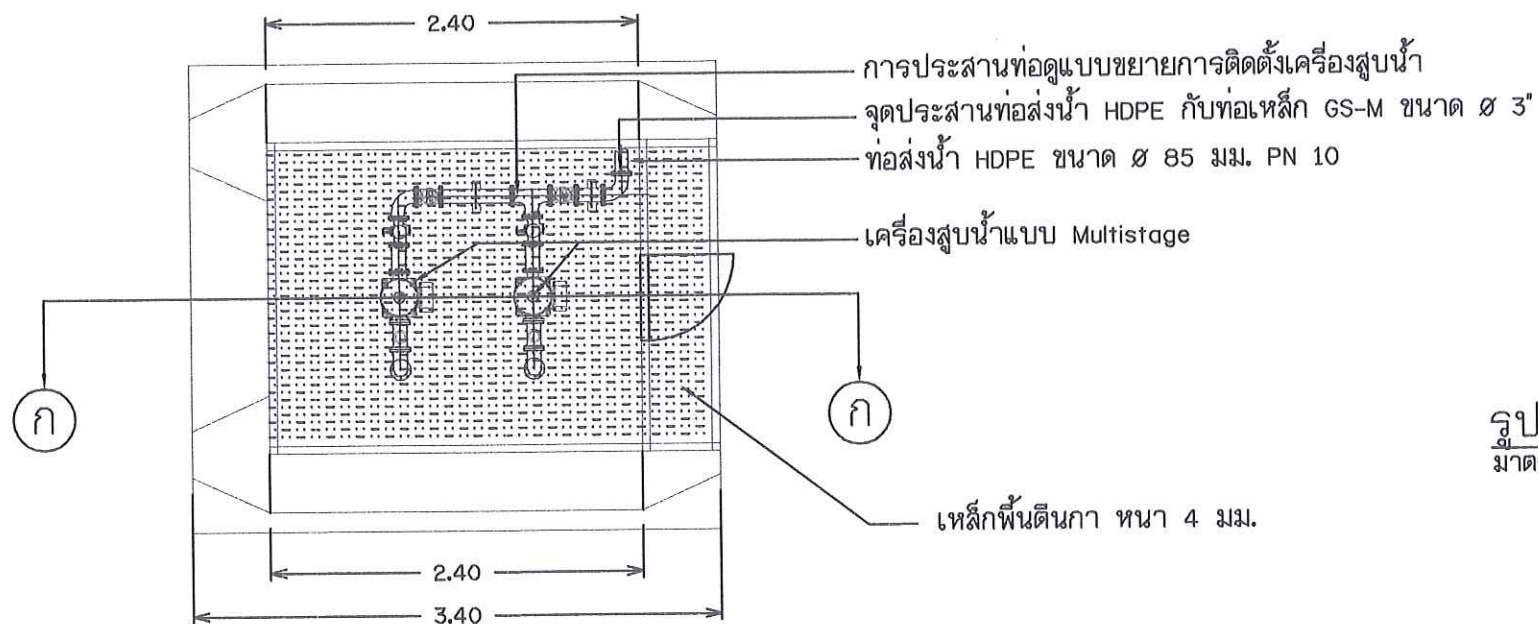
แปลนพื้นแพท่อนลอย มาตราส่วน 1:50
