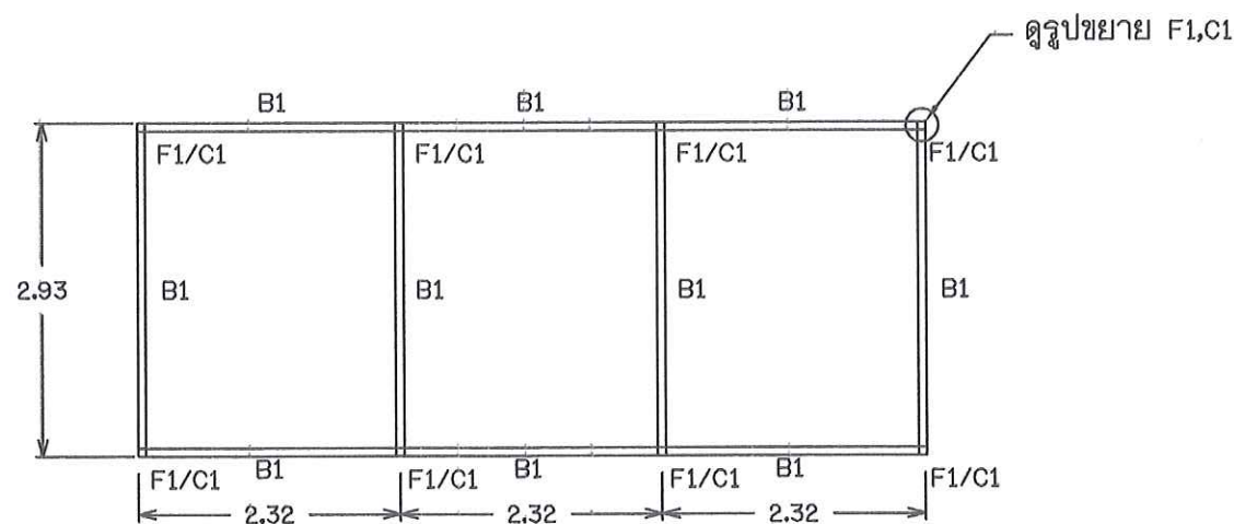
แปลนฐานรากและคานเหล็ก
