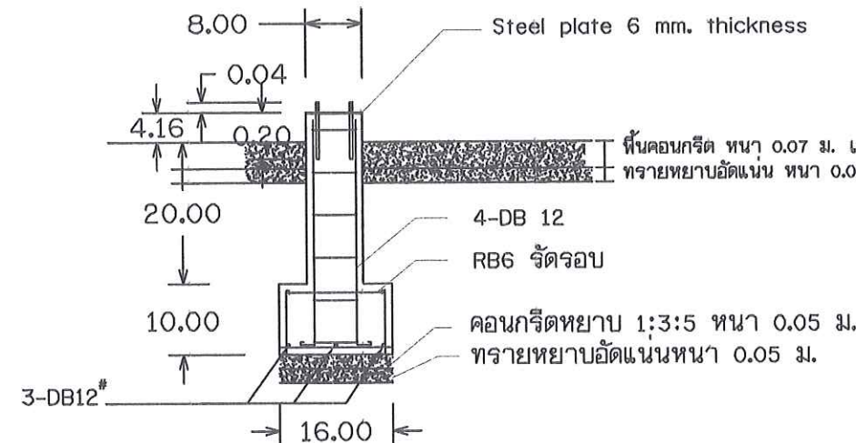
รูปขยาย F1
