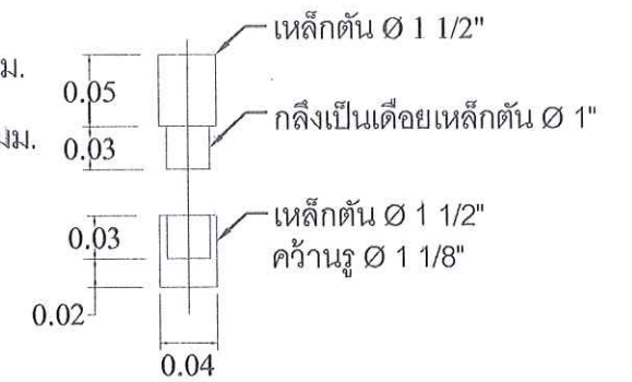
แบบขยายบานพับประตูเหล็ก
