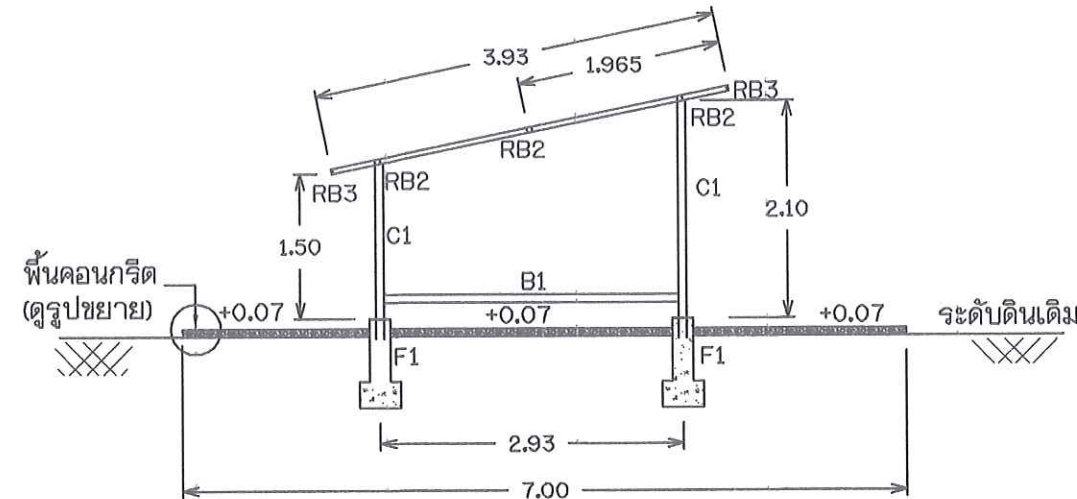
รูปตัดโครงรับแรง
