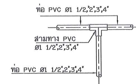
15. แบบการต่อสามทาง PVC
