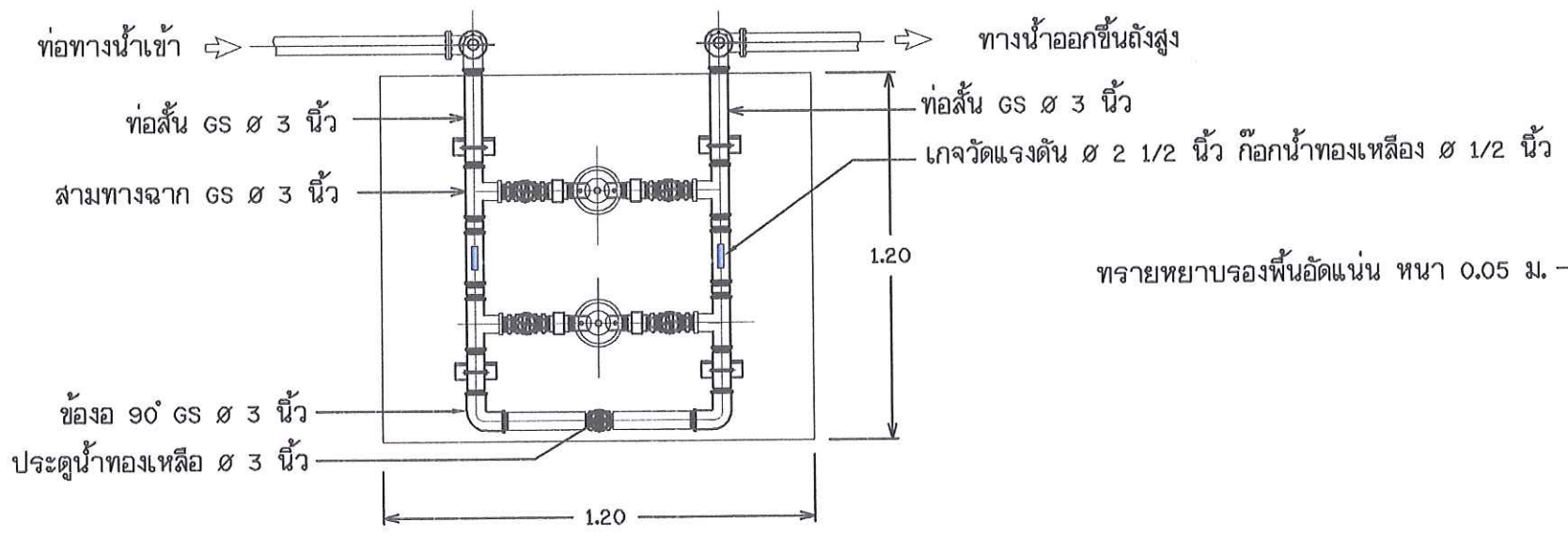
แปลนระบบกรองเศษตร มาตราส่วน not to scale
