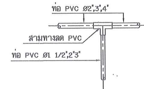
13. แบบการต่อสามทางลด PVC
