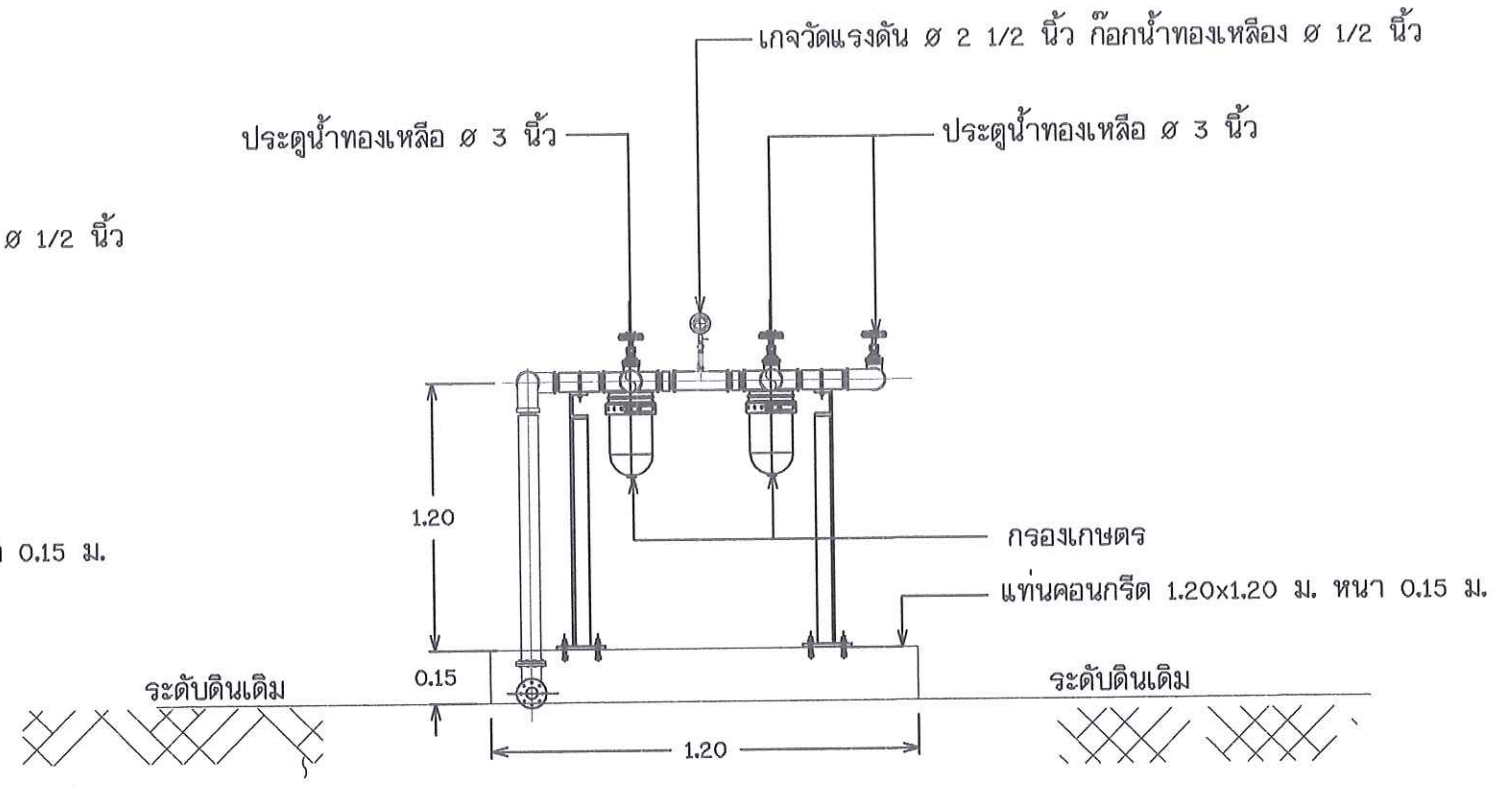
รูปด้านข้าง มาตราส่วน not to scale
