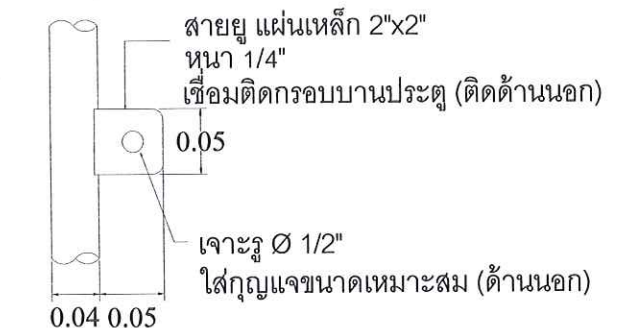
แบบขยายสายยู
