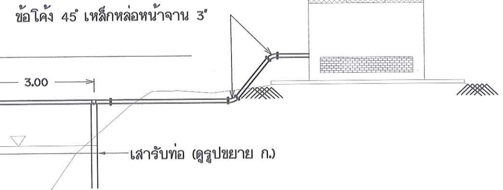
18. แบบการติดตั้งท่อดูด
