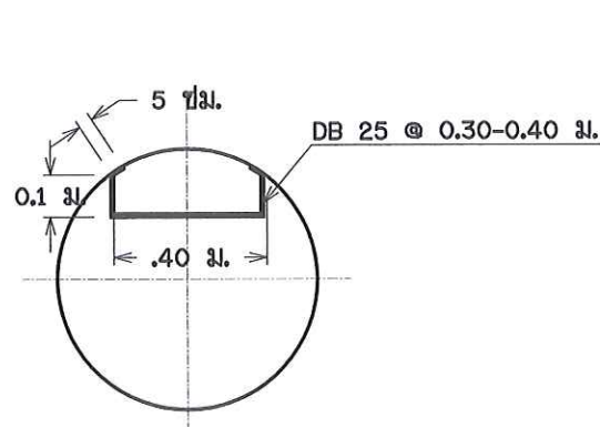
รูปขยายบันไดภายในส่วน column
