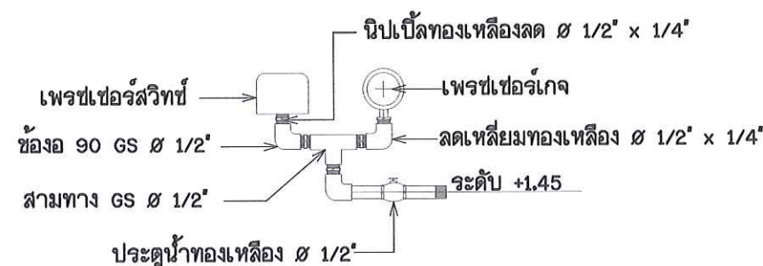
แบบขยายสวิตช์ควบคุมและเกจวัดความดัน
