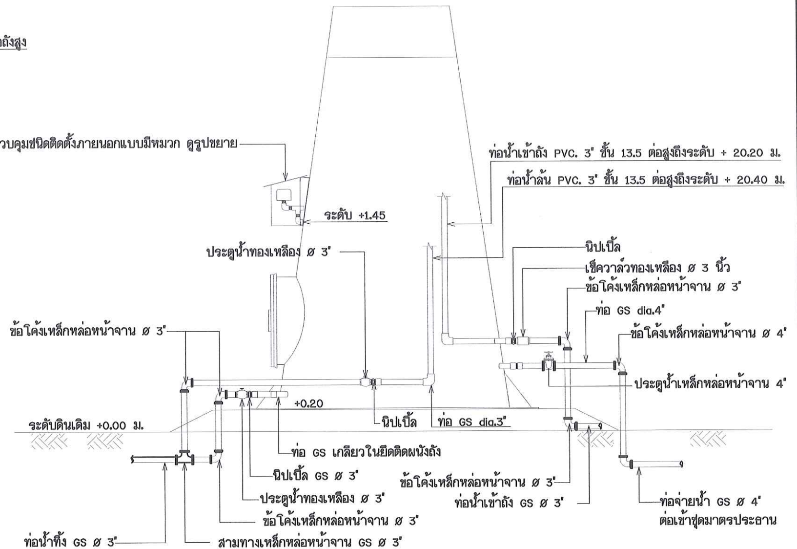
แบบแสดงการเดินท่อในห้องสูง มาตราส่วน 1 : 25
