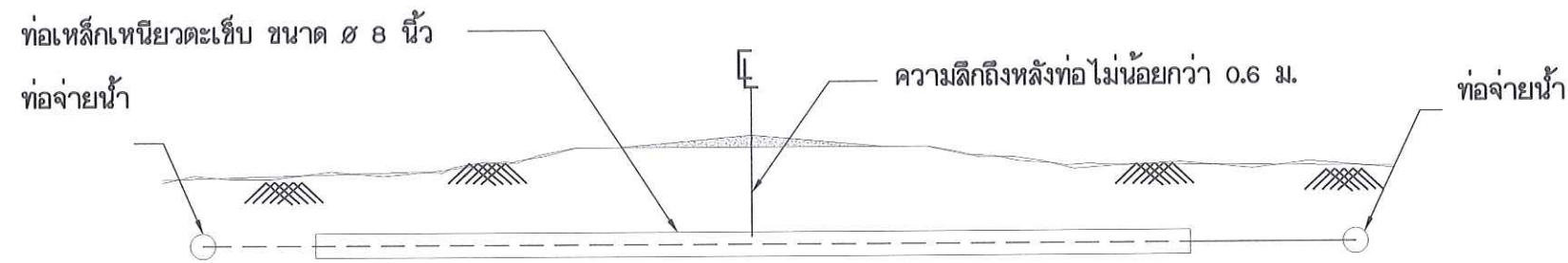
12. การเดินท่อใต้ถนน ท่อ ๒, 3, 4, 6"
