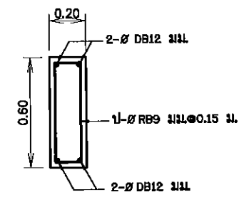
แบบขยาย 1 ขยายคานคอดิน GB1
