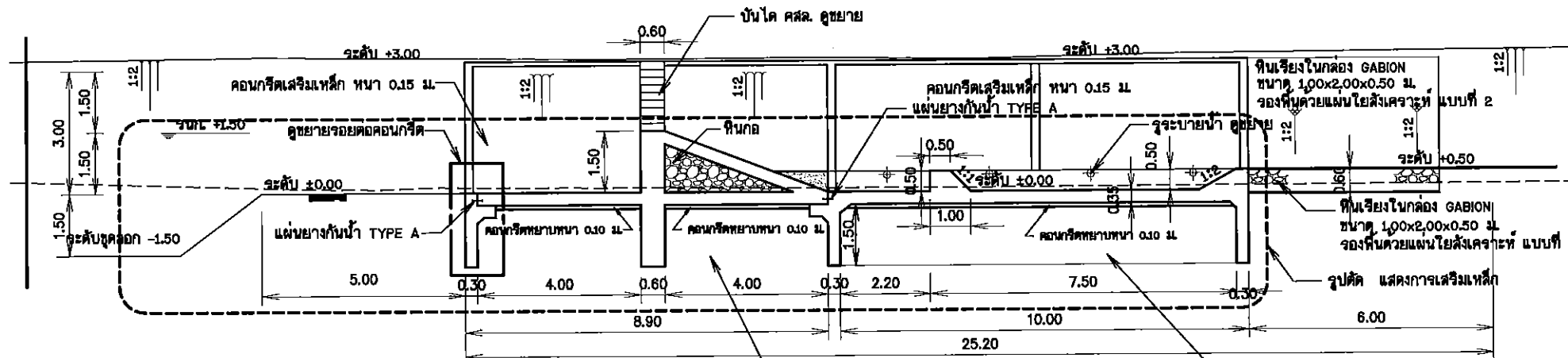
รูปตัด ข - ข
