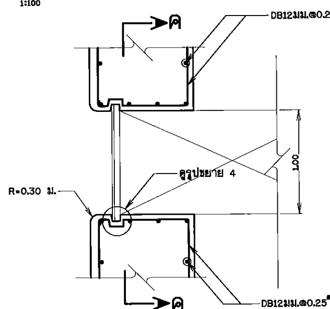
รูปขยายช่องระบายทราย
