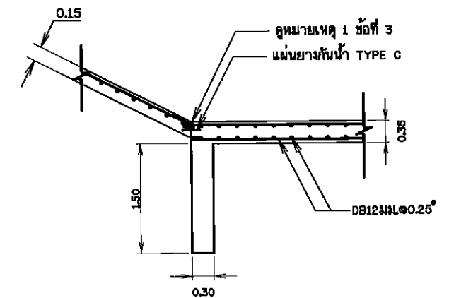
รูปขยาย 3
