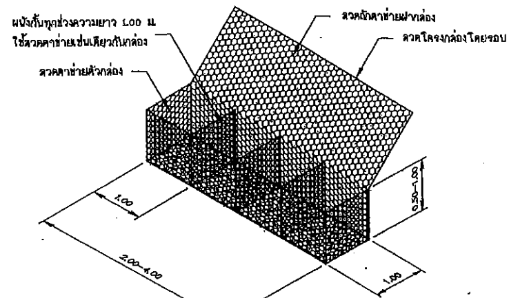
กล่องลวดตาข่ายแบบ GABION
