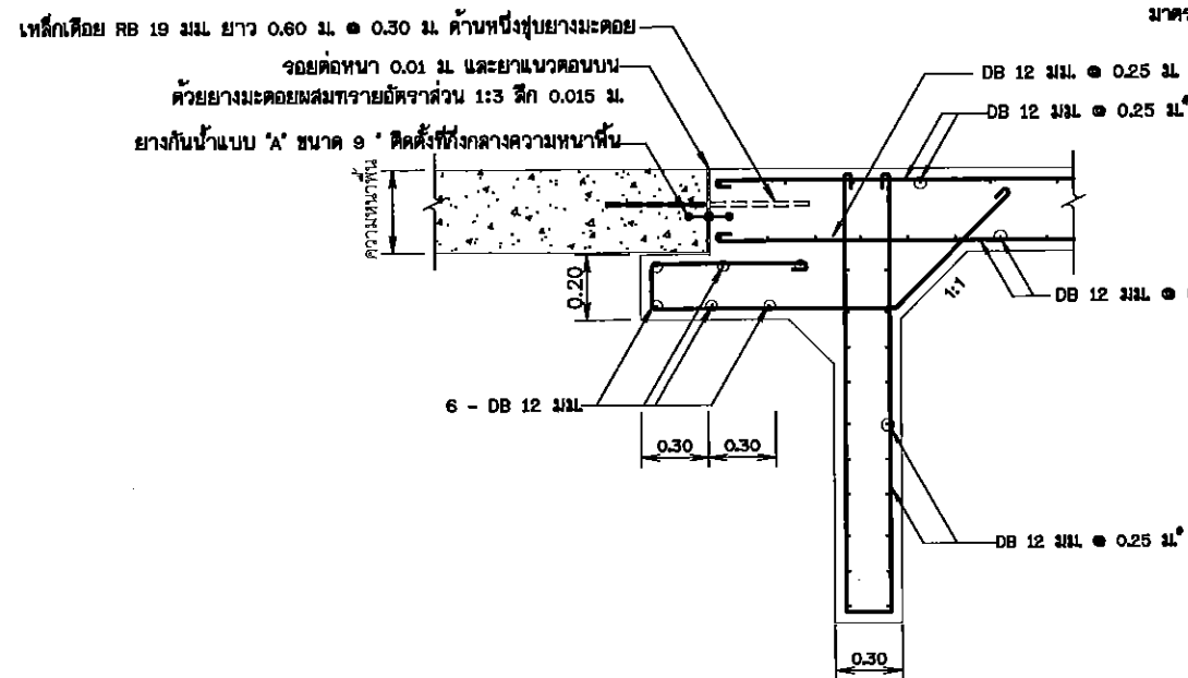
รูปขยายรอยต่อคอนกรีต A
