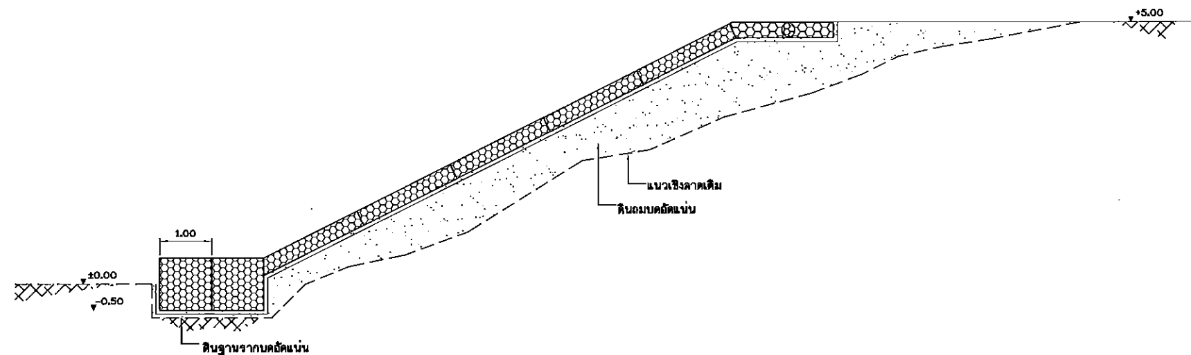
ความสูง 5.00 เมตร ระบบป้องกันการกัดเซาะริมตลิ่งแบบวางเรียงด้วยเกเบียนและแมทเทรล กรณีปรับความลาดชันของผิวหน้าเชิงลาดเท่ากับ 1:2 (ตั้ง : ราบ) รูปแบบที่ 2 มาตราส่วน 1:50
