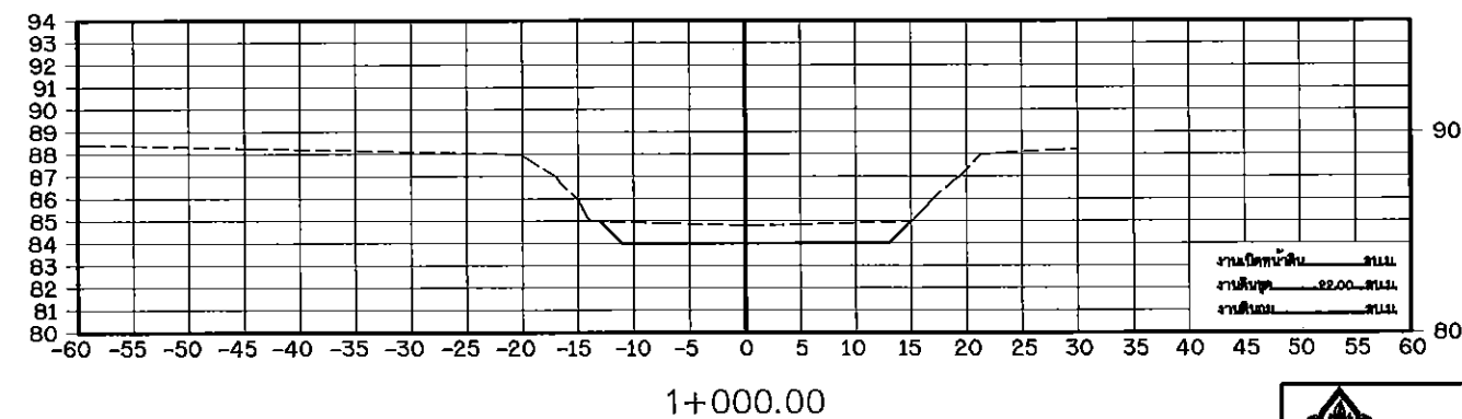
รูปตัดตามขวางแสดงงานดิน มาตราส่วน 1:250
