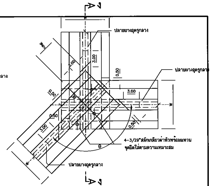
การต่อมุมกันทั้ง 3 ชั้น ไม่แสดงขนาดส่วน
