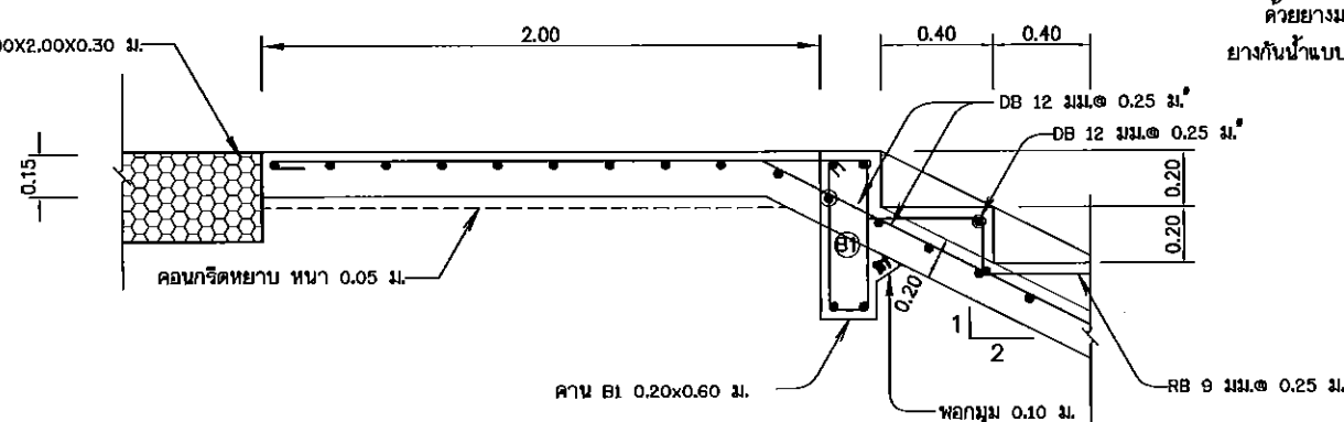
แบบขยาย ①
