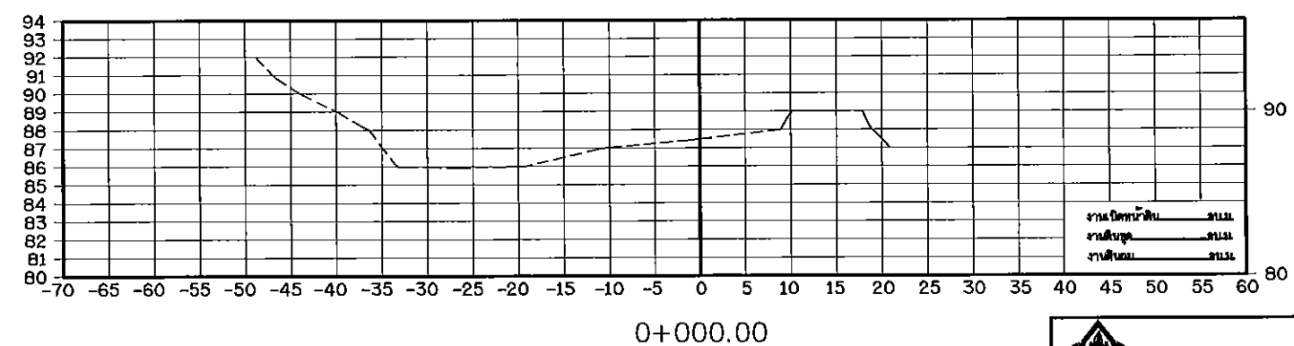
รูปตัดตามขวางแสดงงานดิน มาตราส่วน 1:250
