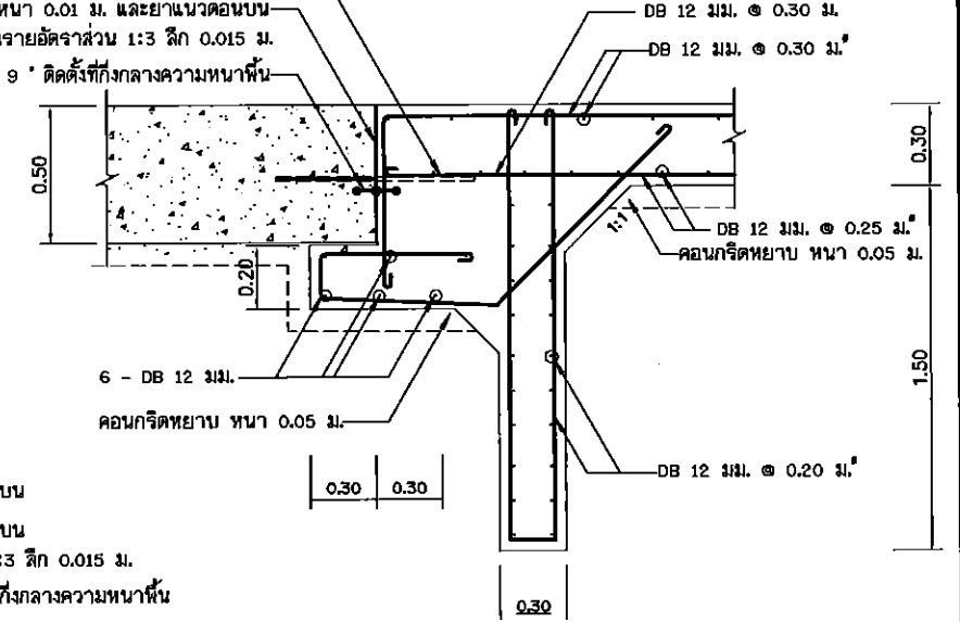
รูปขยายรอยต่อคอนกรีต
