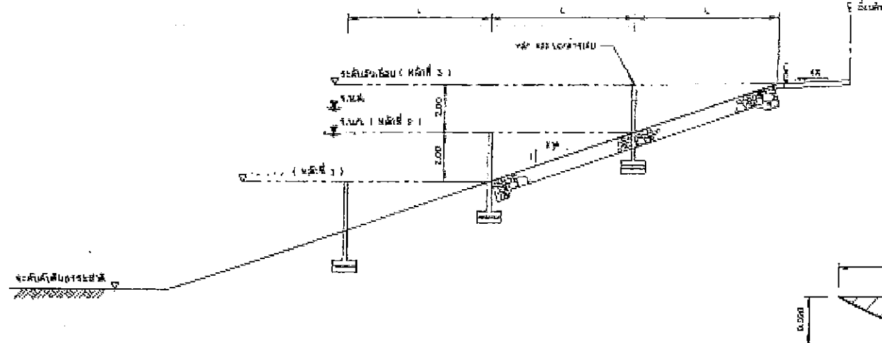
รูปตัดทั่วไปแสดงตำแหน่งหลักบอกค่าระดับน้ำ
