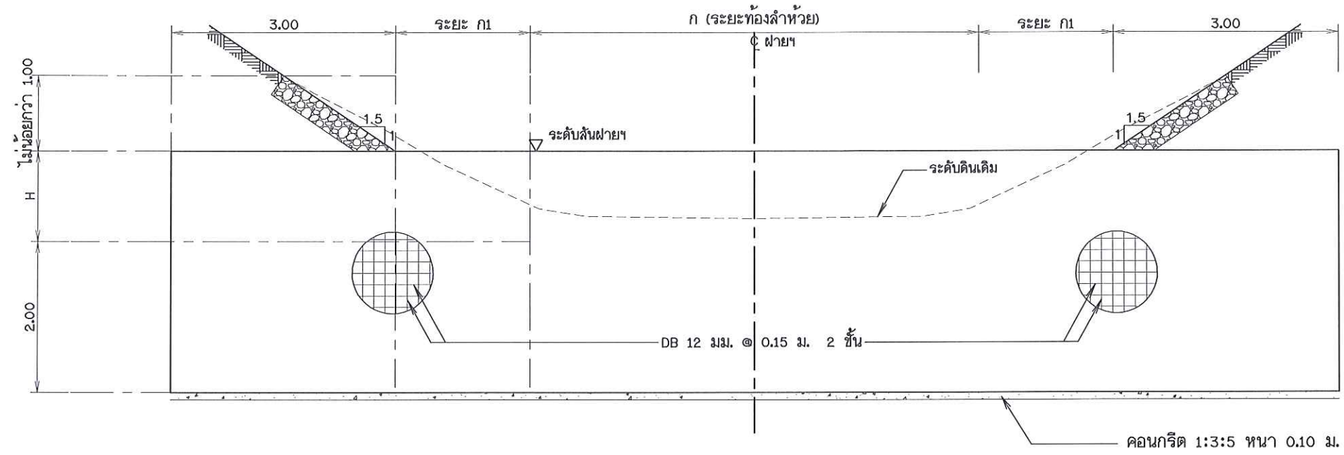
รูปตัด ข-ข มาตราส่วน 1:50
