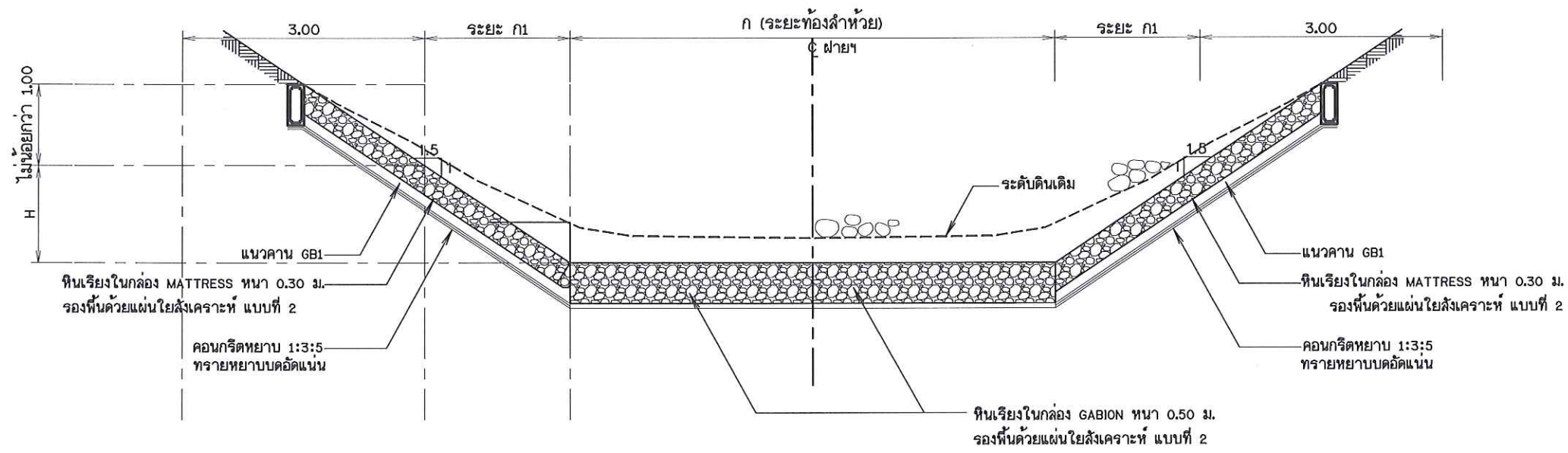
รูปตัด ค-ค มาตราส่วน 1:50
