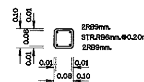
รูปตัด ข - ข มาตรฐาน 1:10
