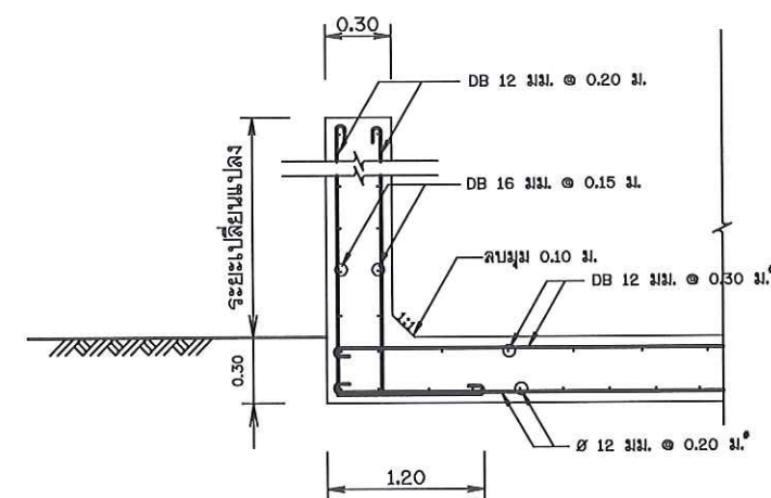
รูปตัด " 10 "
