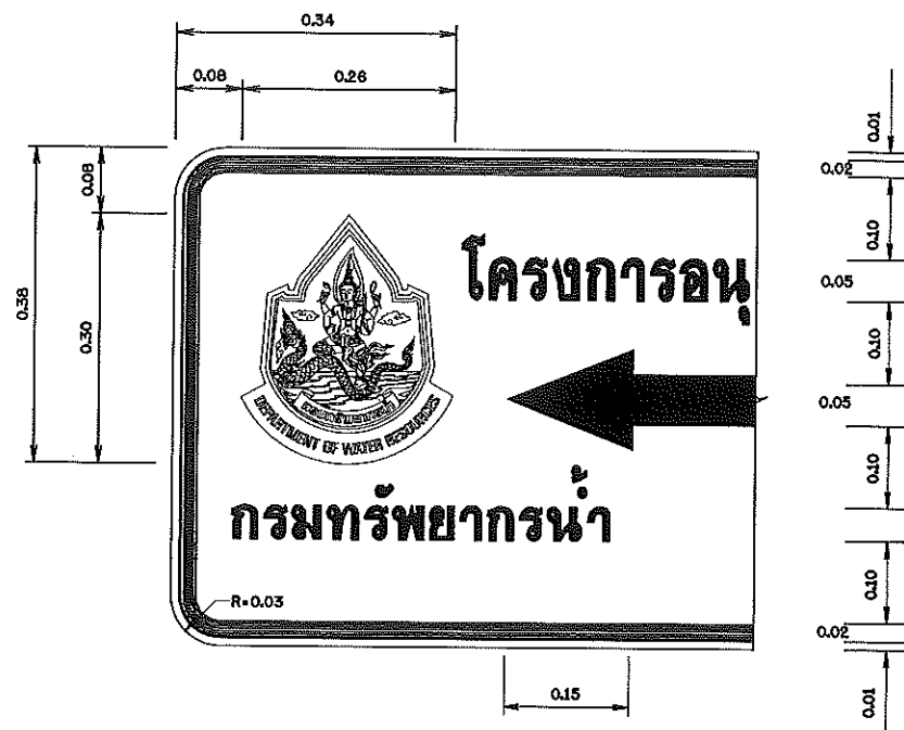
รูปขยายตราสัญลักษณ์ มาตรฐาน 1:15
