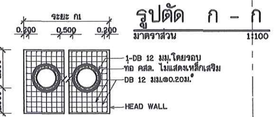
ขยายการเสริมเหล็กกำแพงปากท่อ มาตราส่วน 1:100
