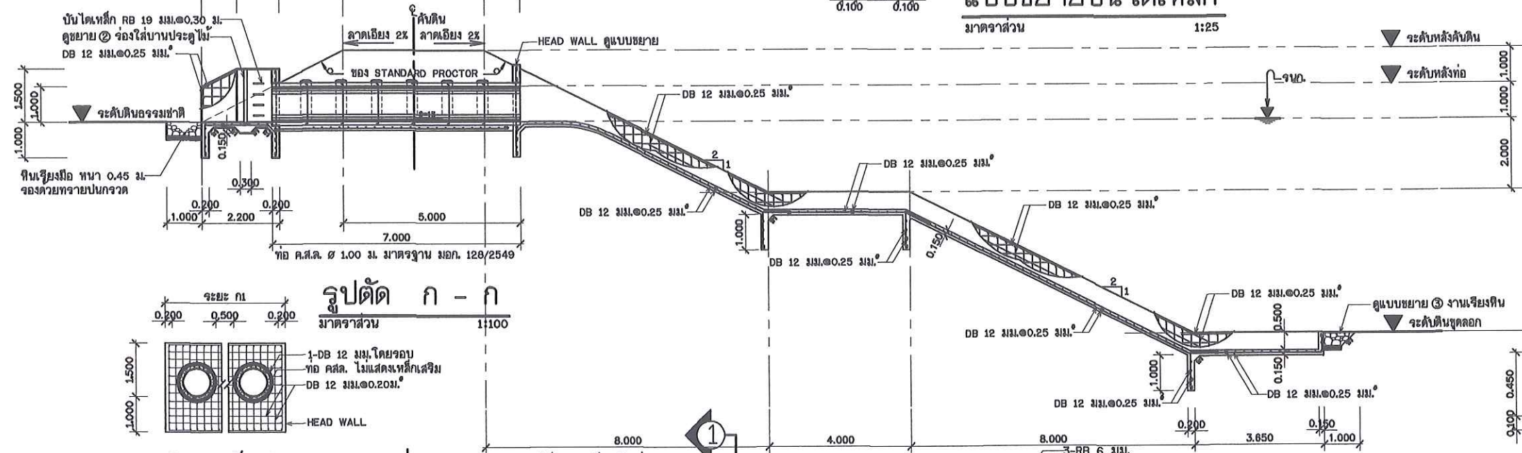
ขยายการเสริมเหล็กกำแพงปากท่อ มาตราส่วน 1:100
