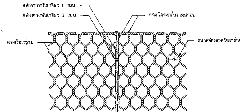
รูปแสดงการพันลวดระหว่างกล่องลวดตาข่ายและฟาบิต
