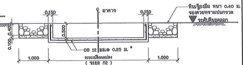
รูปตัด ค - ค มาตราส่วน 1:50
