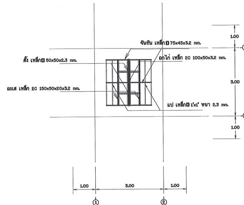
แปลนหลังคา
