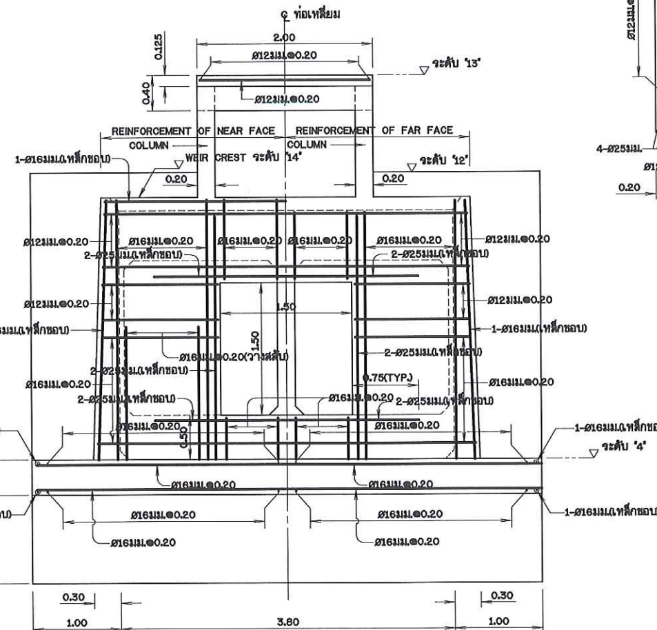
รูปตัด ค-ค มาตราส่วน 1:30
