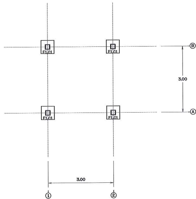
แปลนฐานราก
