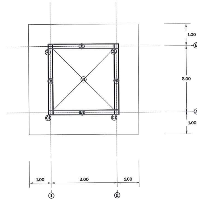
แปลนคาน
