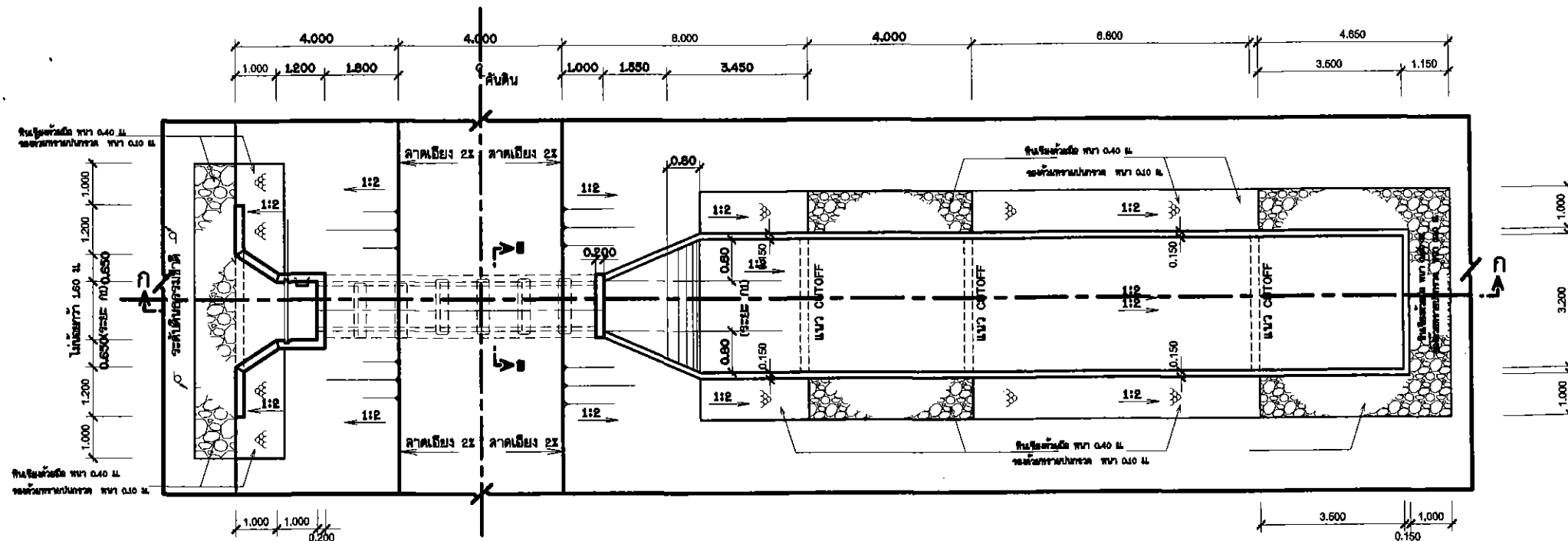
แปลนอาคารท่อทางน้ำเข้า
