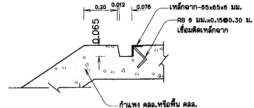
ขยายร่องใส่บานประตูไม้
