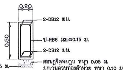
ขยายคานคอดิน GB1
