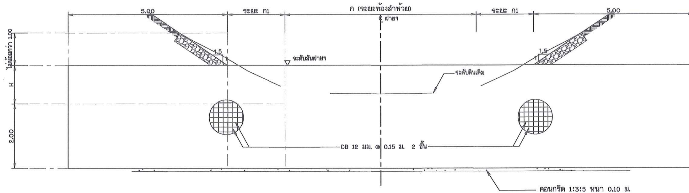
รูปตัด ข-ข
