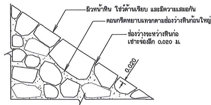
ขยายคอนกรีตฉาบพื้นใหญ่
