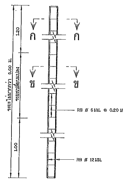
รายละเอียดย่อยราย คสส.
