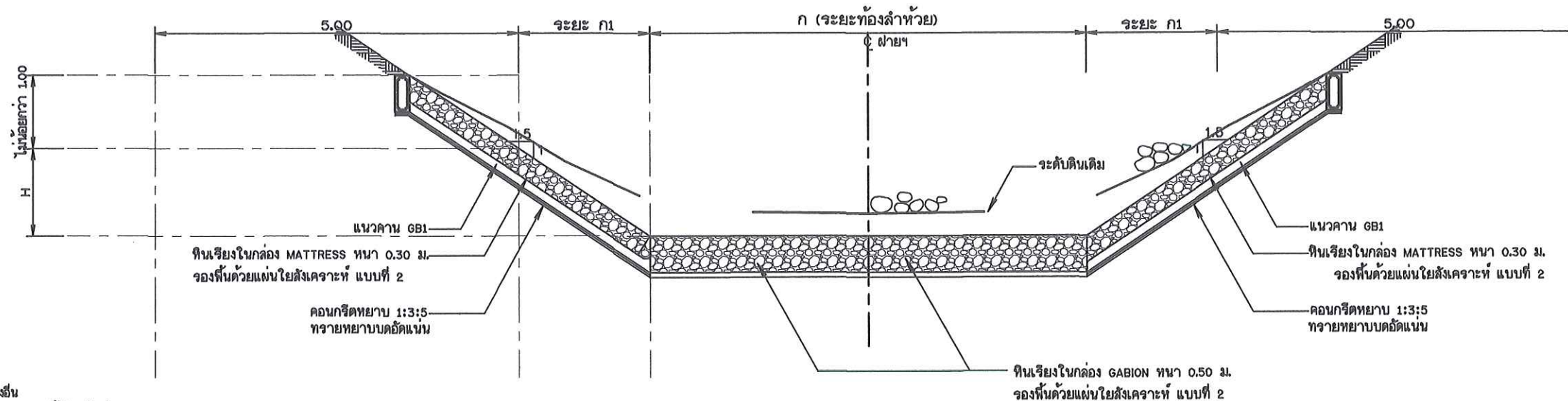
รูปตัด ค-ค
