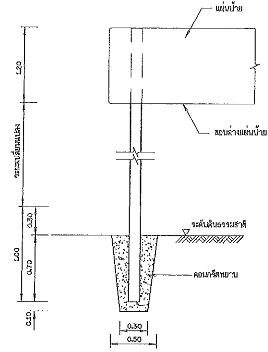
รายละเอียดการติดตั้งเสาป้าย นางสาว..... 1:20
