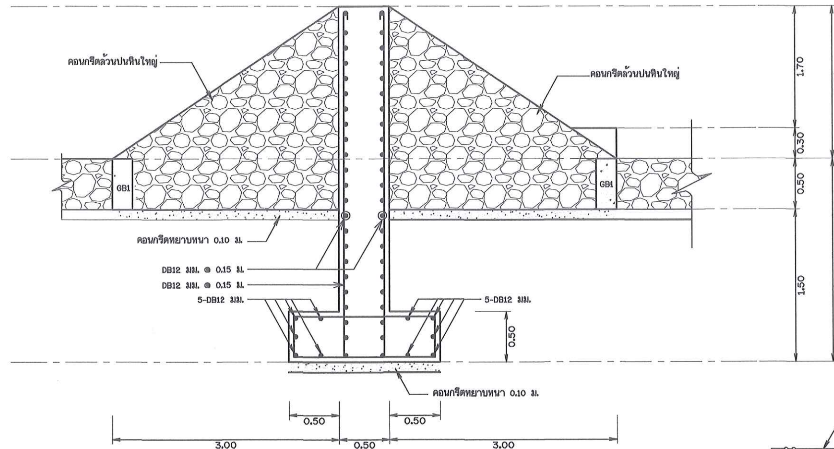
รูปตัดแสดงการเสริมเหล็กแกนฝายฯ
