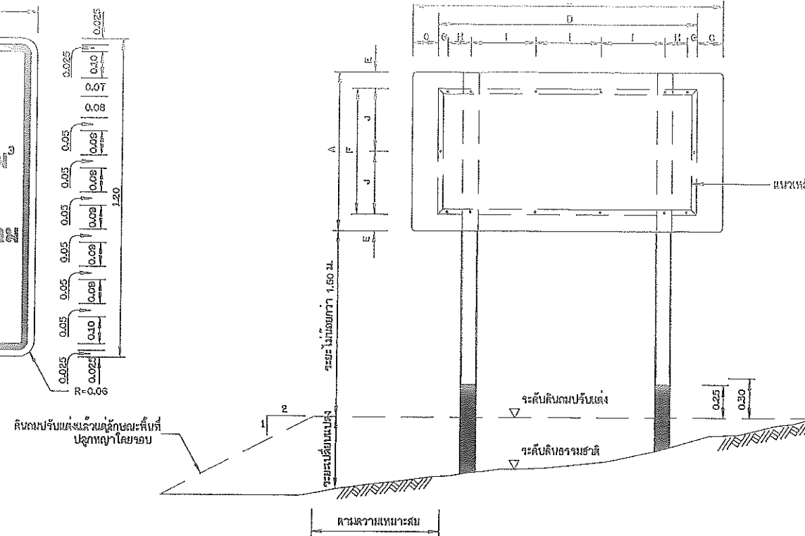
รูปแสดงการประกอบแผนปาย ๒๕๕๐ ๑๕:๒๐
