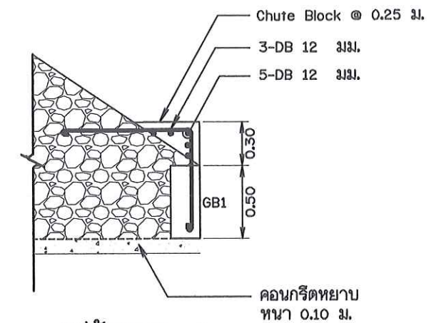
รูปตัดขยาย 1 มาตราส่วน 1:25
