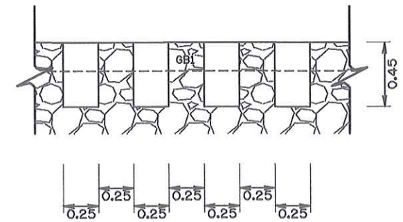
แปลนขยาย 1 มาตราส่วน 1:25
