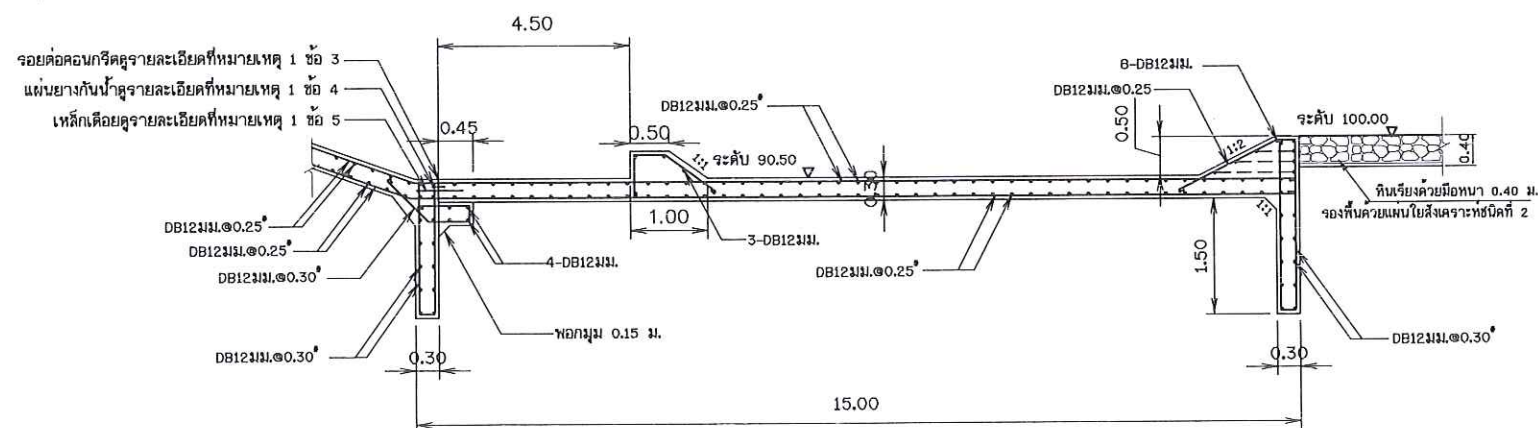
รูปขยาย 2 มาตราส่วน 1:50
