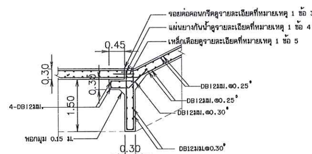
รูปขยาย 3 มาตราส่วน 1:50
