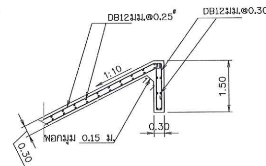
รูปขยาย 4 มาตราส่วน 1:50
