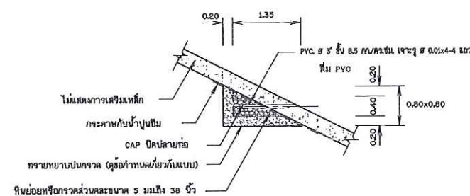
แบบขยาย รุระบายน้ำ B มาตราส่วน 1:50
