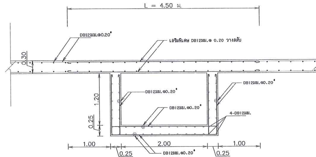
รูปตัด ค-ค มาตราส่วน 1:25
