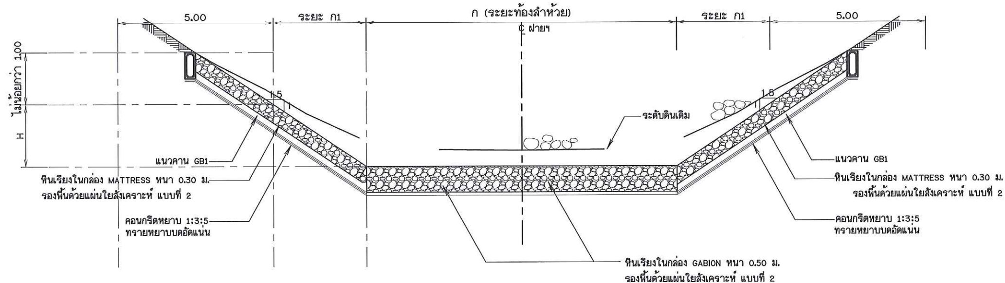
รูปตัด ค-ค
