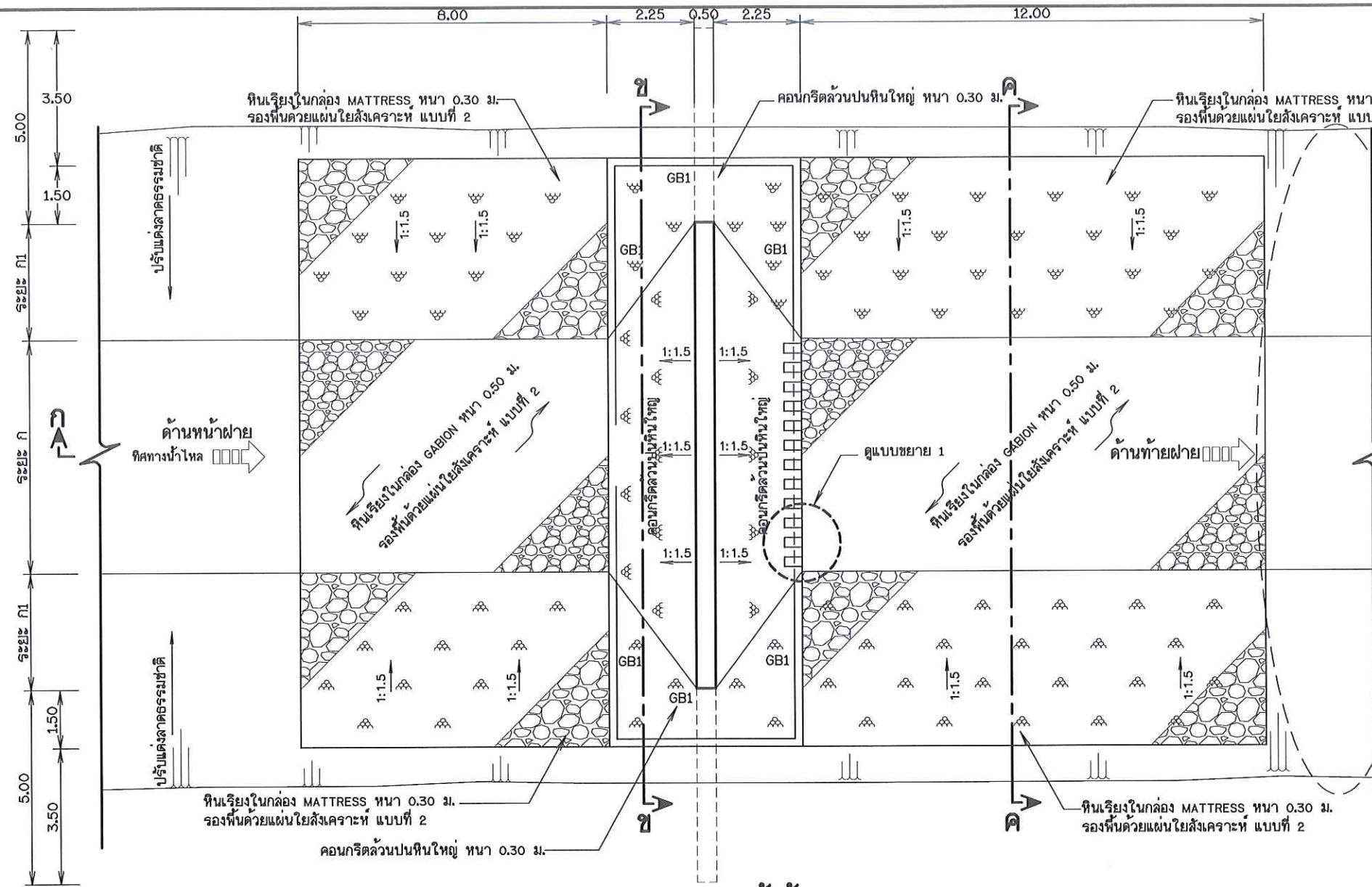
แปลนอาคารฝายน้ำล้น
