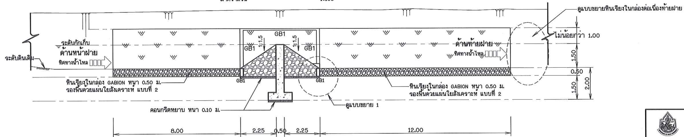
รูปตัด ก-ก
