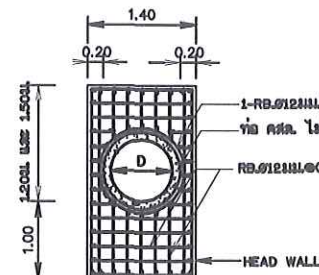
ขยายการเสริมเหล็กกำแพงปากท่อและท้ายท่อ มาตราส่วน 1:50
