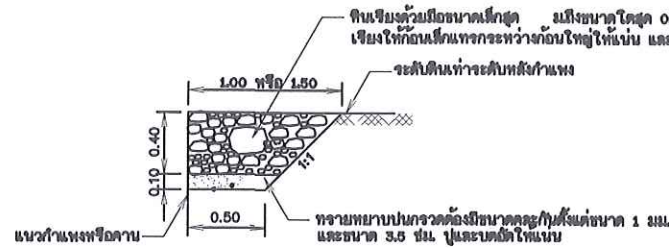
ขยายหินเรียง มาตราส่วน 1:10
