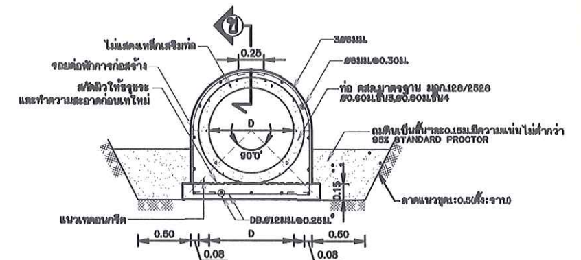
รูปตัดการวางท่อ คสล. มาตราส่วน 1:25
