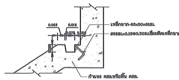
ขยายร่องใส่บานประตูไม้ มาตราส่วน 1:10
