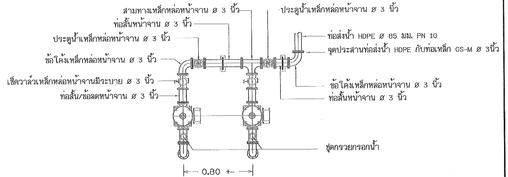
แบบขยายแสดงการติดตั้งเครื่องสูบน้ำ มาตรฐาน 1:25
