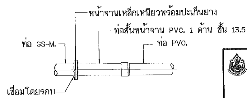
11. การบรรจุบ่อก่อเหล็กอบสังกะสี (G/S) กับท่อ PVC.
