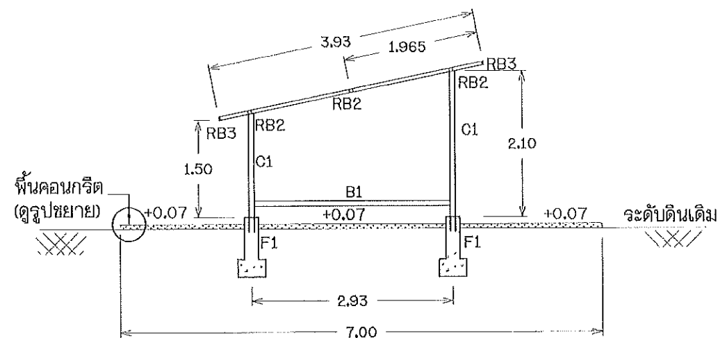
รูปตัด โครงรับแรง มาตราส่วน 1:75
