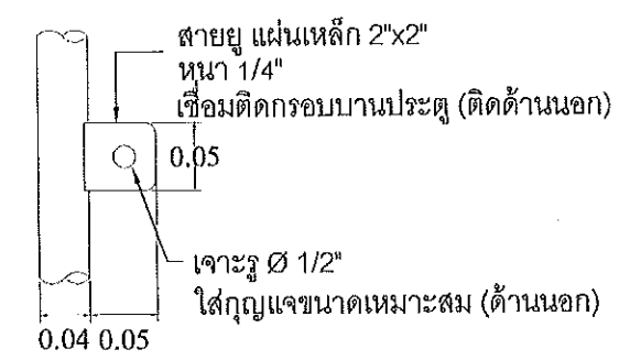
แบบขยายสายยู
