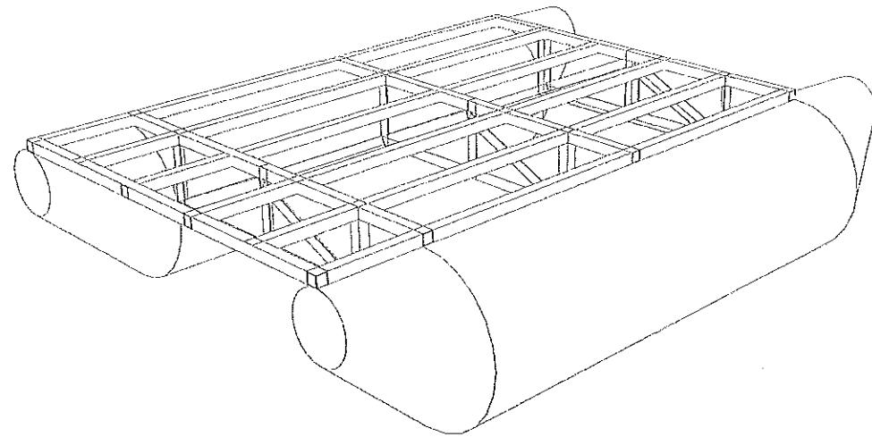
รูปแสดงการติดตั้งโครงเหล็ก มาตรฐาน not to scale
