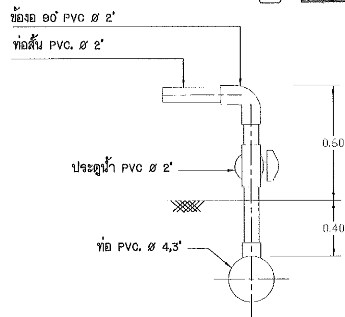
19. แบบจุดจ่ายน้ำ
