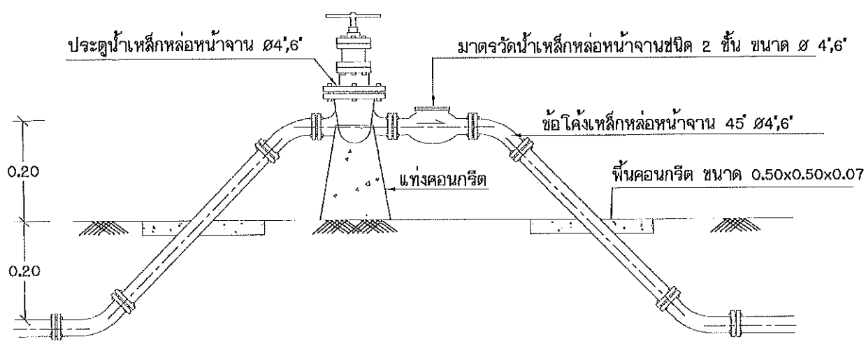
10. การติดตั้งมาตรวัดน้ำบนพื้นดิน ๑ 4", 6"
