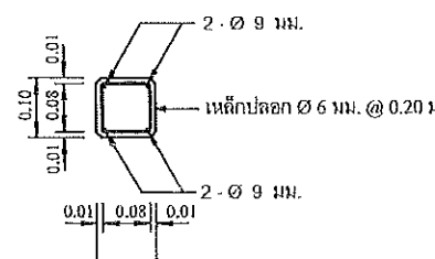
รูปตัด ข - ข
