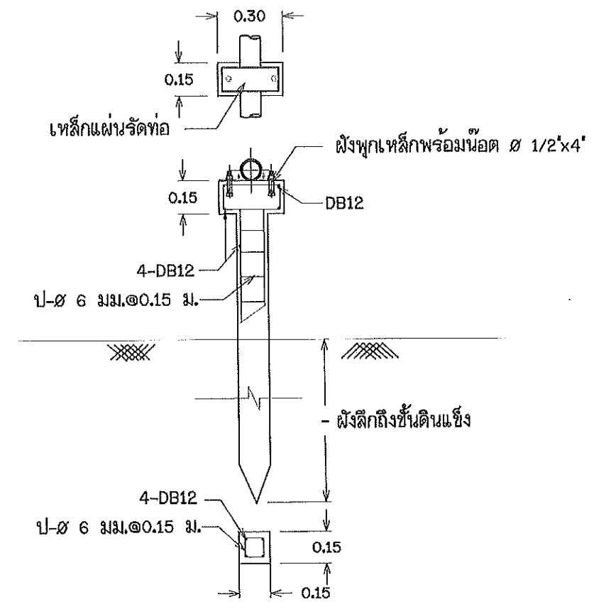
18. แบบการติดตั้งท่อดูด
