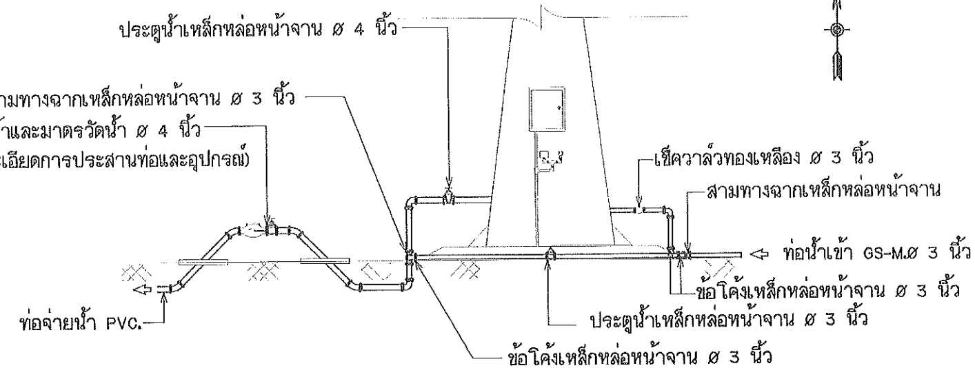
รูปขยายท่อจ่ายน้ำหอดึงสูง มาตราส่วน not to scale
