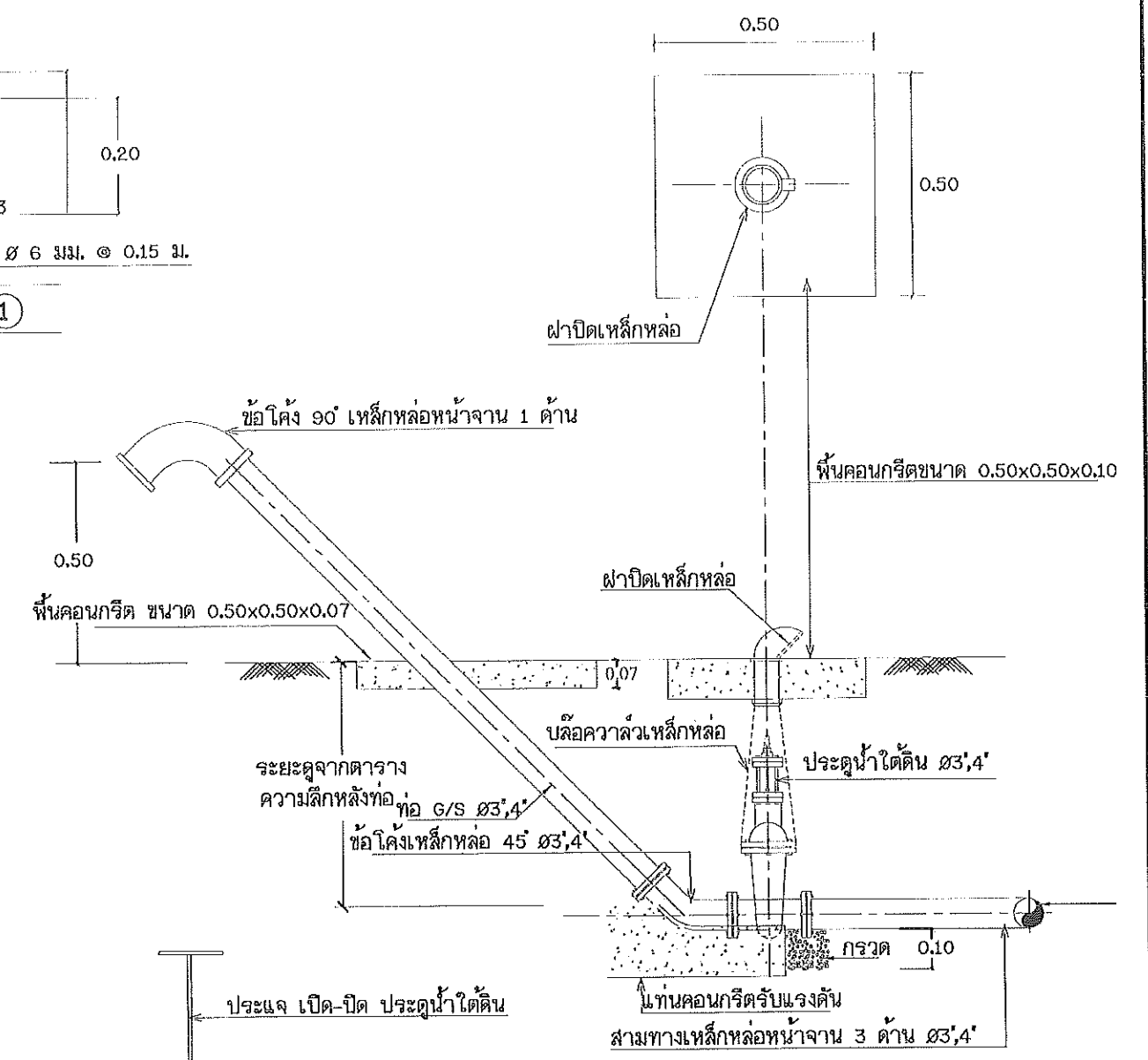
9. แบบการติดตั้งประตูปะบายตะกอน
