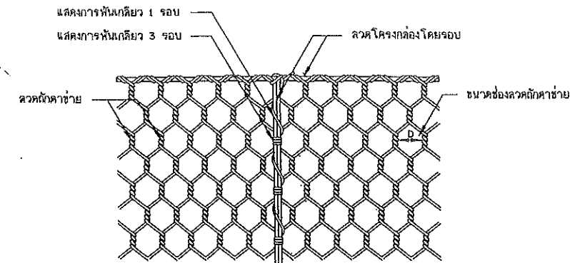
รูปแสดงการผันลวดระหว่างกล่องลวดตาข่ายและฝาปิด
