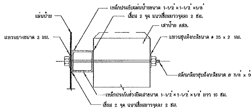
รูปตัดขยายการยึดแผ่นป้ายและเสา A000000 1:20
