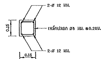
รูปตัด ก - ก A000000 1:10
