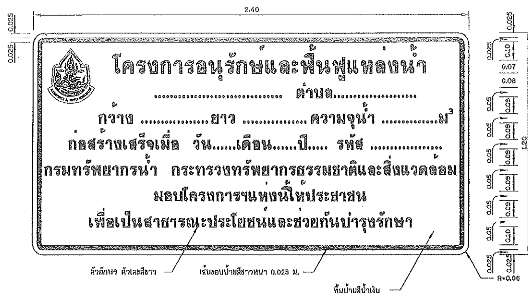
ป้ายโครงการ A000000 1:10
