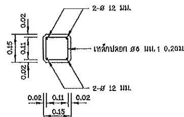
รูปตัด ข - ข A000000 1:10
