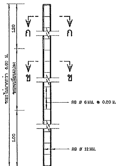
รายละเอียดเสาป้าย คสล. A000000 1:20
