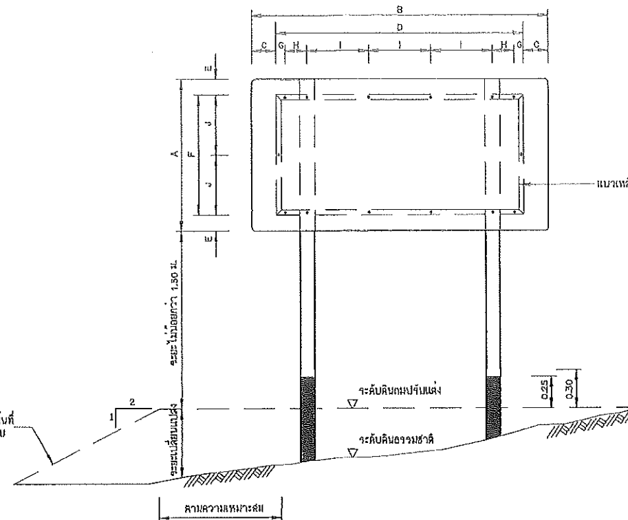
รูปแสดงการประกอบแผ่นป้าย A000000 1:20
