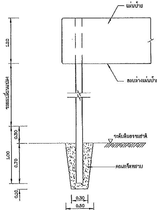
รายละเอียดการติดตั้งเสาป้าย A000000 1:20
