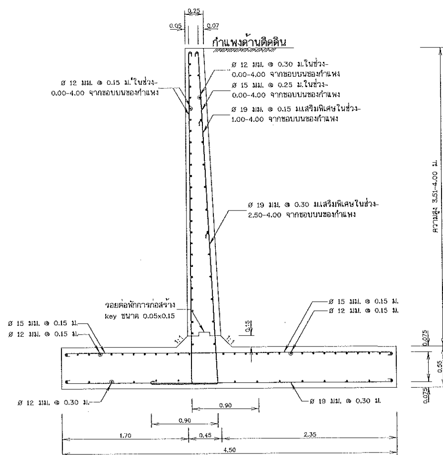
รูปขยายกำแพงกันดินความสูงระหว่าง 3.51-4.00 เมตร
