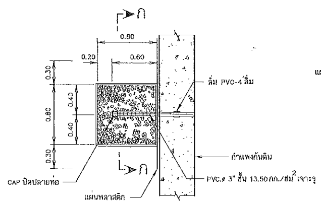
รูปขยายท่อระบายน้ำซีเมนต์กึ่งกำแพง
