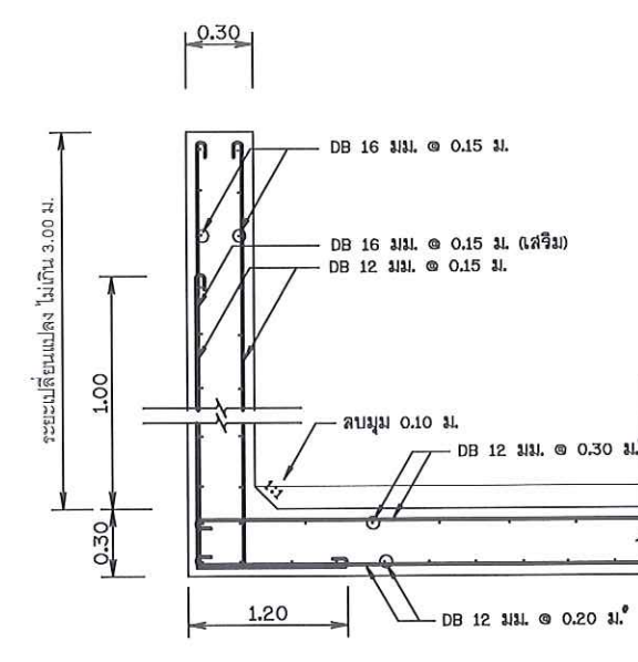
รูปตัด " ก "
