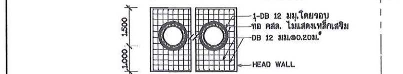
ขยายการเสริมเหล็กกำแพงปากท่อ
