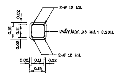
รูปตัด ข - ข
