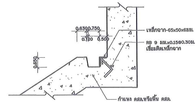
ขยายร่องไถ่บานประตู่ไม้
