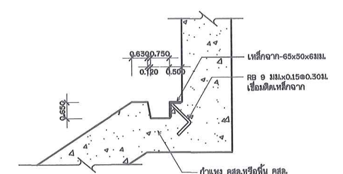
ขยายร่องไต่บานประตูไม้
