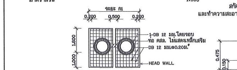
ขยายการเสริมเหล็กกำแพงท้ายท่อ
