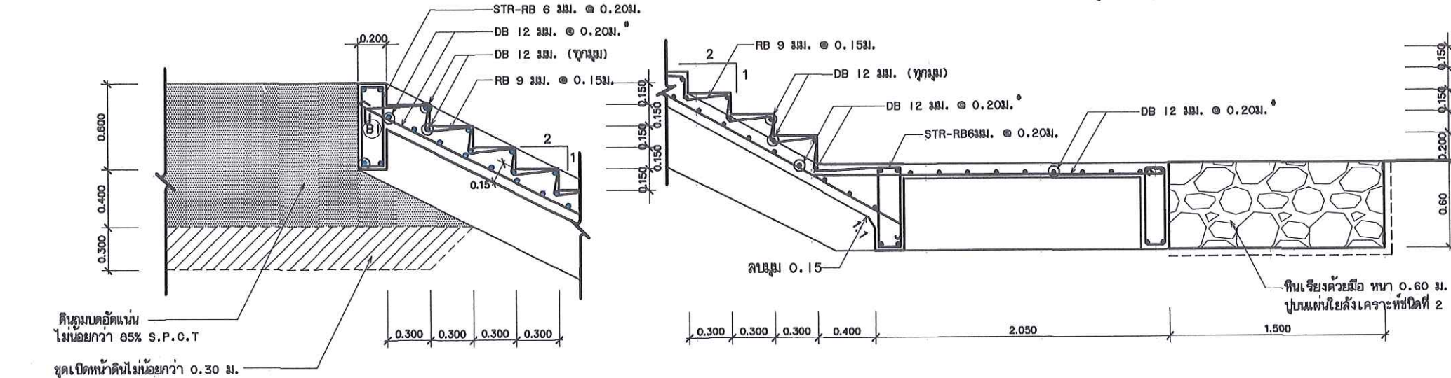
ดูแบบขยาย 1-ข
