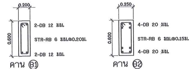
ขยายคาน B1 และ คาน B2
