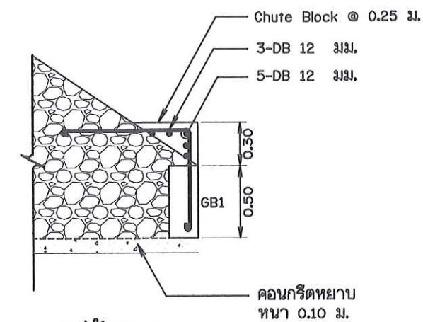
รูปตัดขยาย 1 มาตราส่วน 1:25
