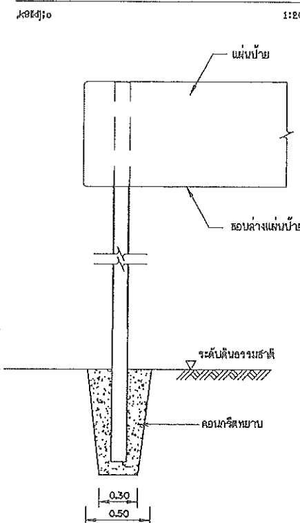
รายละเอียดการติดตั้งเสาป้าย
