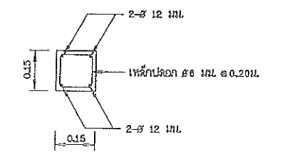
รายละเอียดเสาป้าย คสล. มาตราส่วน 1:20
