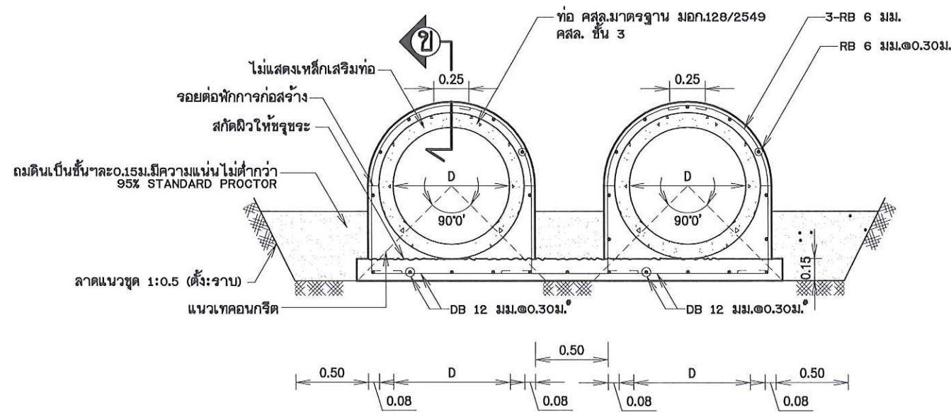
รูปตัดแนว ข - ข
