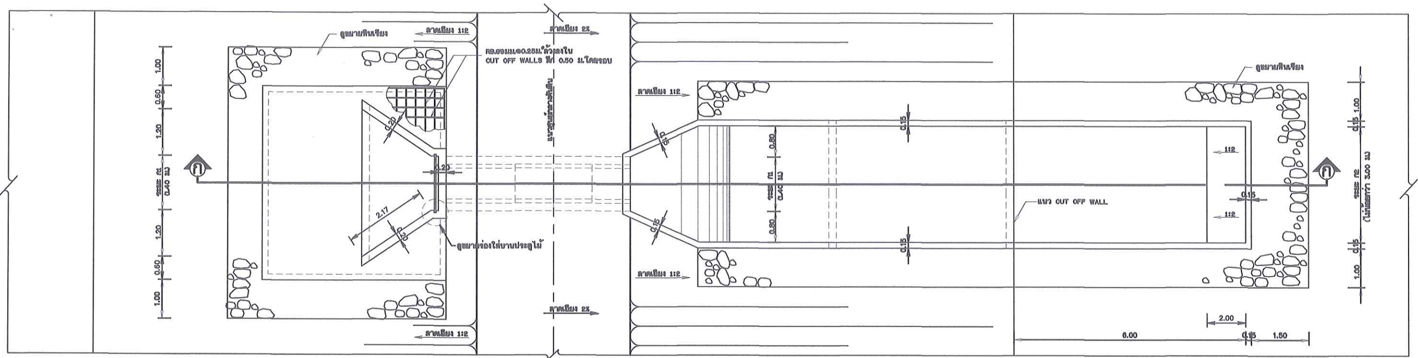
แปลนอาคารระบายน้ำ 1-Dia.0.80m มาตราส่วน 1:50
