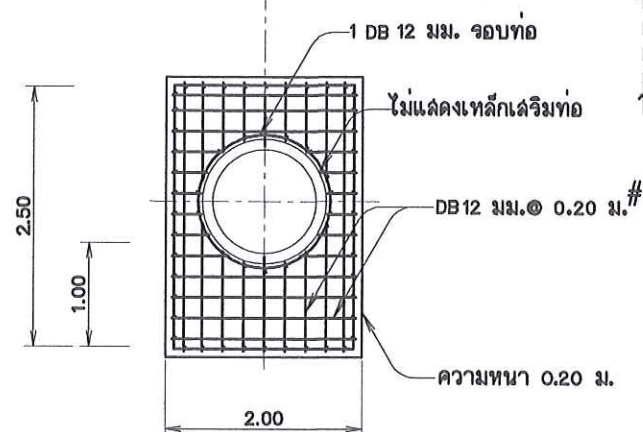
ขยายการเล่าริมหลักกำแพงปากท่อและท้ายท่อ
