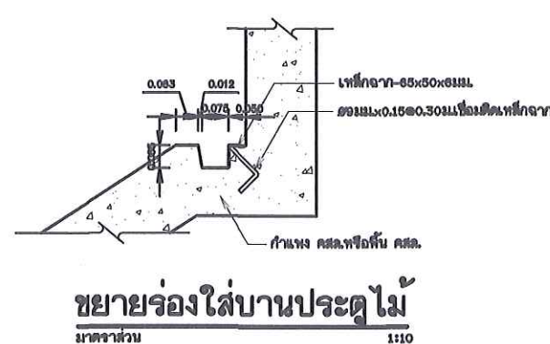
ขยายการเสริมเหล็กกำแพงปากท่อและท้ายท่อ มาตราส่วน 1:50
