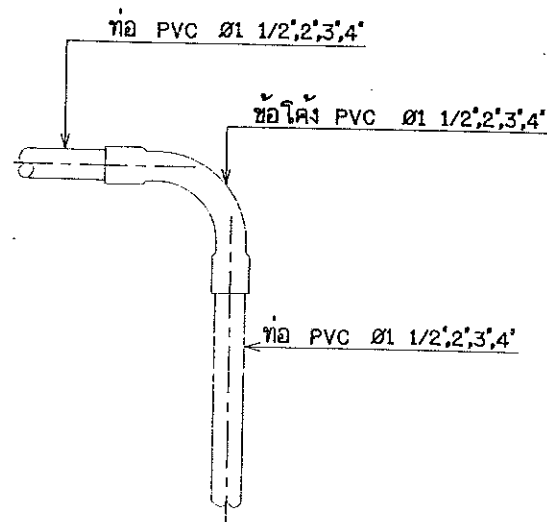
6. แบบการต่อข้อต่อ 90° PVC.
