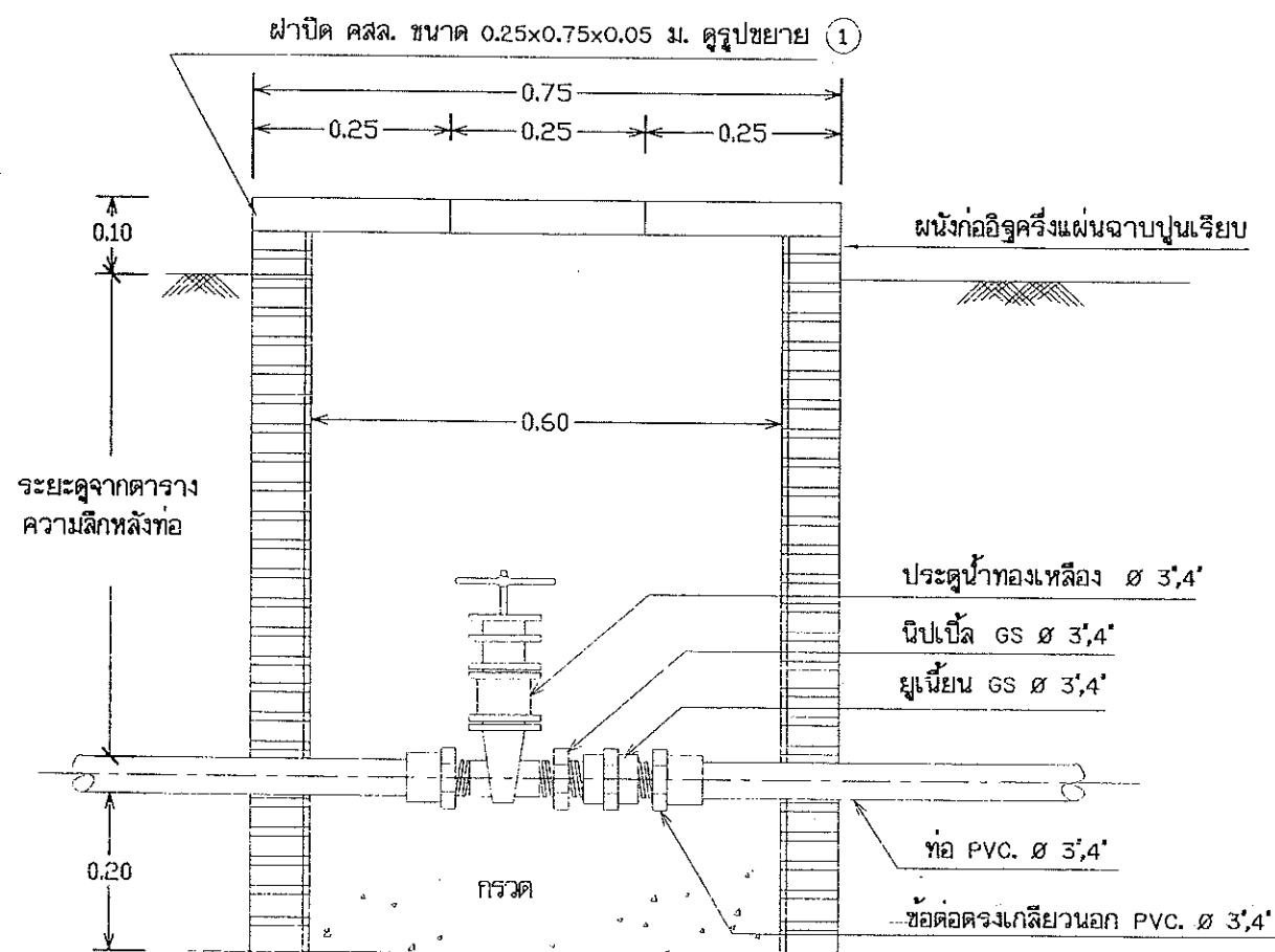
16. แบบการติดตั้งประตูป้าทองเหลือง ขนาด 0.75x0.75 ม.
