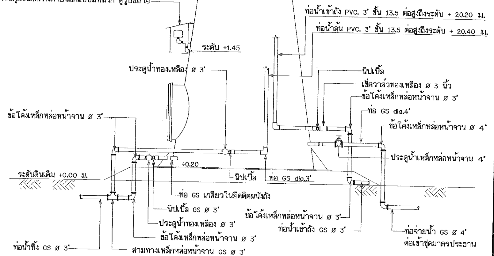
แบบแสดงการเดินท่อในหอถังสูง มาตราส่วน 1 : 25
