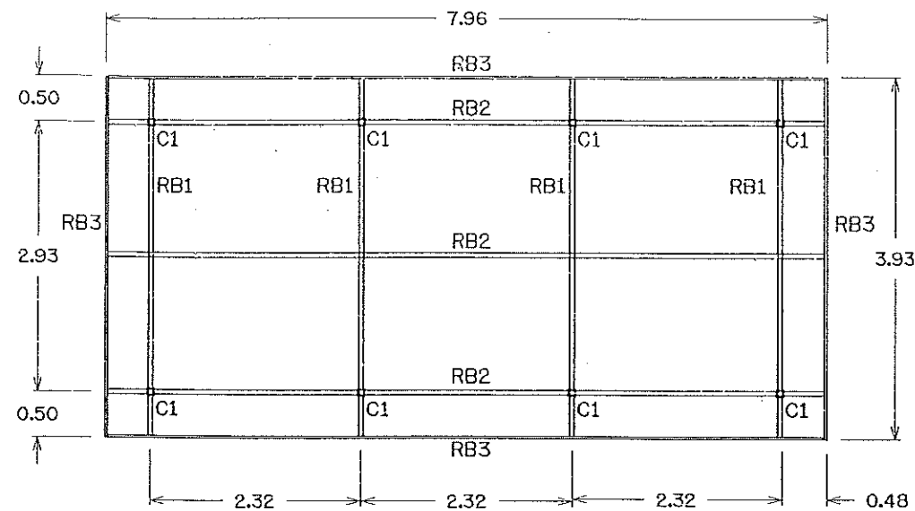
แปลนคานโครงหลังคา มาตรฐาน 1:75
