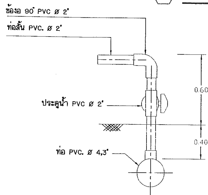
19. แบบจุดจ่ายน้ำ
