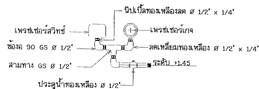
แบบขยายสิทธิ์ควบคุมและกำจัดความดัน
