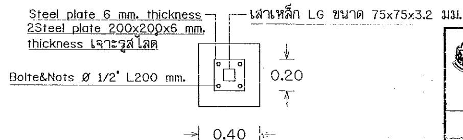
รูปขยาย C1 มาตรฐาน 1:25
