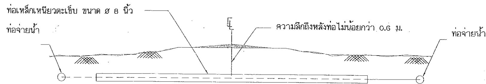
12. การเดินท่อใต้ถนน ท่อ \varnothing 2'3'4'6''
