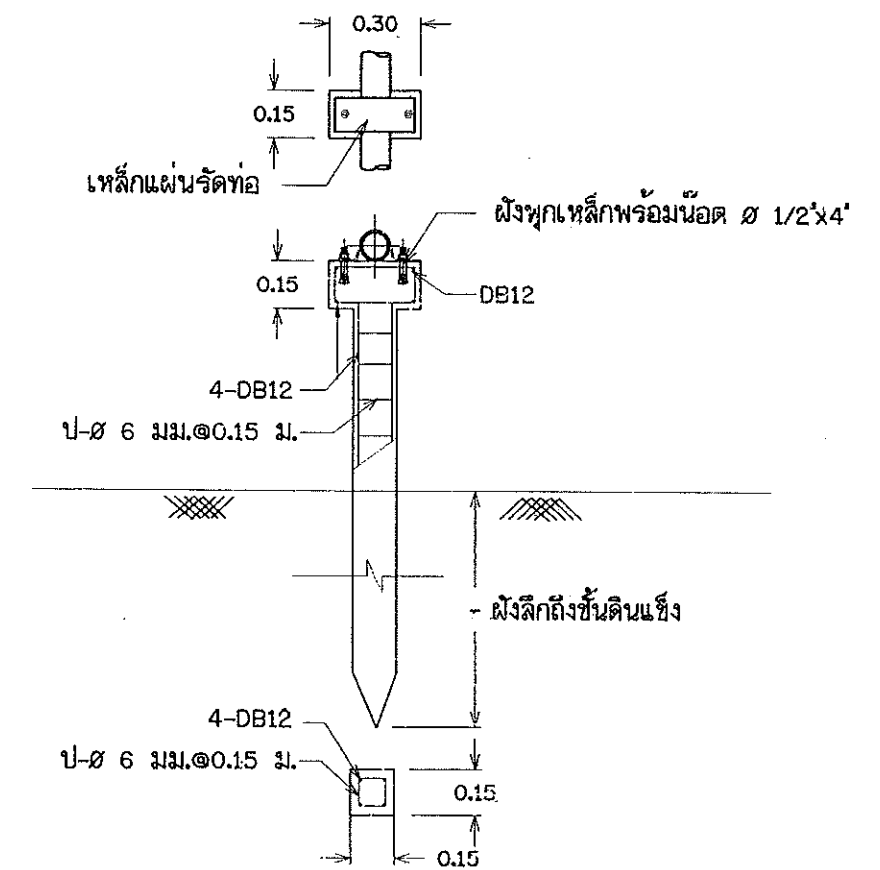
21. เสารับท่อเดี่ยว (รูปขยาย ข.)
