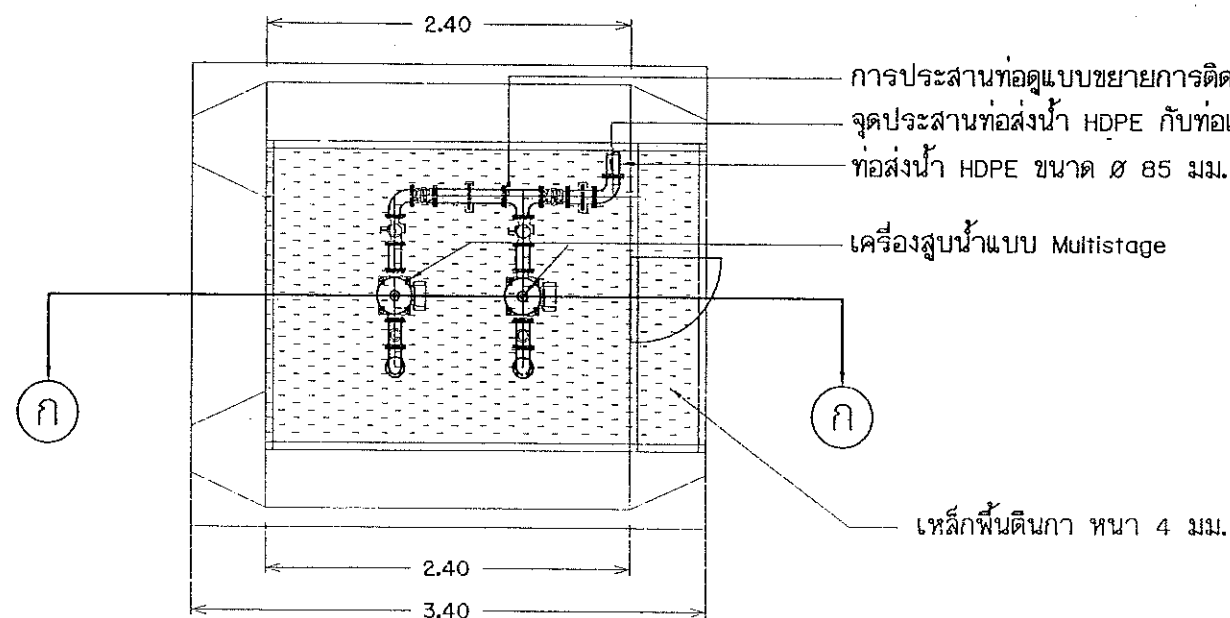
แปลนพื้นแพท่อนลอย มาตราส่วน 1:50
