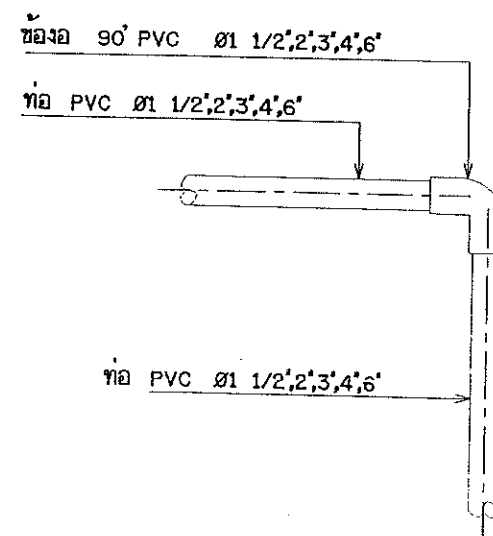
7. แบบการต่อข้อต่อ 90° PVC.
