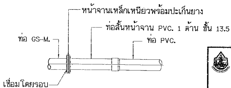
๑๑. การบรรจุบท่อเหล็กอับลังกะลี (G/S) กับท่อ PVC.
