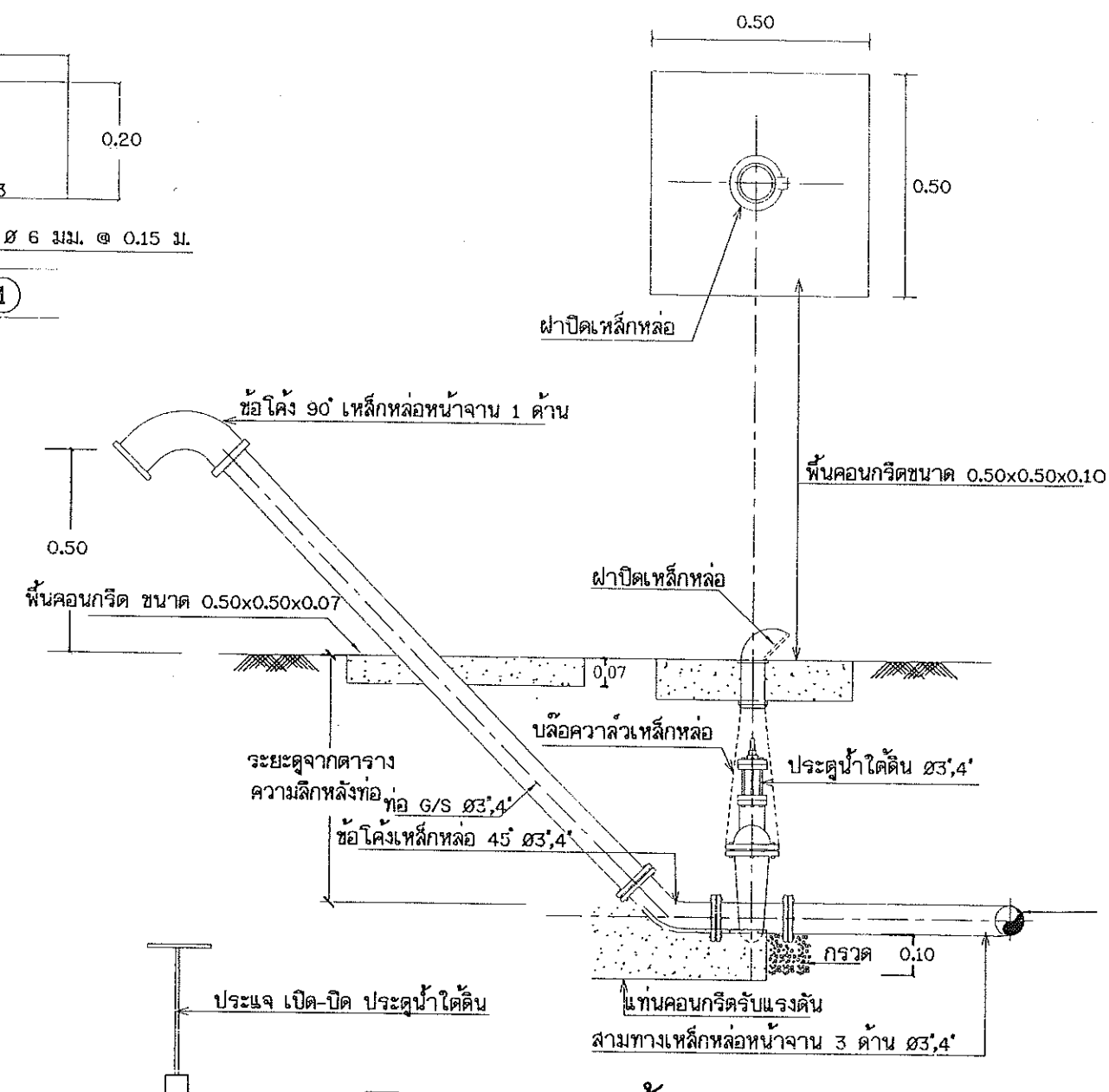
๙. แบบการติดตั้งประตูละบายตะกอน
