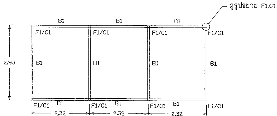
แปลนฐานรากและคานเหล็ก มาตรฐาน 1:75
