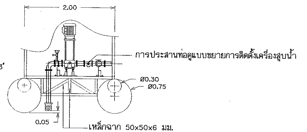
รูปขยายกันโครงและเครื่องสูบน้ำ มาตราส่วน 1:50
