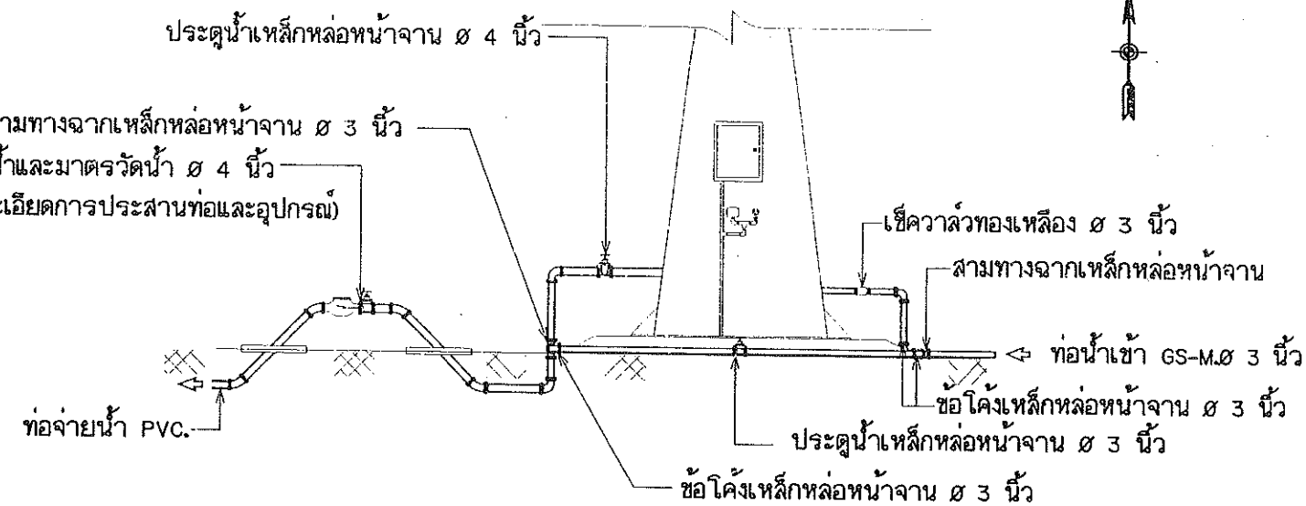
รูปขยายท่อจ่ายน้ำหม้อถังสูง มาตราส่วน not to scale
