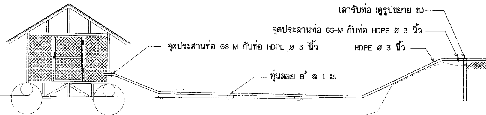
19. แบบจุดจ่ายน้ำ
