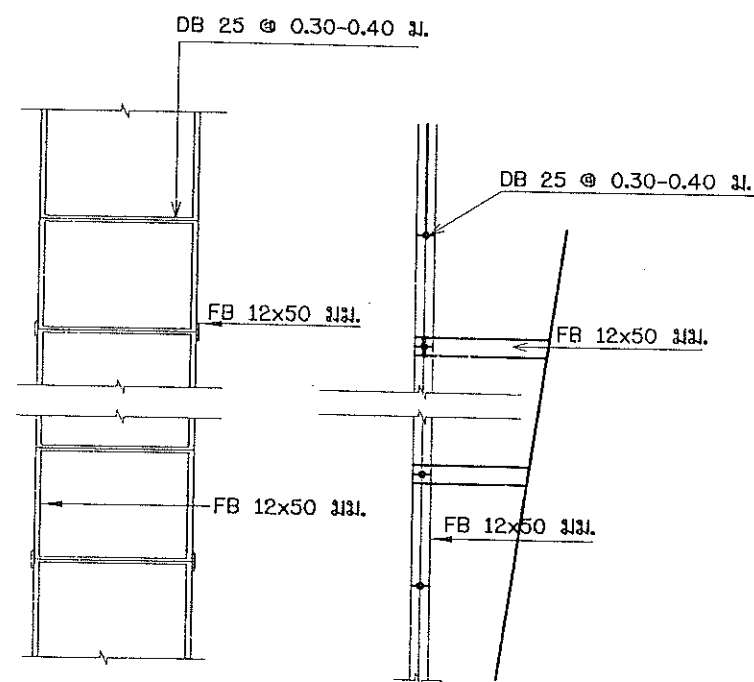
แบบขยายบันได ภายในห้องสูง มาตรฐาน 1 : 20
