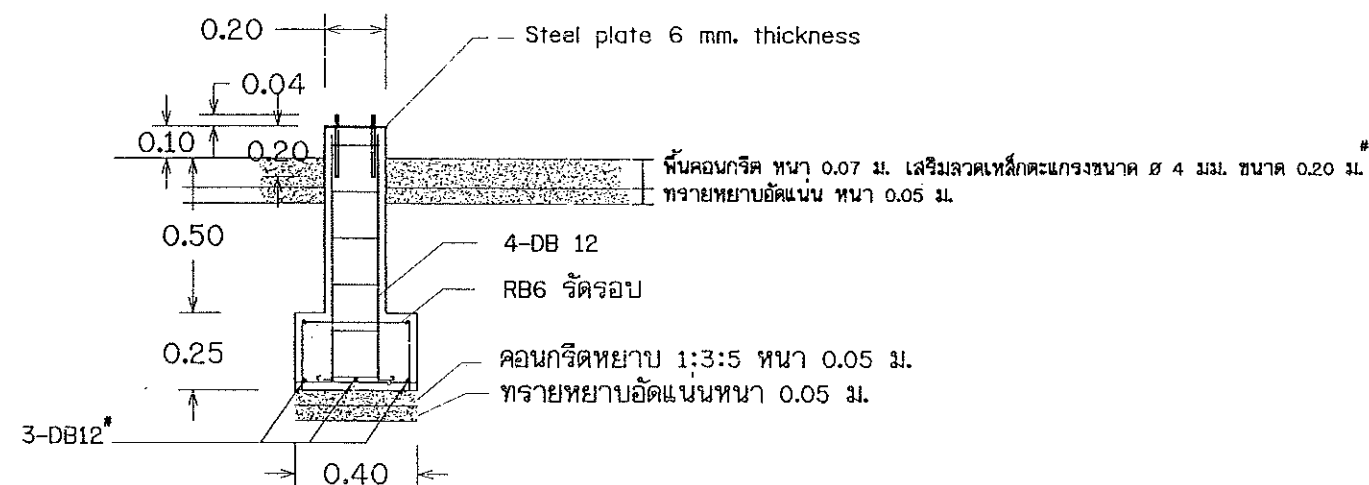
รูปขยาย F1 มาตรฐาน 1:25
