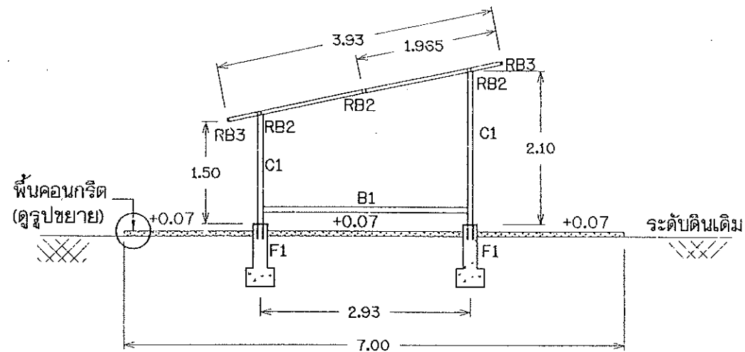
รูปตัดโครงรับแฉ่ง มาตรฐาน 1:75
