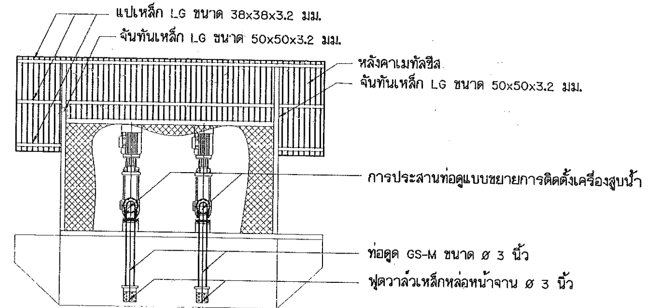
รูปตัด ก ก ท่อนลอย มาตราส่วน 1:50
