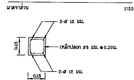
รายละเอียดเส้า پای คสล.
