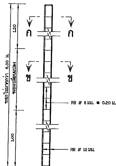
รายละเอียดเส้า پای คสล.
