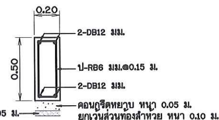
ขยายคานคอดิน GB1
