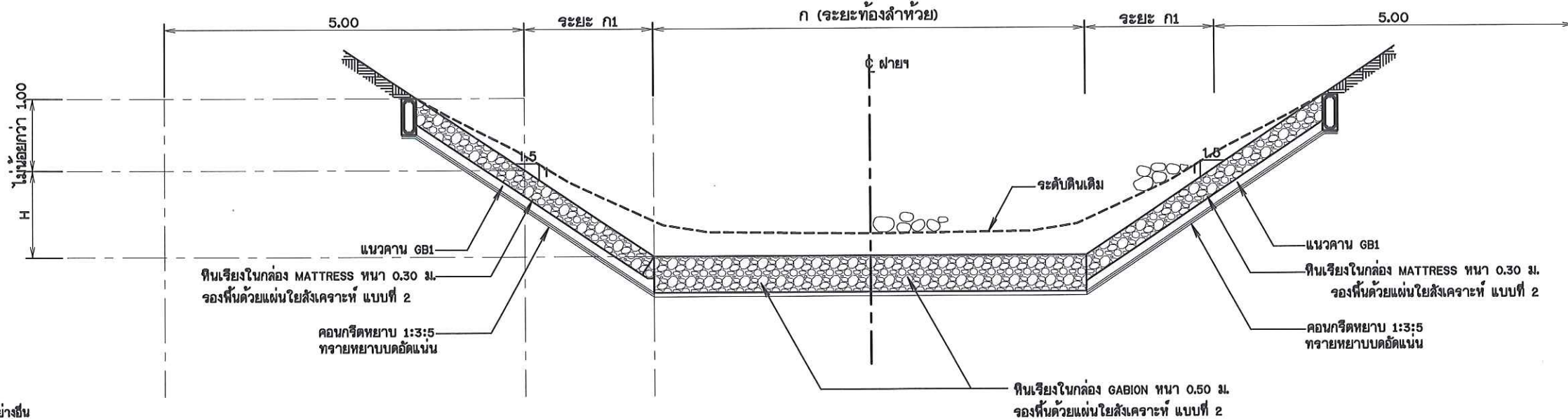
รูปตัด ค-ค
