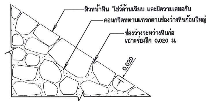
ขยายคอนกรีตล้นบนหินใหญ่
