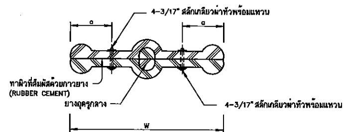
รูปตัด ก-ค ไม่แสดงขนาดส่วน
