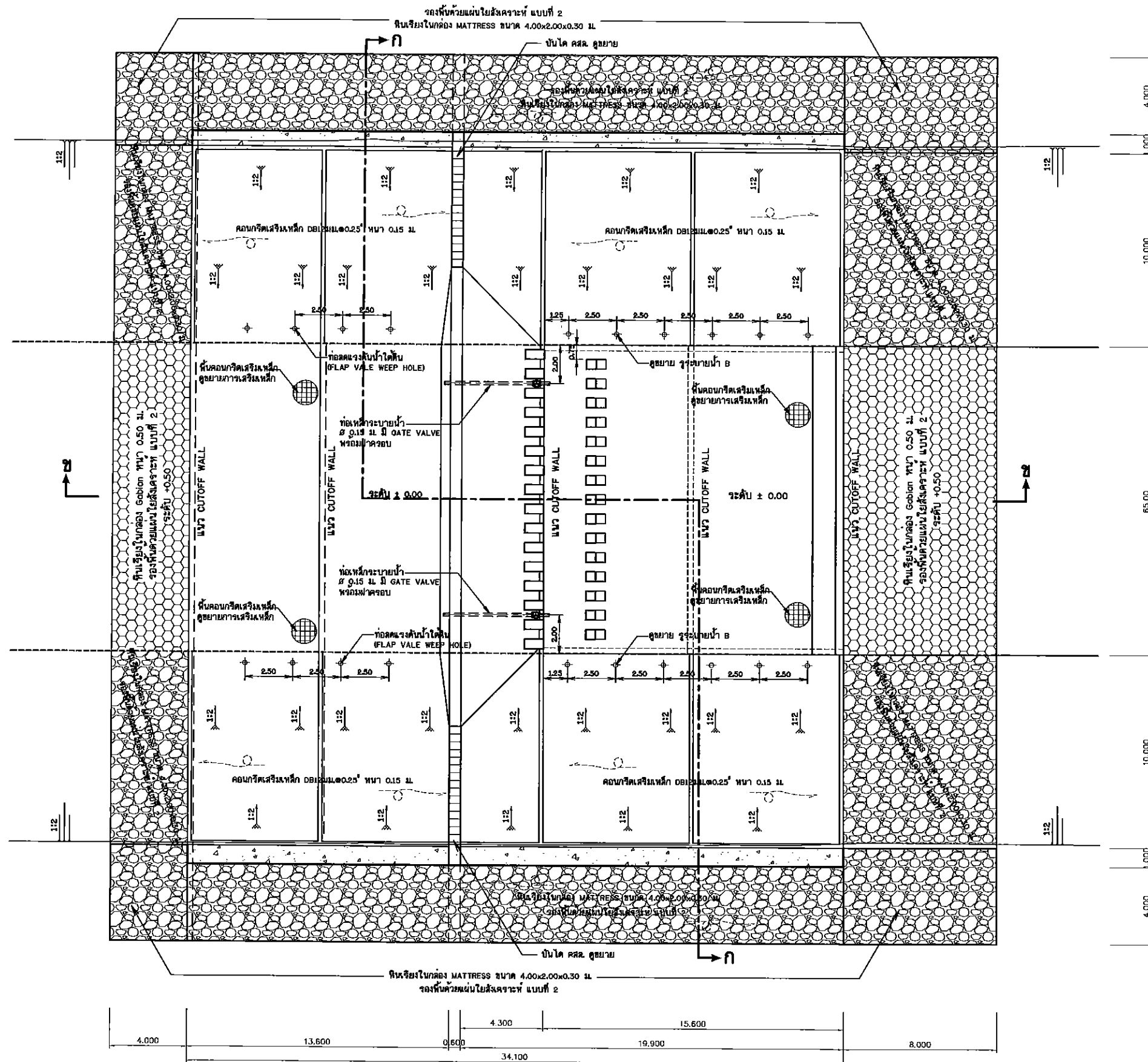
แปลนฝายชลอน้ำ คลส. มาตราส่วน 1:150
