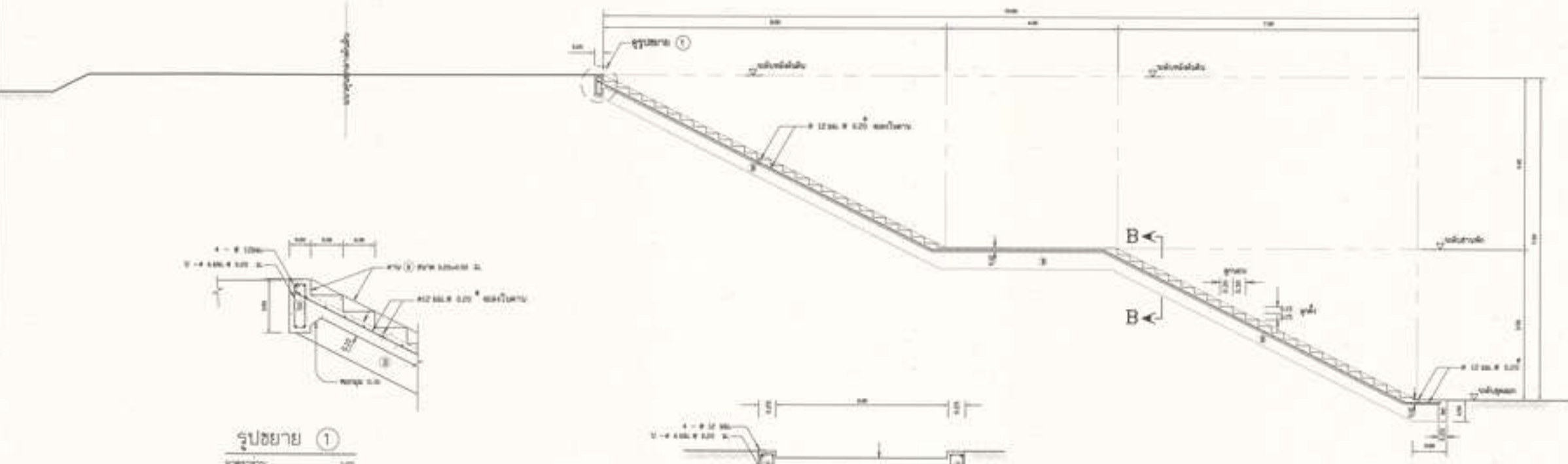
รูปตัด A - A มาตราส่วน 1:50
