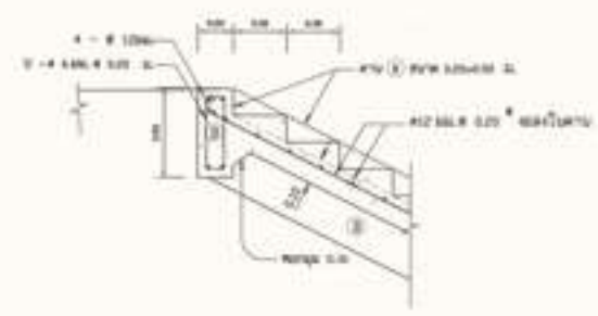
รูปขยาย ① มาตราส่วน 1:25
