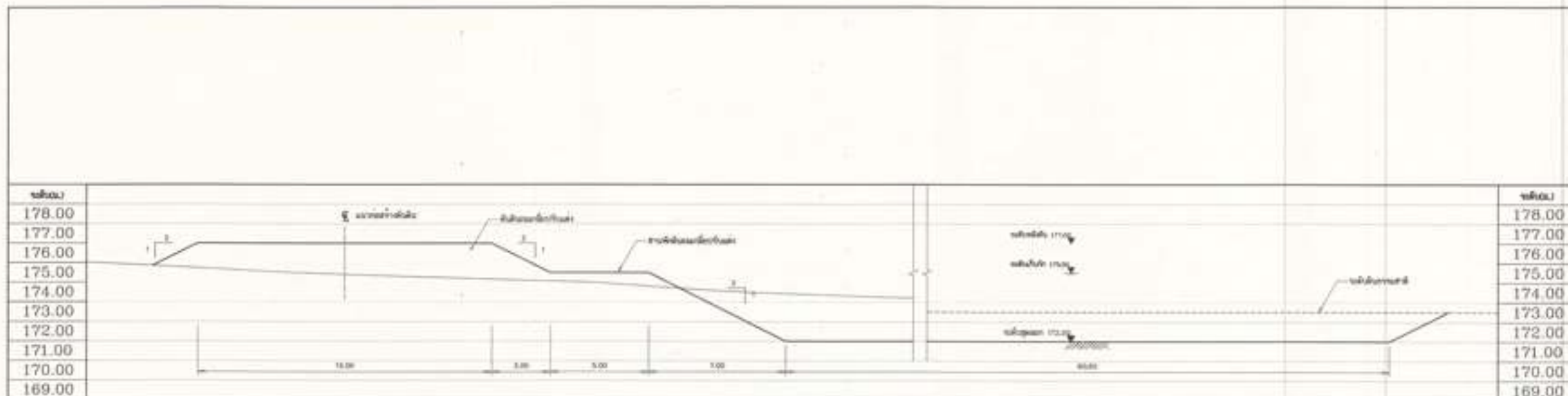
รูปตัด ก - ก ขนาดจริง 1:100
