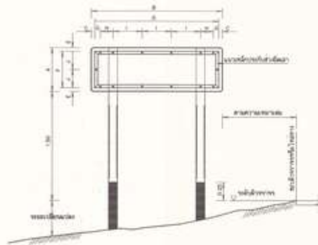
รูปแสดงการประกอบแผ่นป้าย ขนาด 1.80 x 0.60
