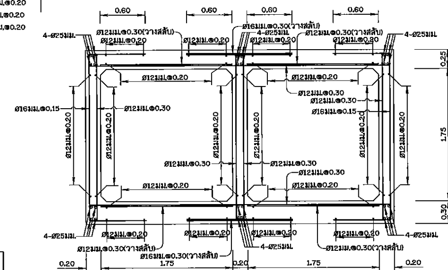
รูปตัด ง-ง มาตราส่วน 1:25
