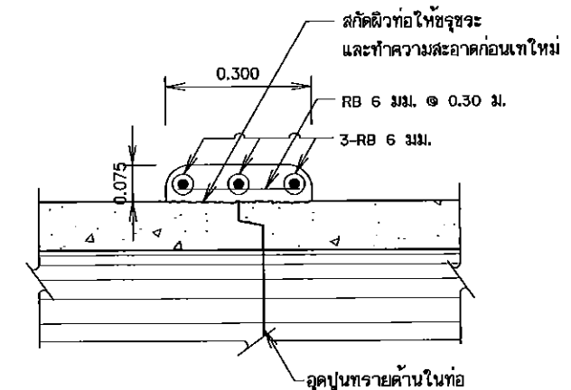
รูปตัด ข - ข
