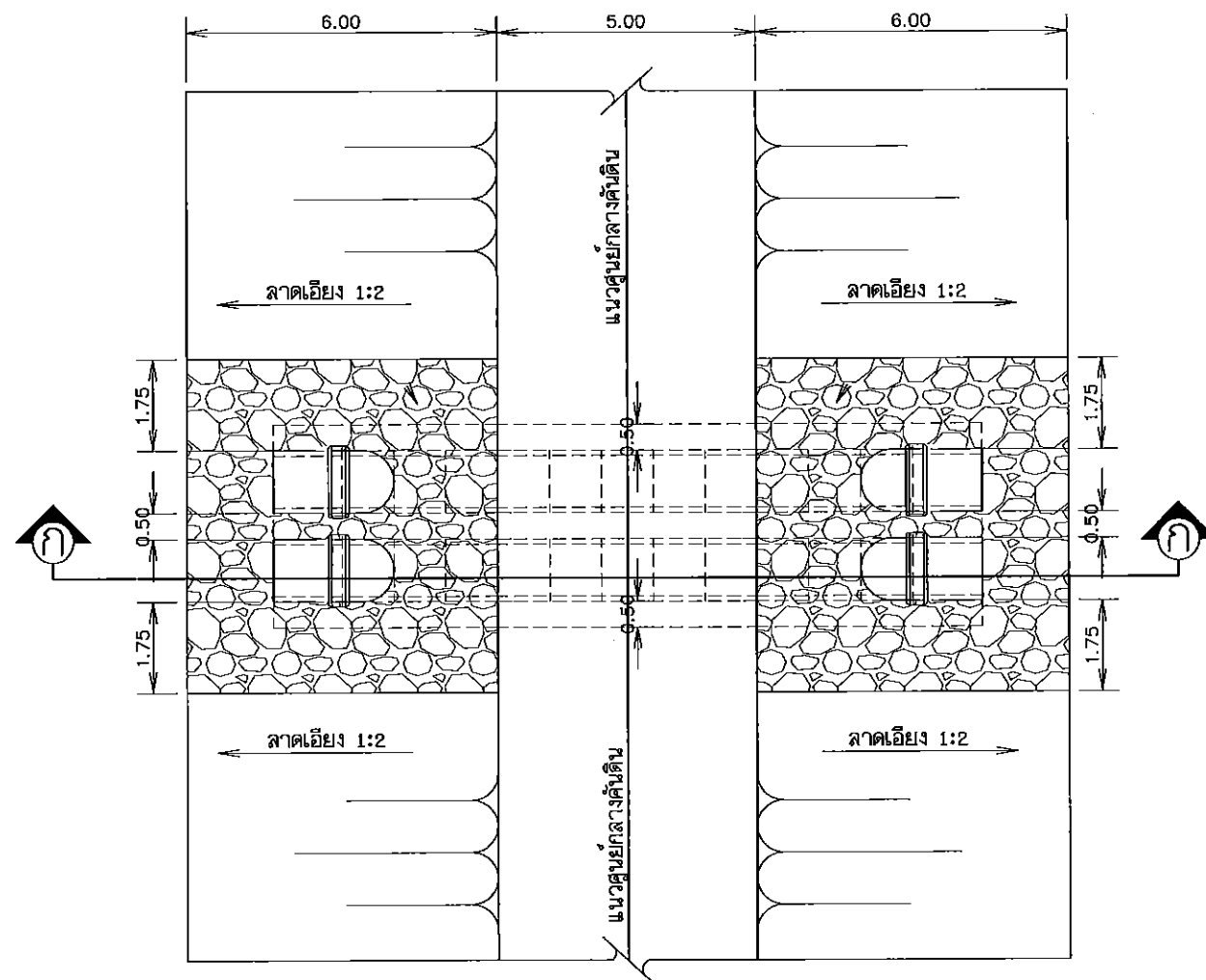
แปลนอาคารทางน้ำเข้า มาตราส่วน 1:100
