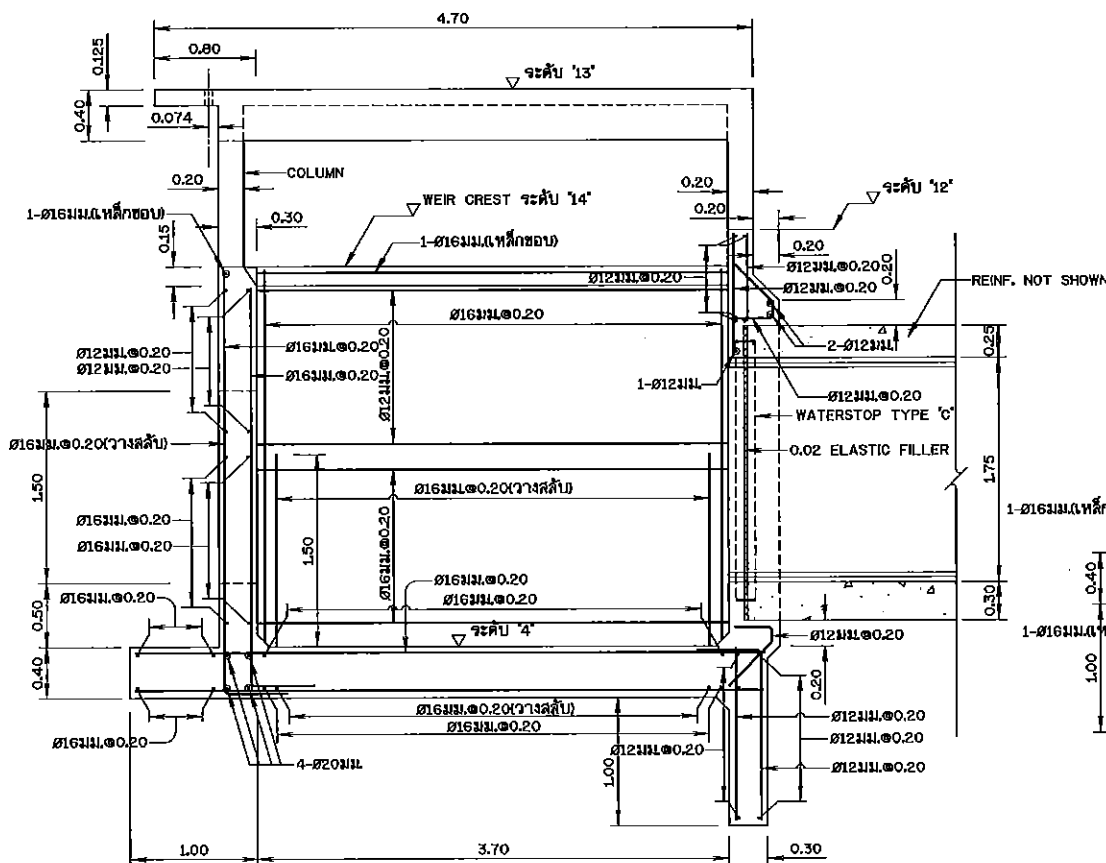
รูปตัด ก-ก (REIN. OF FAR FACE) มาตราส่วน 1:30
