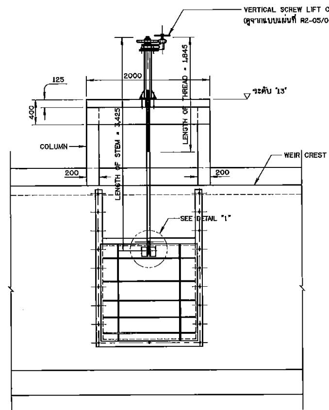
ASSEMBLY มาตราส่วน 1:30
