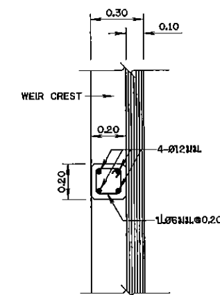
รูปตัด ข1-ข1 (COLUMN) มาตราส่วน 1:15
