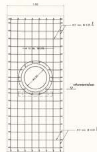
แบบขยายคอนกรีตปากท่อด้านในและด้านนอก ท่อ 1 แถว ขนาดทอ 1 : 100
