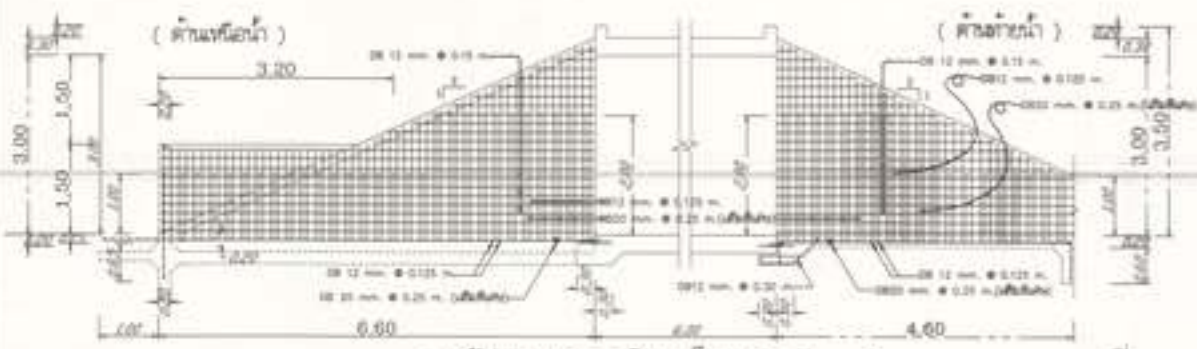
รูปตัดขยายการเสริมเหล็กแนว D - D มาตราส่วน 1:50
