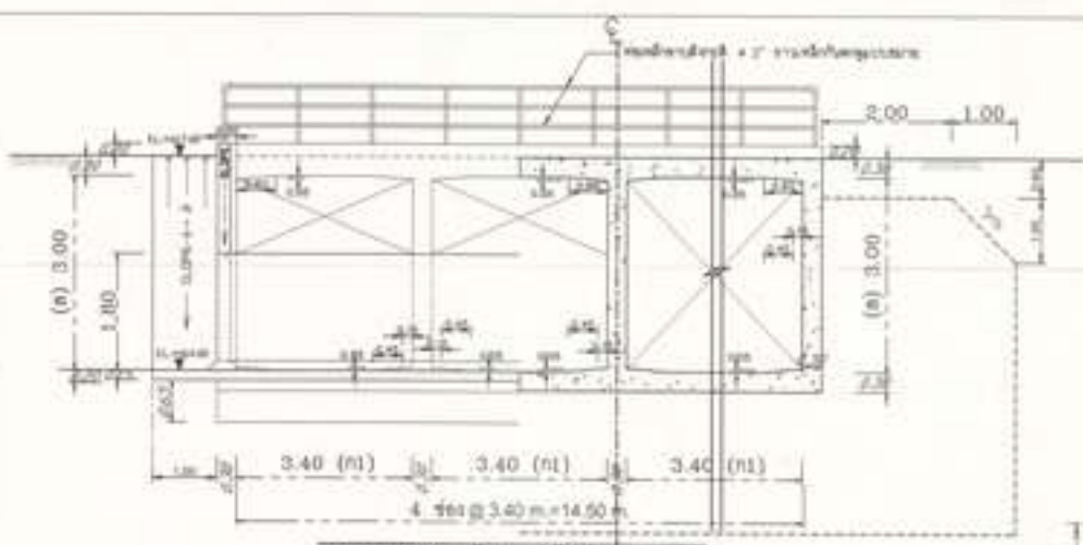
SECTION C - C 1 : 50
