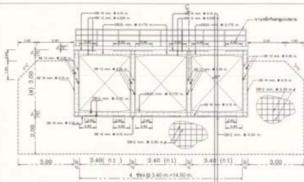
รูปตัดขยายการเสริมเหล็กแนว B - B มาตราส่วน 1:50
